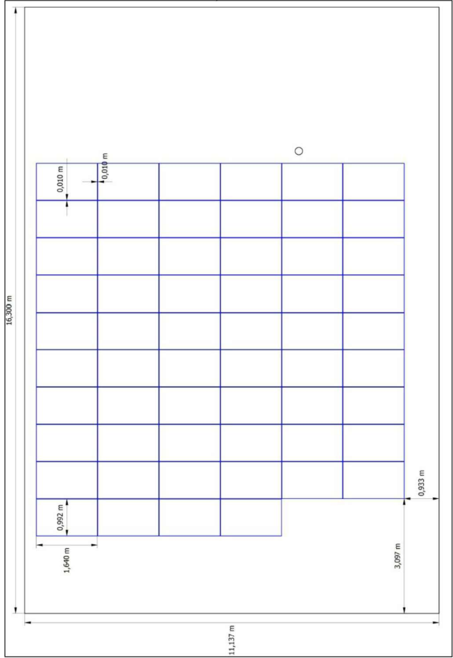
střeška č.1: Fotovoltaická elektrárna část 1 58 ks panelů 290Wp
