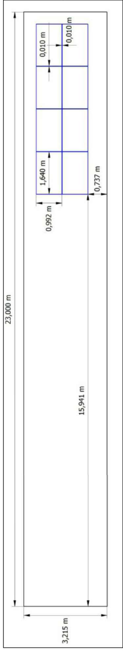
střeška č.2: Fotovoltaická elektrárna část 2 8 ks panelů 290Wp
