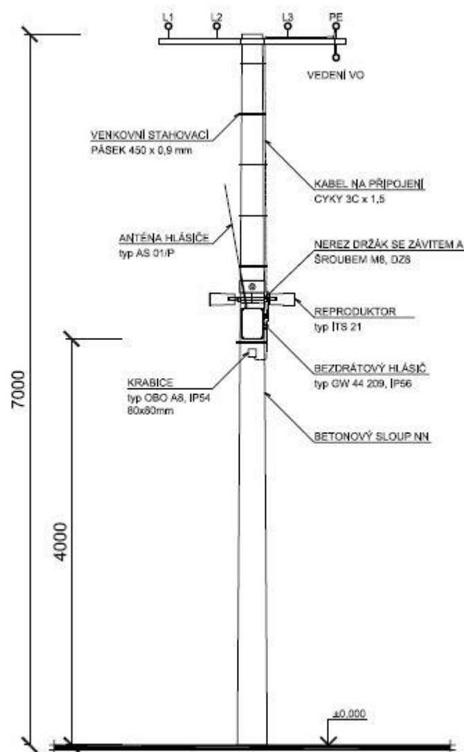
Obrázek 5:: Schéma instalace bezdrátových hlásičů
