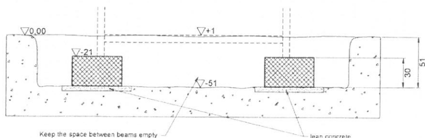
Sez. A-A
