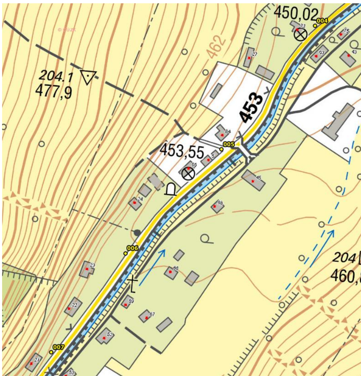
Umístění hlásičů v obci Holčovice – detail 2
