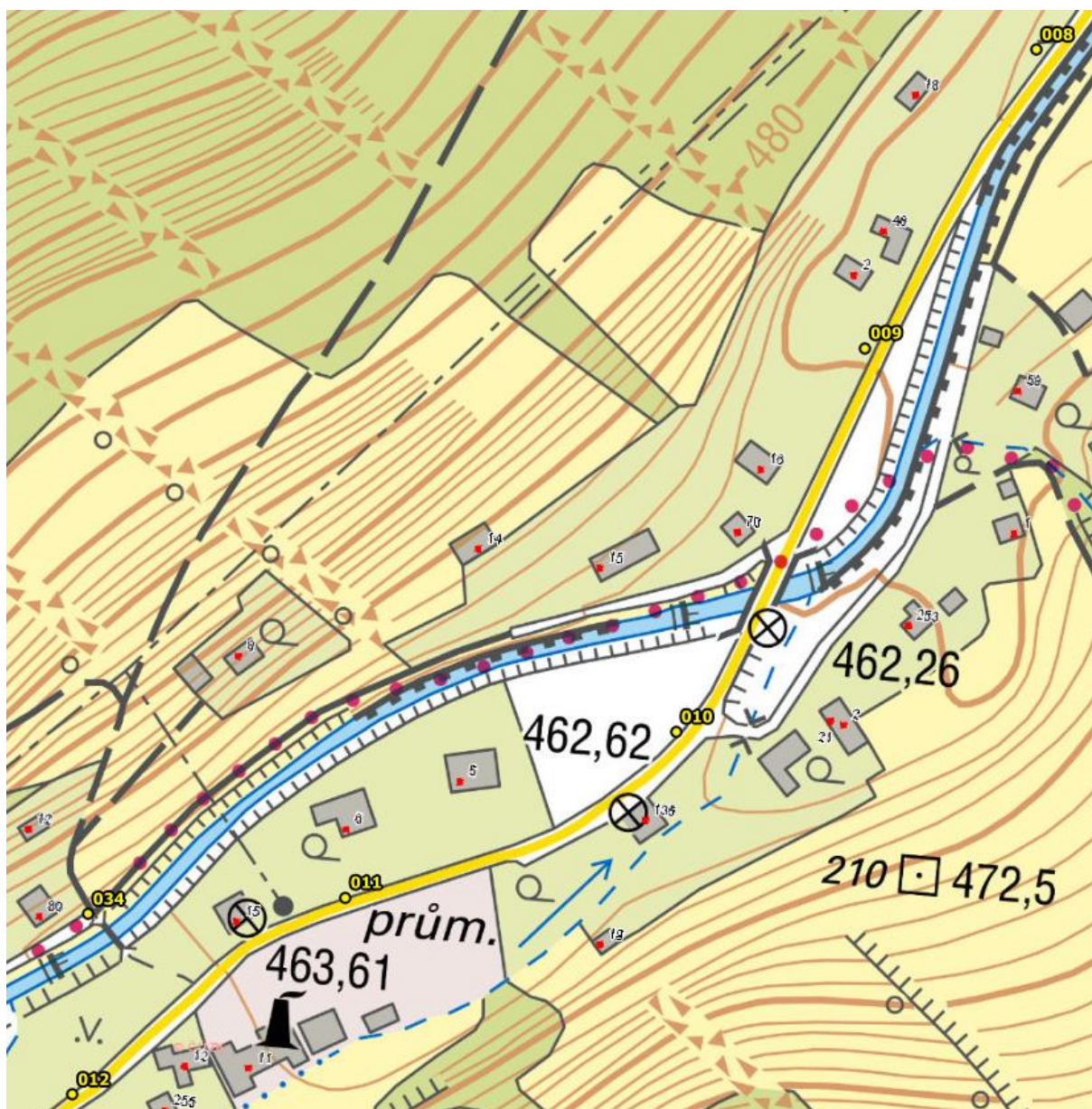
Umístění hlásičů v obci Holčovice – detail 3
