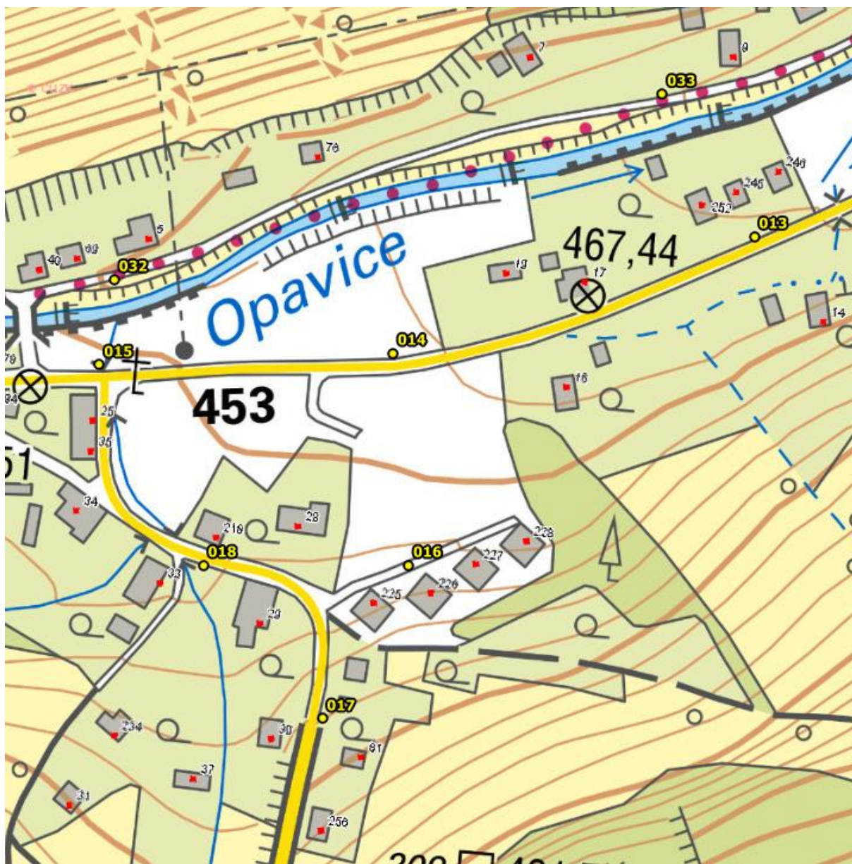
Umístění hlásičů v obci Holčovice – detail 4
