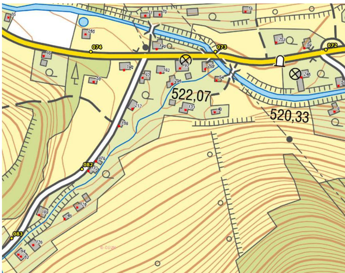
Umístění hlásičů v obci Holčovice – detail 15
