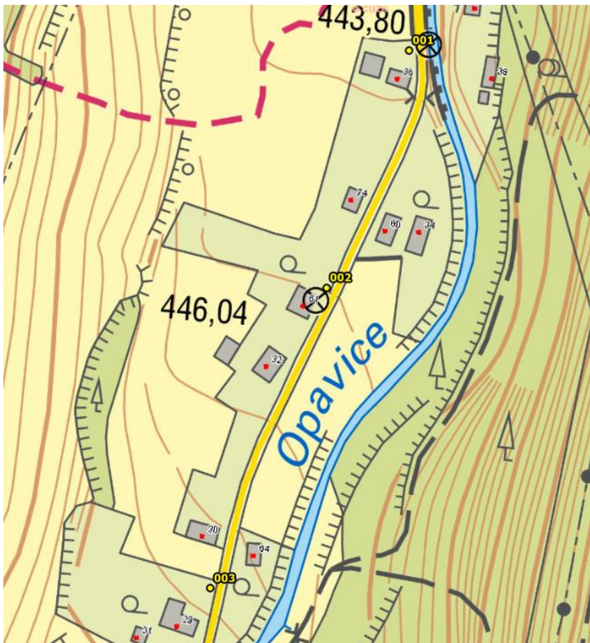
Umístění hlásičů v obci Holčovice – detail 1
