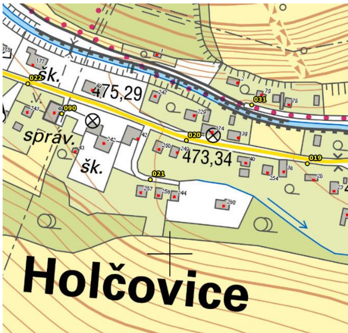
Umístění hlásičů v obci Holčovice – detail 5
