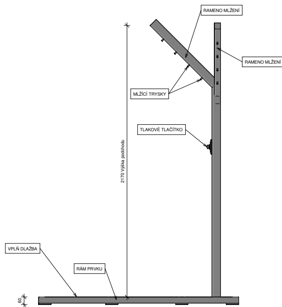
2 POHLED BOČNÍ 1 : 10
