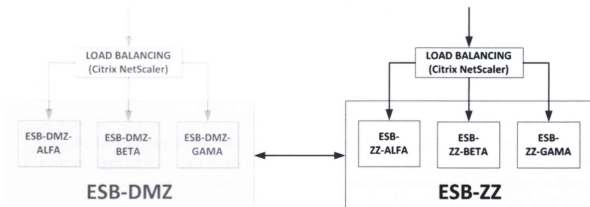
Obrázek: Rozložení zátěže a zajištění zastupitelnosti v ZZ
