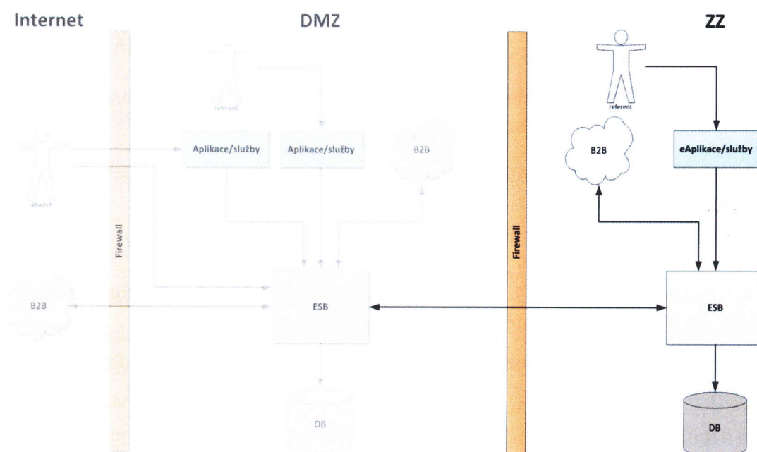
Obrázek: Modernizace architektury ZZ a její napojení na DMZ
