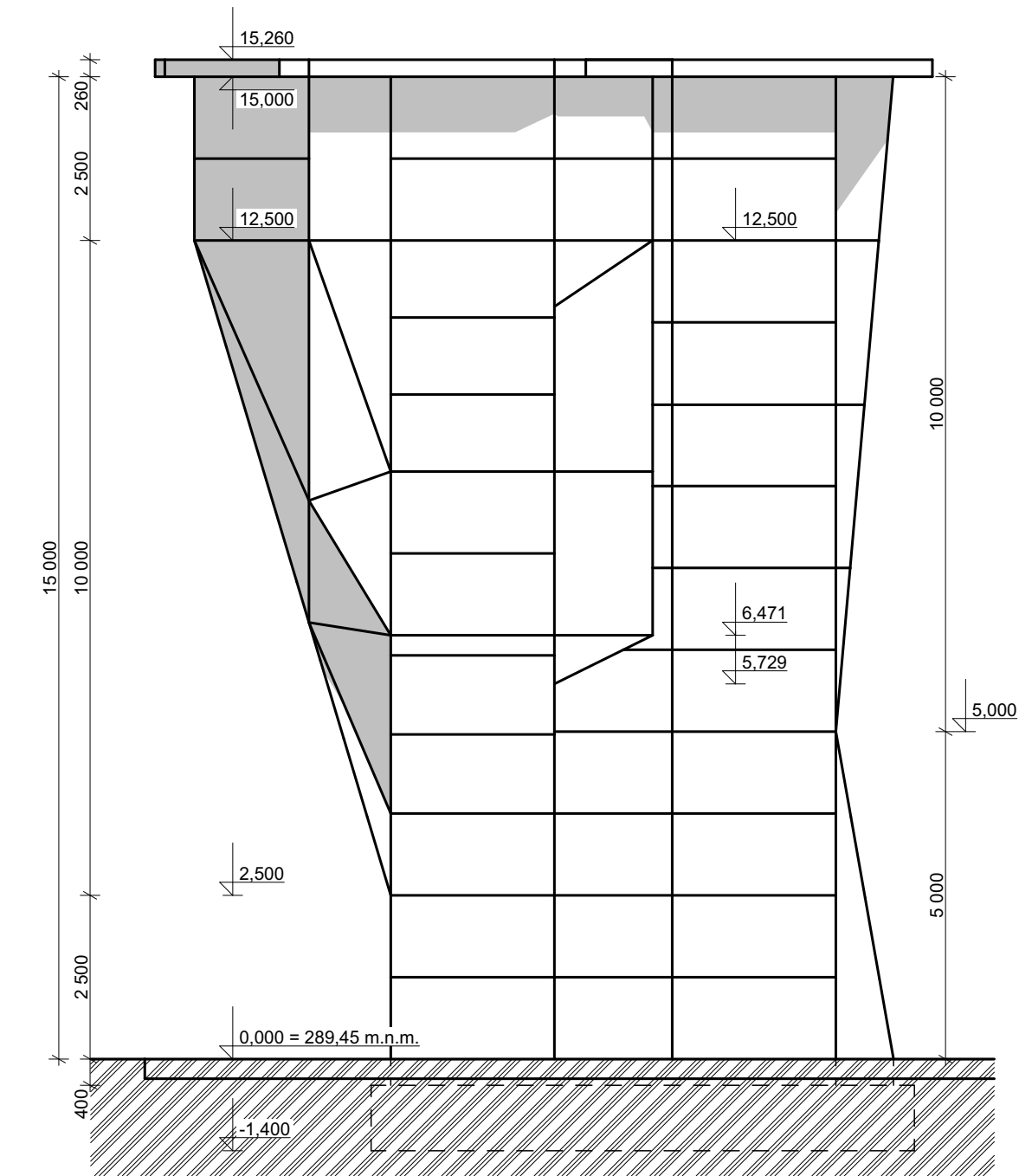
POHLED SEVEROZÁPADNÍ
