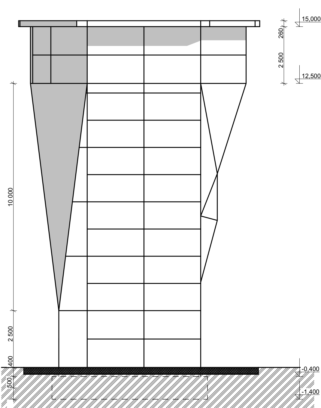
POHLED SEVEROVÝCHODNÍ
