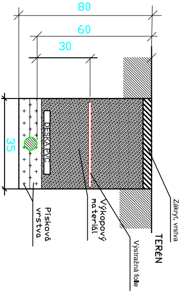
ŘEZ KABELOVYD U TRASDU V TERÉNU
