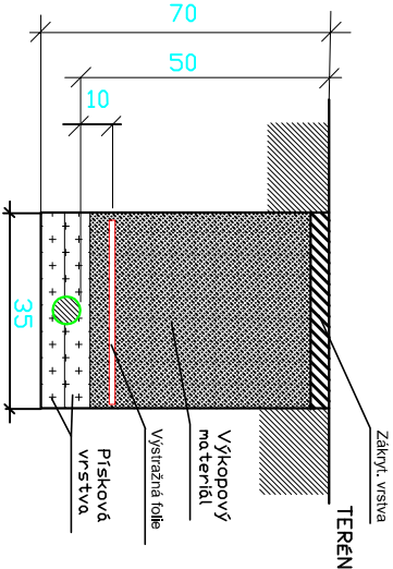
ŘEZ KABELOVYD U TRASDU V CHODNIKU
