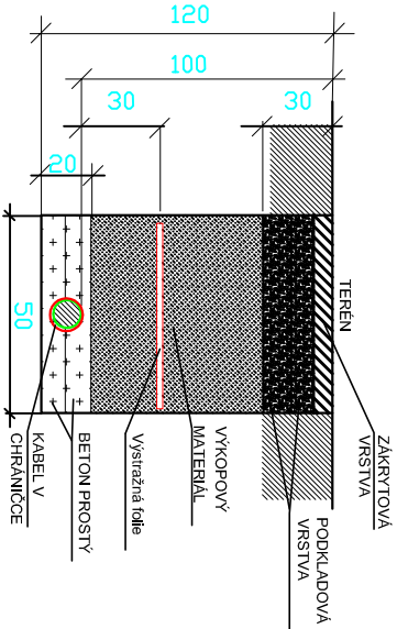
ŘEZ KABELOVYD U TRASDU VE VOZOVCE
