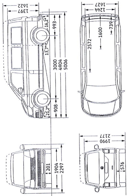
Transporter kombi s krátkým rozvorem se základní střechou a středně vysokou střechou
