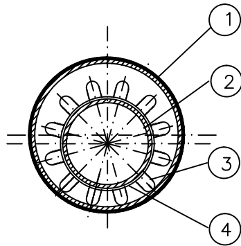
VZOROVÝ PŘÍČNÝ ŘEZ CHRÁNIČKOU
