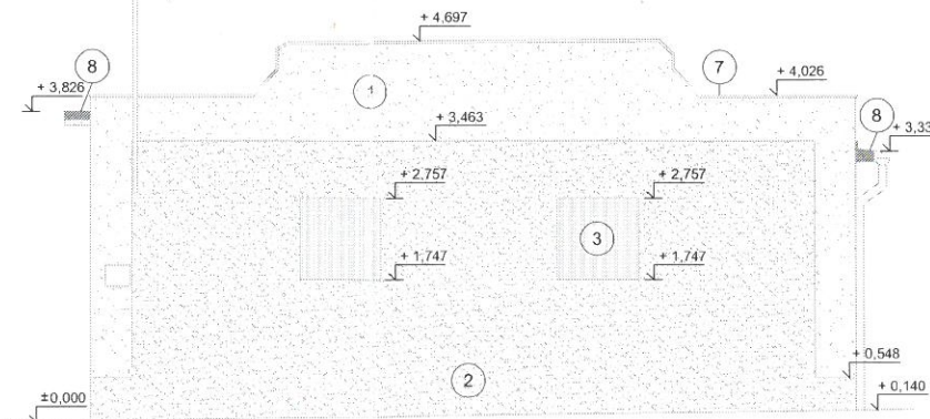
JÍŽNÍ POHLED
