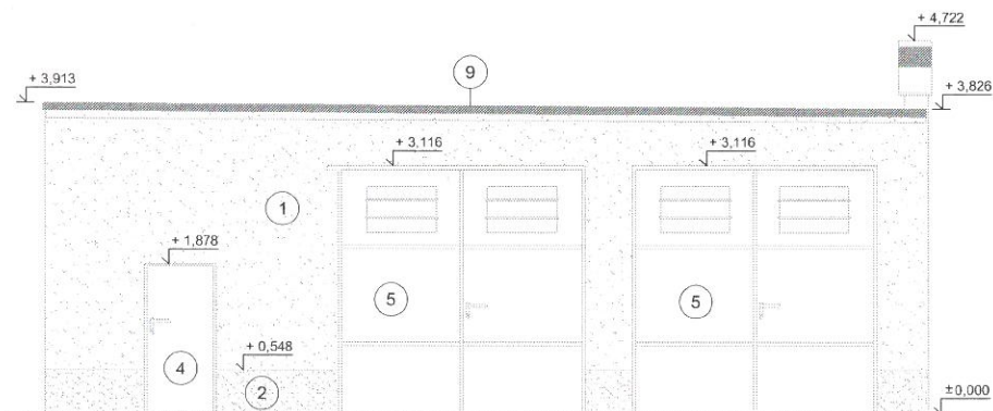
ZÁPADNÍ POHLED
