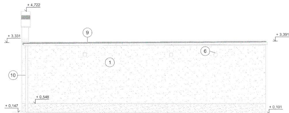
VÝCHODNÍ POHLED
