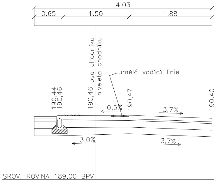
Charakteristický řez—3 úsek—A km 0,060 00
