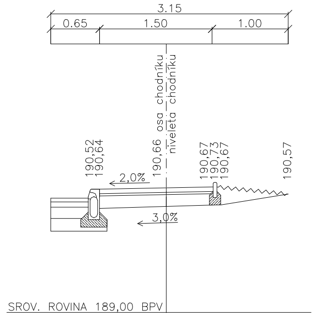
Charakteristický řez—4 úsek—A km 0,080 00
