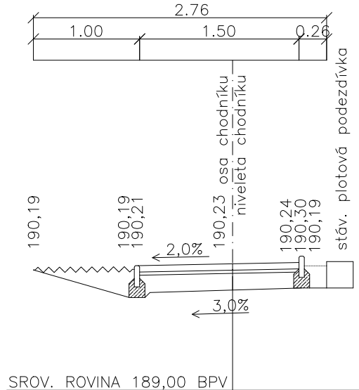
Charakteristický řez—1 úsek—A km 0,020 00
