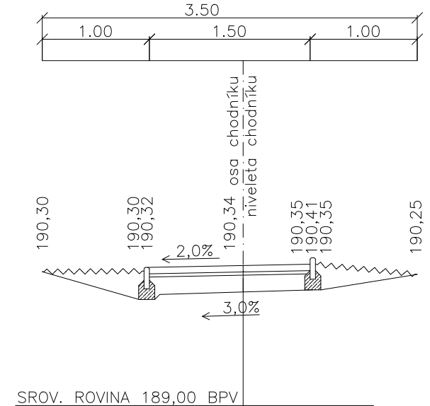
Charakteristický řez—2 úsek—A km 0,040 00
