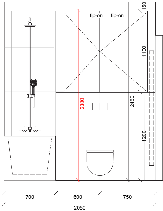
POHLED P2_KOUPELNA_ BYT C3 (zrcadlově), C4, B3 (zrcadlově), B4
