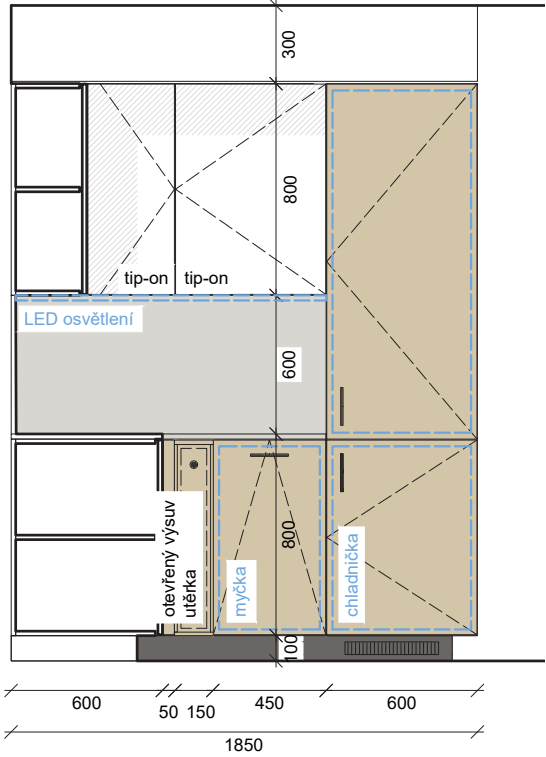
POHLED_KUCHYŇSKÁ LINKA_ BYT B2
