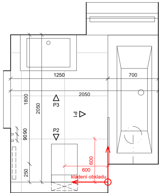
PŮDORYS_KOUPELNA_ BYT C3 (zrcadlově), C4, B3 (zrcadlově), B4
