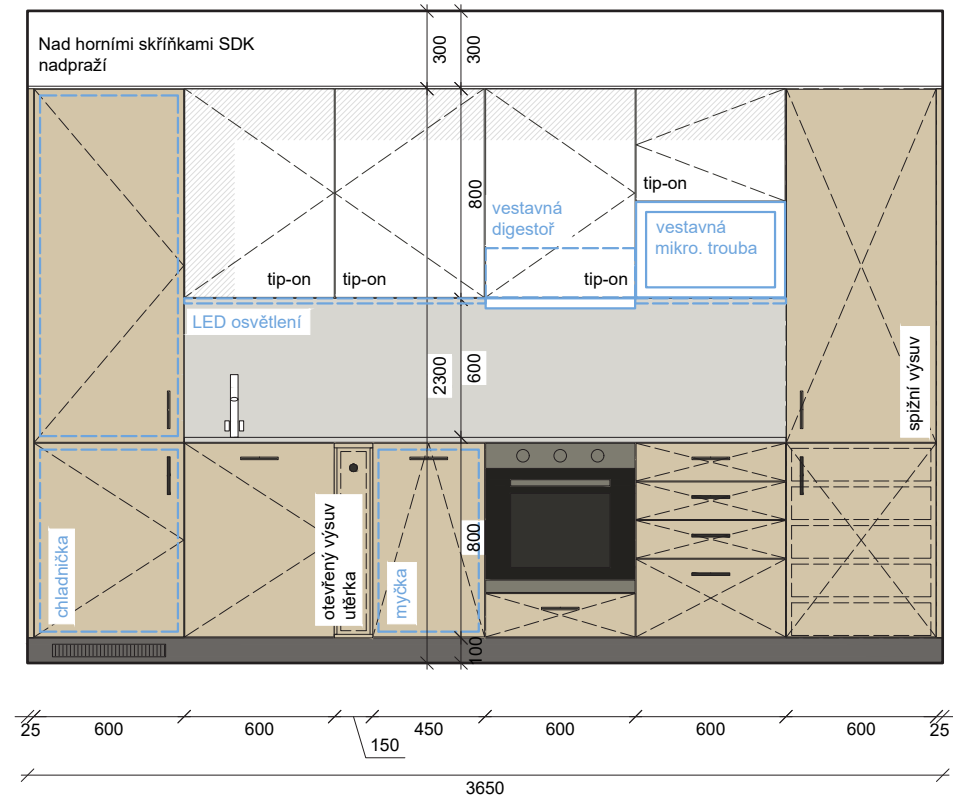
POHLED_KUCHYŇSKÁ LINKA_ BYT A2
