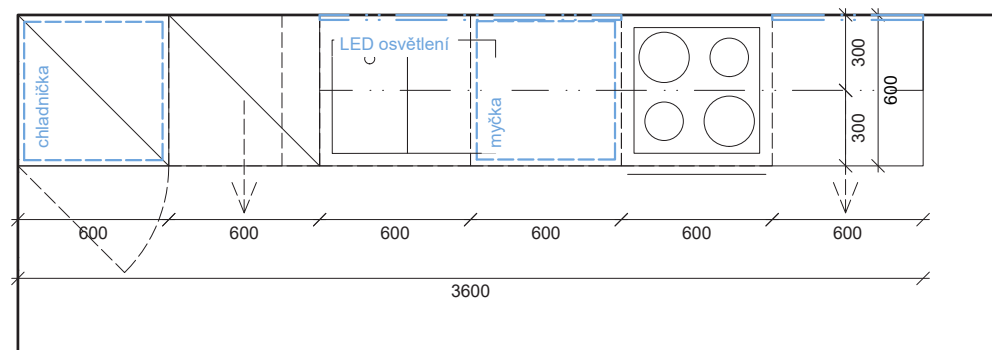
PŮDORYS_KUCHYŇSKÁ LINKA_ BYT B3, B4 (zrcadlořě), C3, C4 (zrcadlořě)
