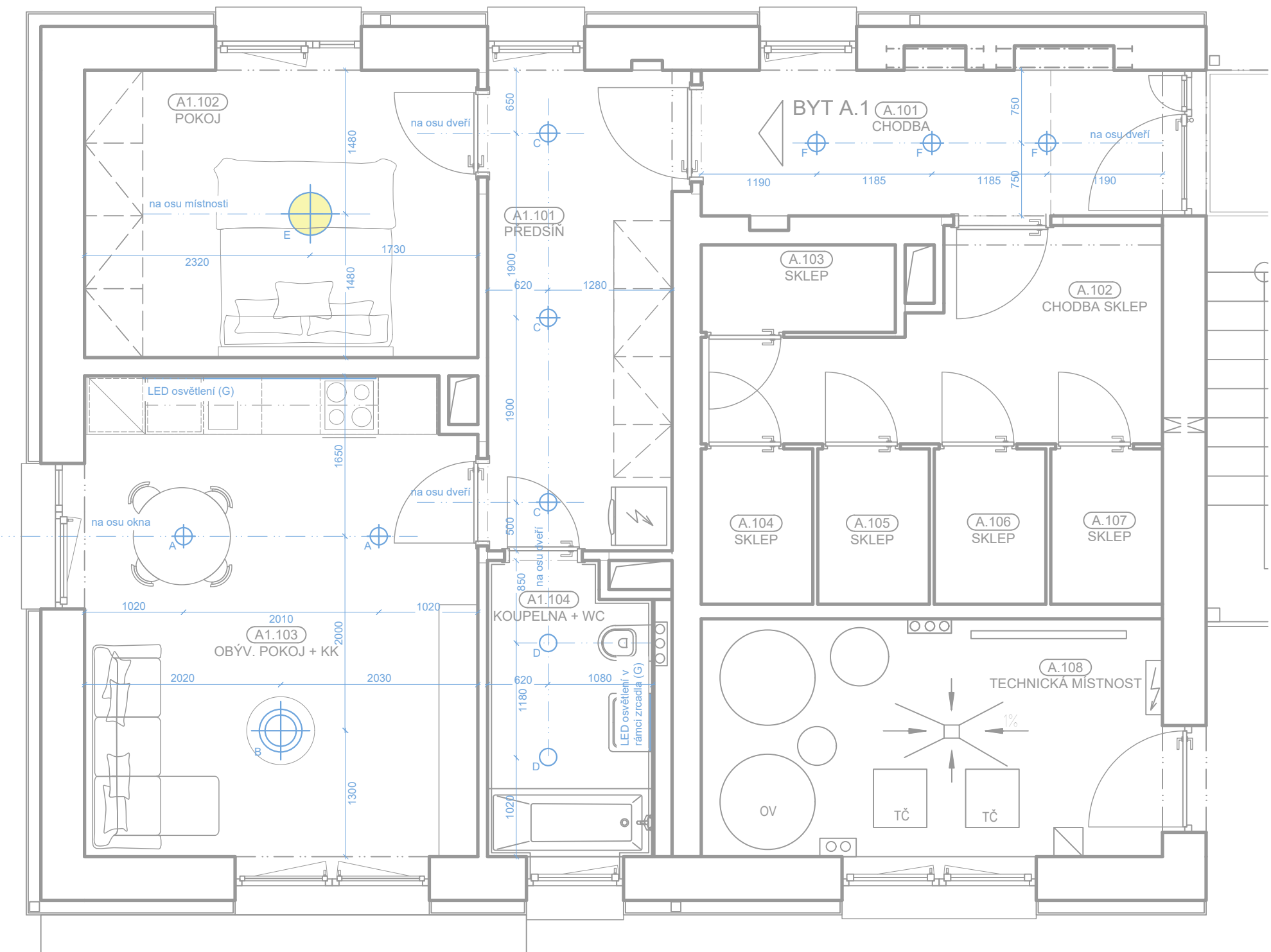
PŮDORYS BYTY A1, A2
