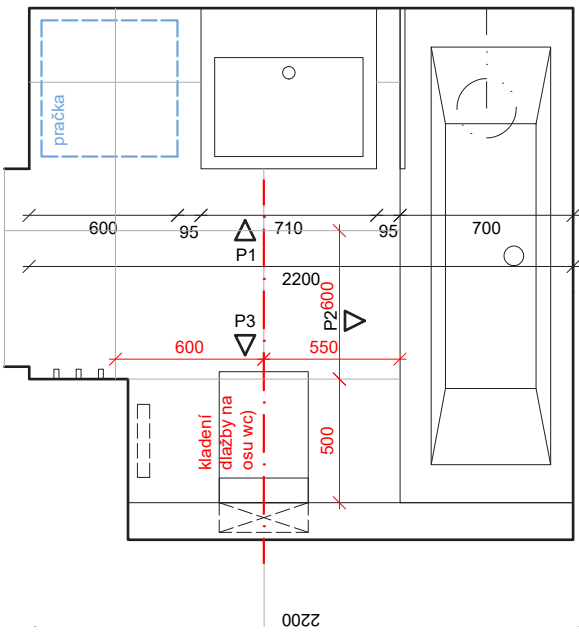
PŮDORYS_KOUPELNA_ BYT B2, C1 (zrcadlově)
