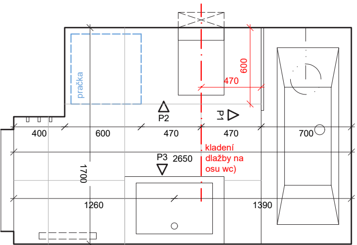
PŮDORYS_KOUPELNA_ BYT A3
