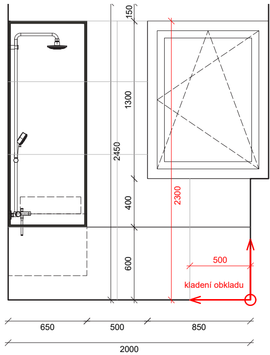
POHLED P2_KOUPELNA_ BYT B1, C2 (zrcadlově)
