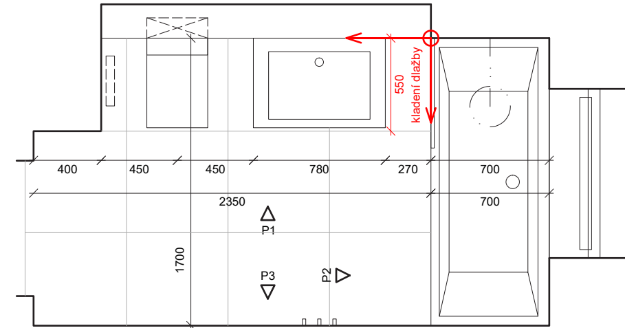
PŮDORYS_KOUPELNA_BYT A2
