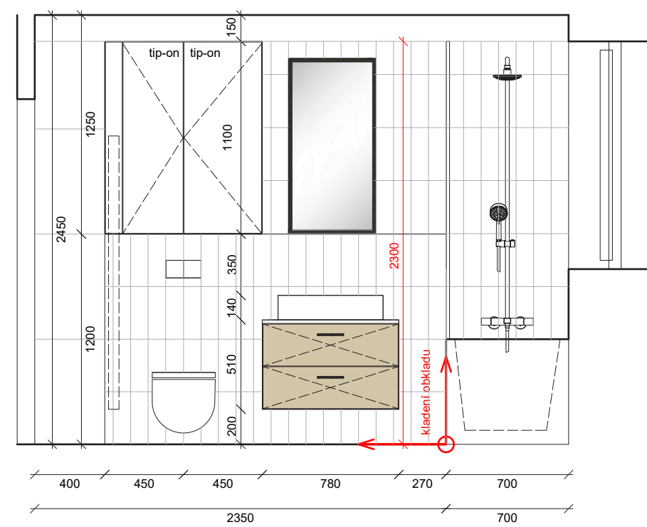
POHLED P1_KOUPELNA_BYT A2
