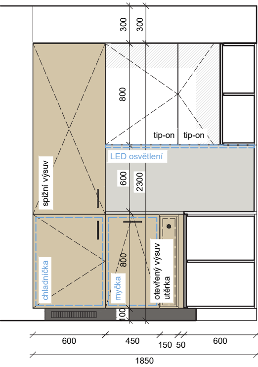
POHLED_KUCHYŇSKÁ LINKA_ BYT C1
