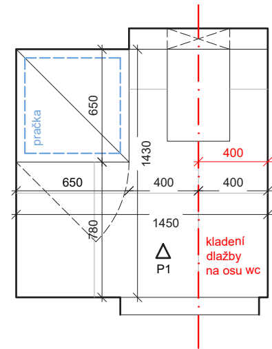
PŮDORYS_WC_ BYT C3 (zrcadlově), C4, B3 (zrcadlově), B4
