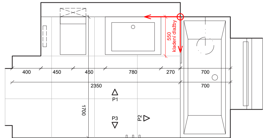
PŮDORYS_KOUPELNA_BYT A1
