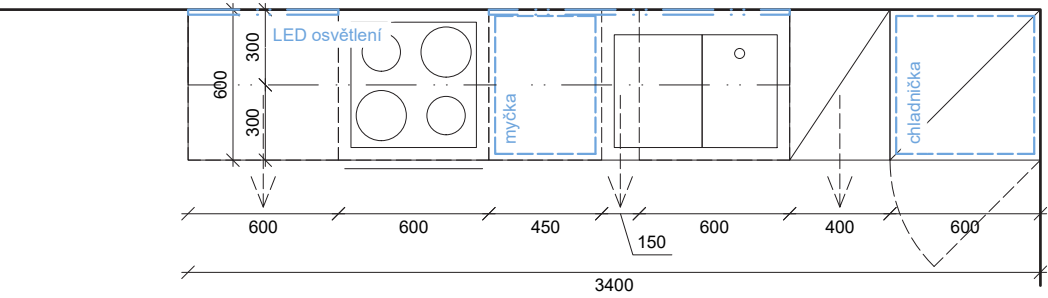
PŮDORYS_KUCHYŇSKÁ LINKA_ BYT C2, BYT B1
