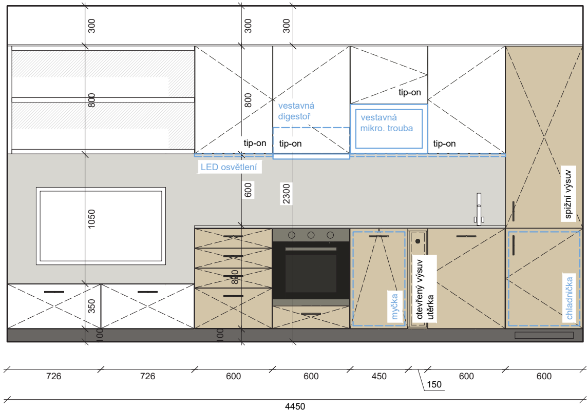
POHLED_KUCHYŇSKÁ LINKA_ BYT A3
