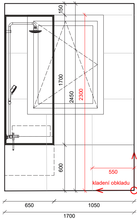
POHLED P2_KOUPELNA_BYT A1_varianta A
