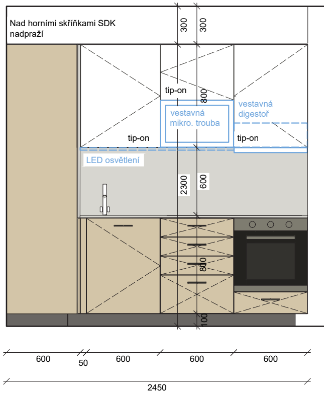
POHLED_KUCHYŇSKÁ LINKA_ BYT C1
