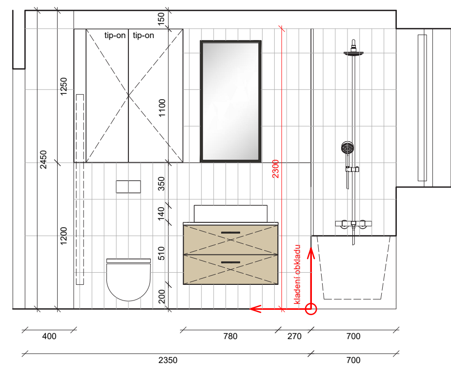
POHLED P1_KOUPELNA_BYT A1
