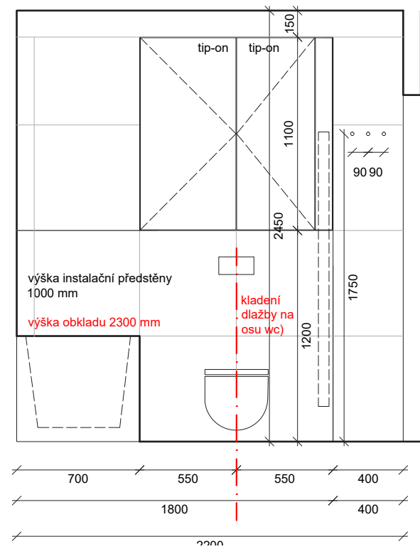
POHLED P3_KOUPELNA_ BYT B2, C1 (zrcadlově)
