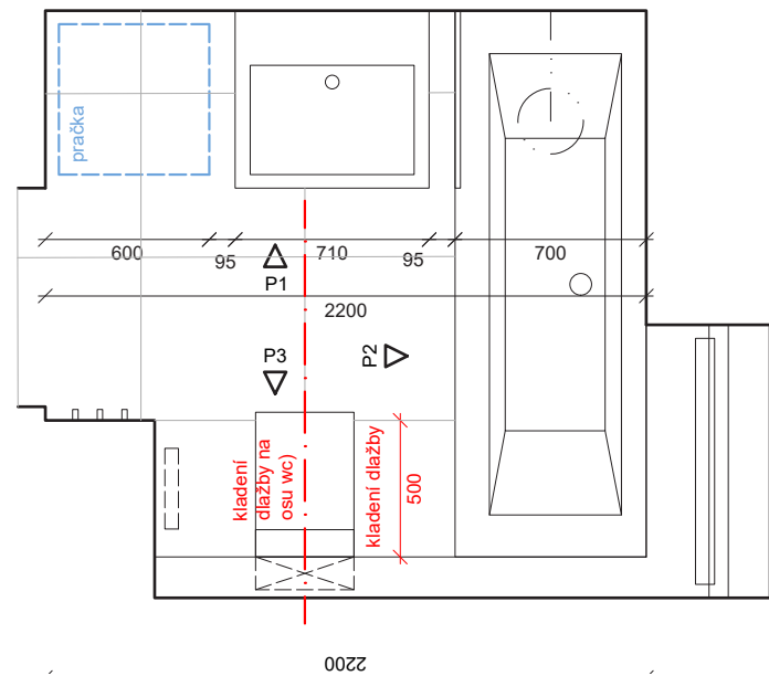
PŮDORYS_KOUPELNA_ BYT B1, C2 (zrcadlově)
