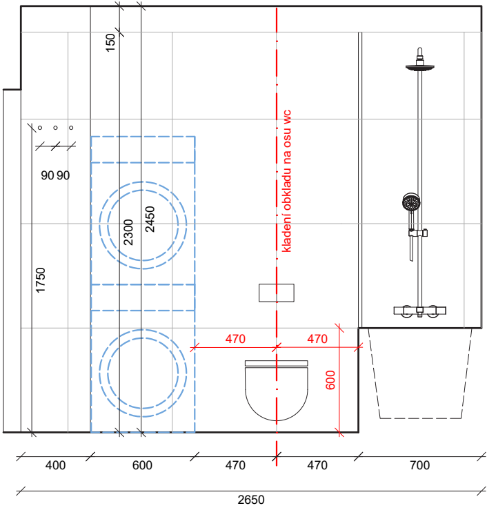
POHLED P2_KOUPELNA_ BYT A3
