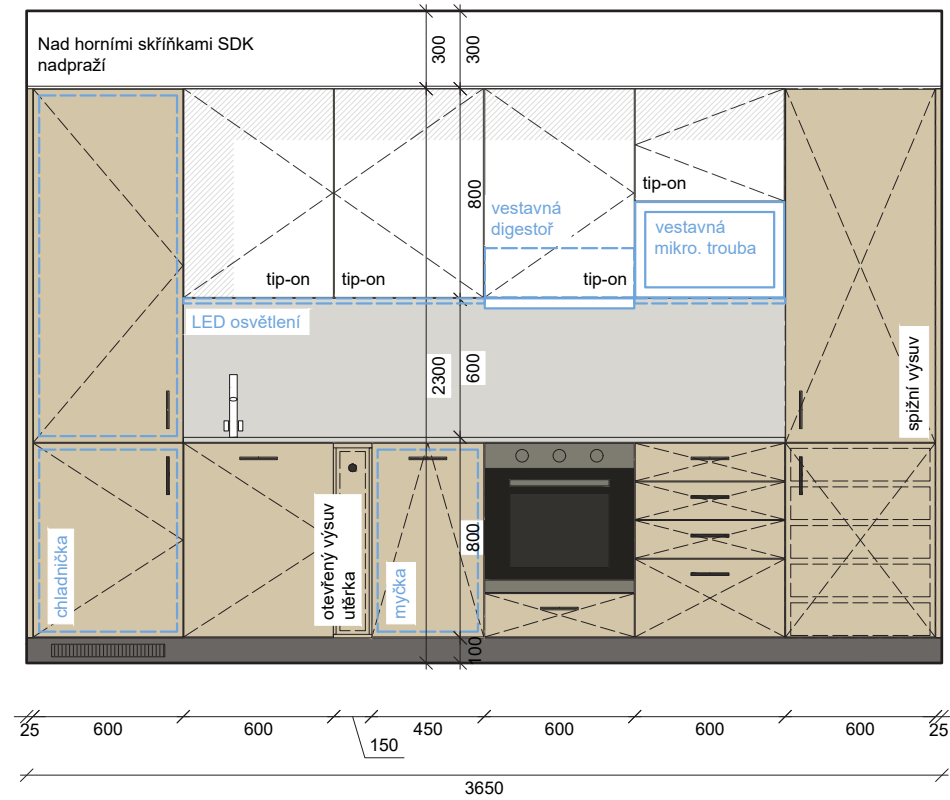
POHLED_KUCHYŇSKÁ LINKA_ BYT A1
