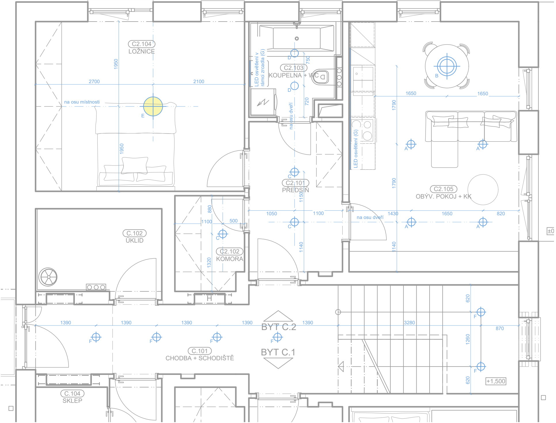
PŮDORYS BYTY B1, C2
