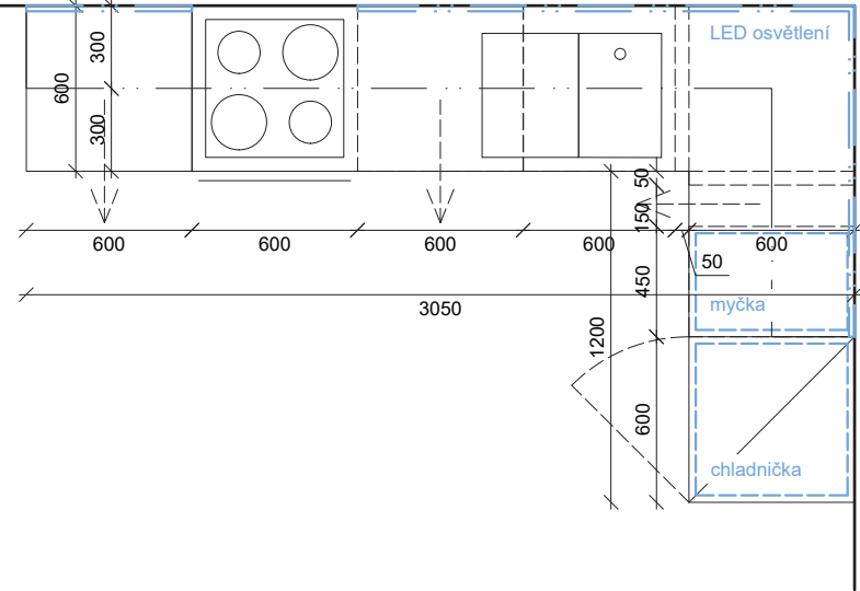
PŮDORYS_KUCHYŇSKÁ LINKA_ BYT B2
