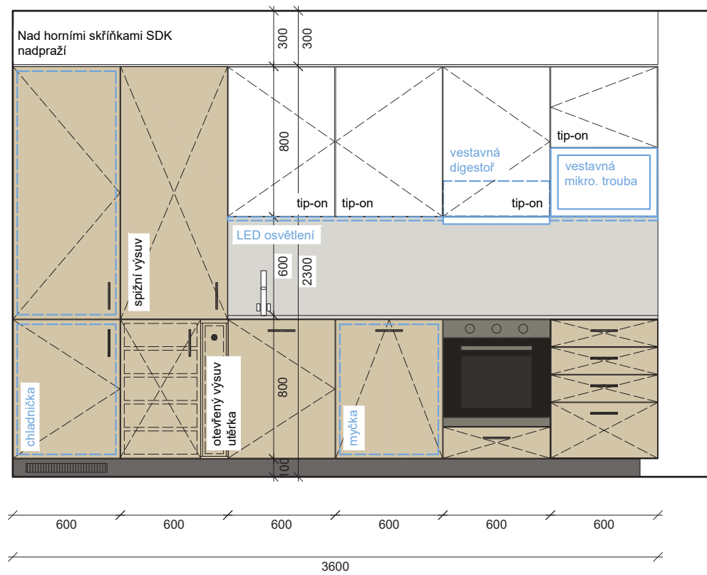
POHLED_KUCHYŇSKÁ LINKA_ BYT B3, B4 (zrcadlořě), C3, C4 (zrcadlořě)
