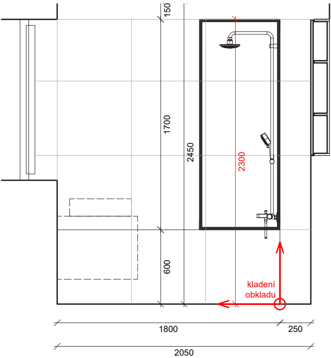
POHLED P1_KOUPELNA_ BYT C3 (zrcadlově), C4, B3 (zrcadlově), B4
