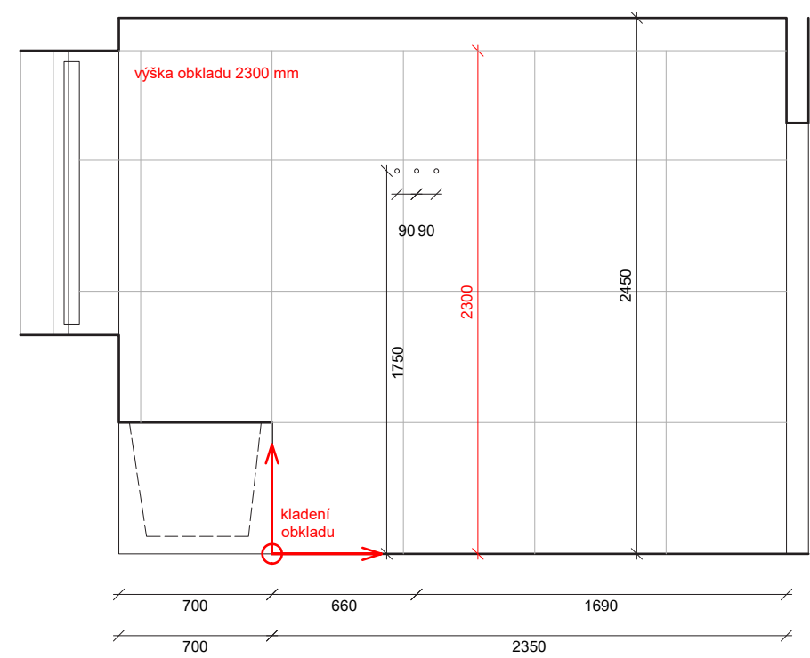
POHLED P3_KOUPELNA_BYT A2
