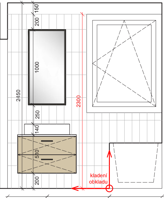
POHLED P3_KOUPELNA_ BYT C3 (zrcadlově), C4, B3 (zrcadlově), B4
