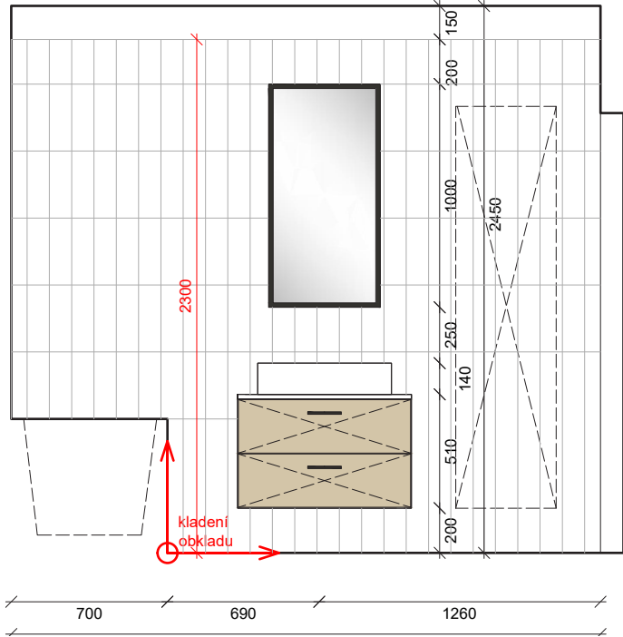
POHLED P3_KOUPELNA_ BYT A3
