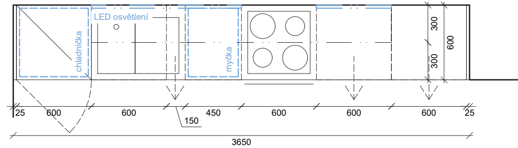
PŮDORYS_KUCHYŇSKÁ LINKA_ BYT A1
