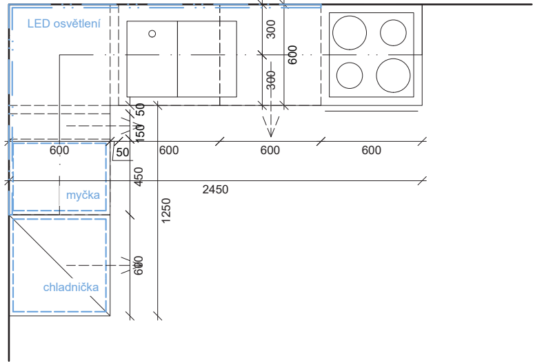
PŮDORYS_KUCHYŇSKÁ LINKA_ BYT C1
