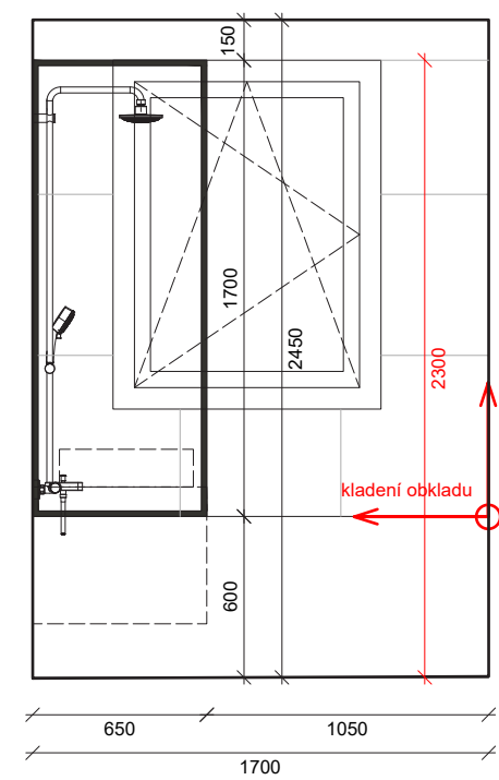
POHLED P2_KOUPELNA_BYT A2
