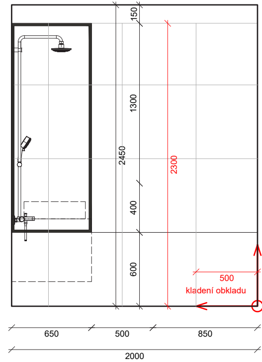
POHLED P2_KOUPELNA_ BYT B2, C1 (zrcadlově)
