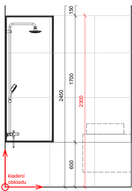
POHLED P1_KOUPELNA_ BYT A3
