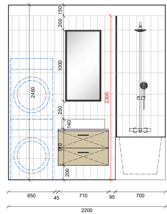
POHLED P1_KOUPELNA_ BYT B2, C1 (zrcadlově)
