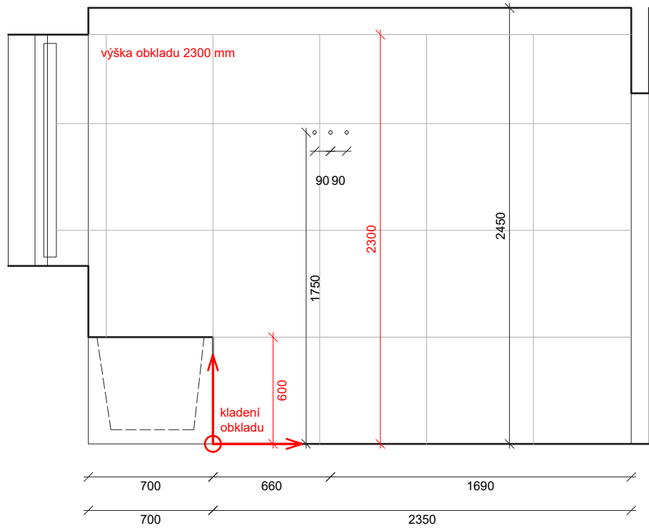
POHLED P3_KOUPELNA_BYT A1
