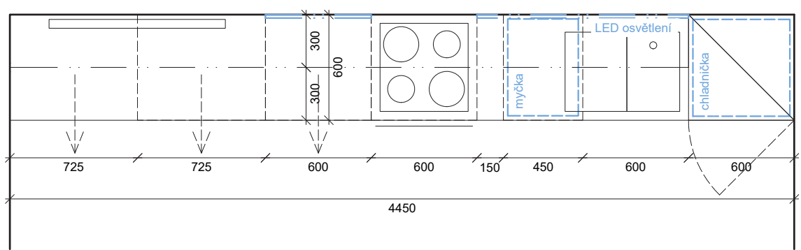
PŮDORYS_KUCHYŇSKÁ LINKA_ BYT A3
