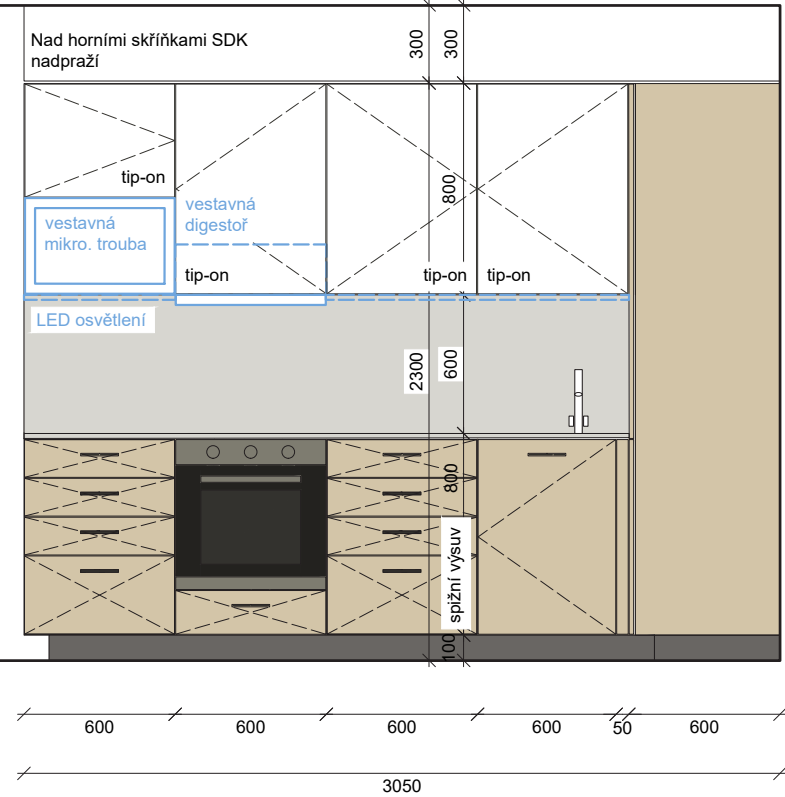
POHLED_KUCHYŇSKÁ LINKA_ BYT B2
