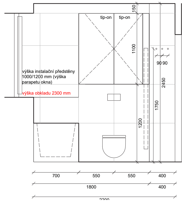
POHLED P3_KOUPELNA_ BYT B1, C2 (zrcadlově)
