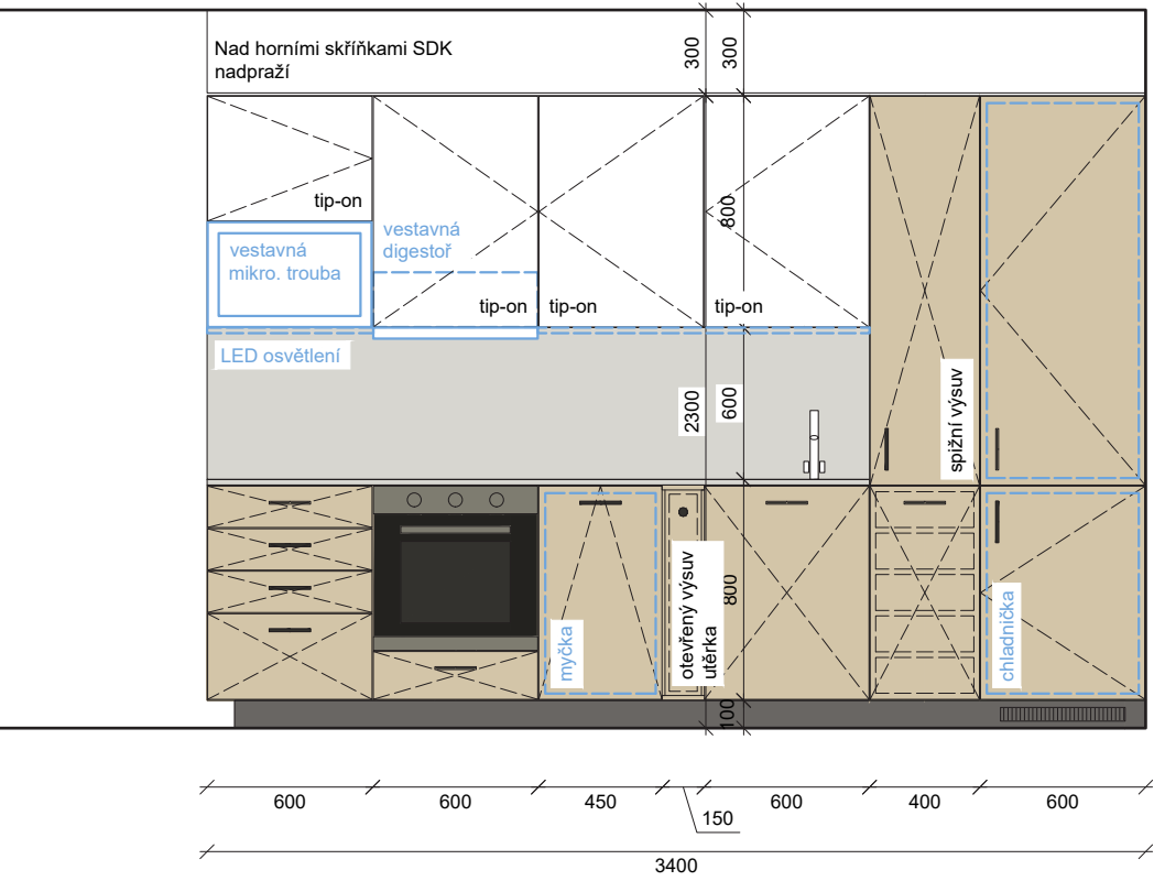
POHLED_KUCHYŇSKÁ LINKA_ BYT C2, BYT B1 (zrca-
