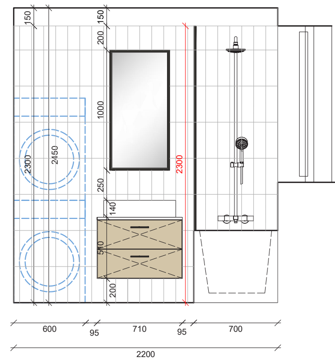
POHLED P1_KOUPELNA_ BYT B1, C2 (zrcadlově)
