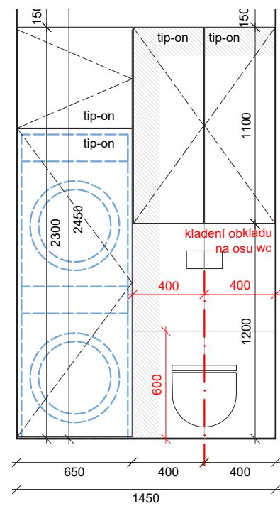
POHLED P1_WC_ BYT C3 (zrcadlově), C4, B3 (zrcadlově), B4
