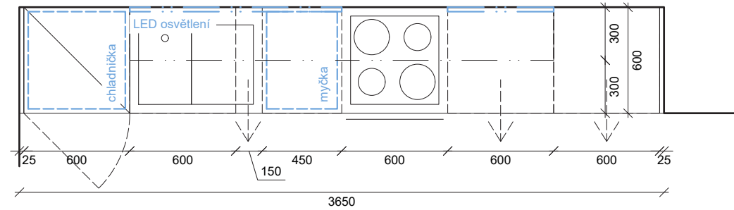
PŮDORYS_KUCHYŇSKÁ LINKA_ BYT A2
