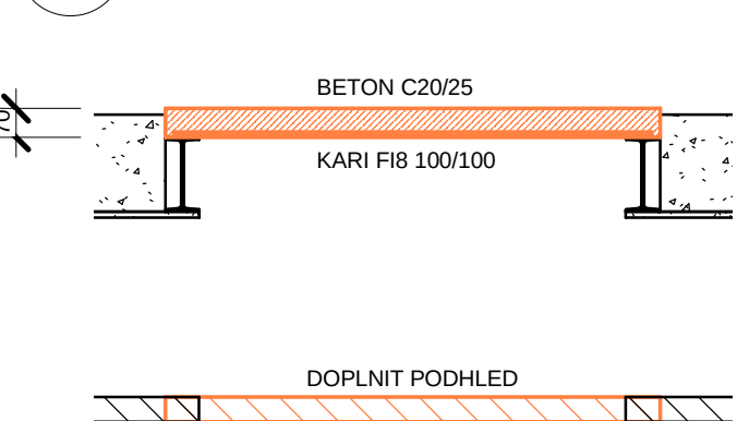
11 DETAIL BETONÁŽE SVĚTLÍKU 2 ŘEZ 1 : 20
