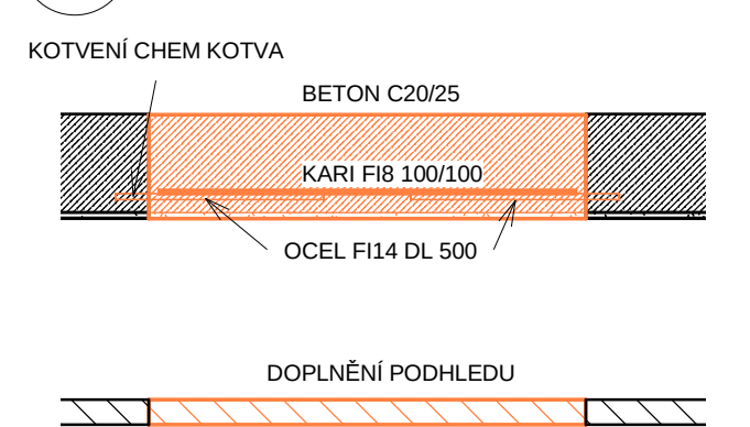
10 DETAIL BETONÁŽE SVĚTLÍKU 1 ŘEZ 1 : 20
