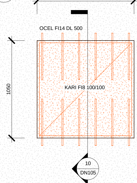
10 DETAIL BETONÁŽE SVĚTLÍKU 1 ŘEZ 1 : 20
