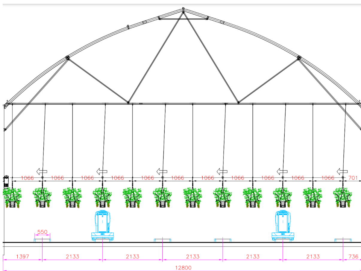
Obrázek 2 Schéma rozložení kolejnic vertikálně
