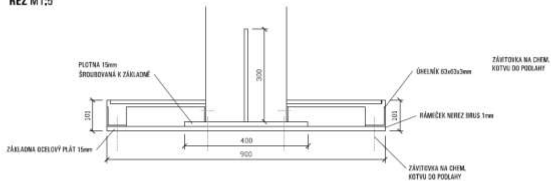
ŘEZ M1:5
