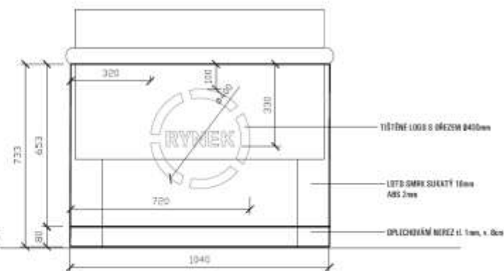
POHLED ČELNÍ M1:20
