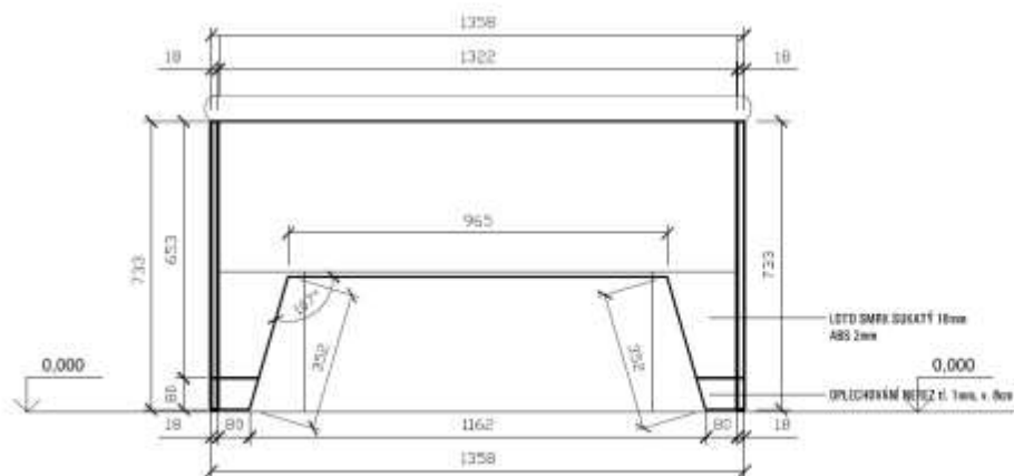
POHLED BOČNÍ M1:20
