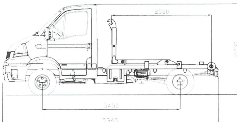
FIAT DUCATO rozvor 3450 mm + CS.NH 2,5/25L
