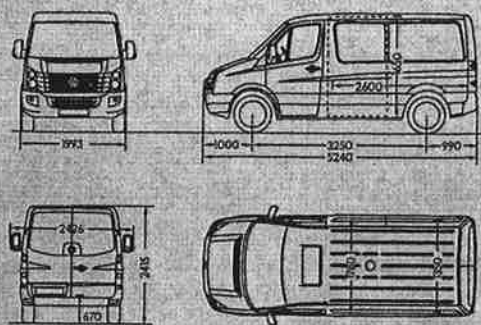
Crafter 30/35 kombi, krátký rozvor se základní střechou
