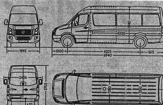
Crafter 35 kombi, dlouhý rozvor s vysokou střechou
