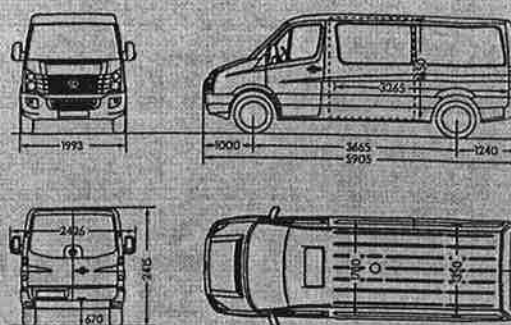
Crafter 30/35 kombi, střední rozvor se základní střechou
