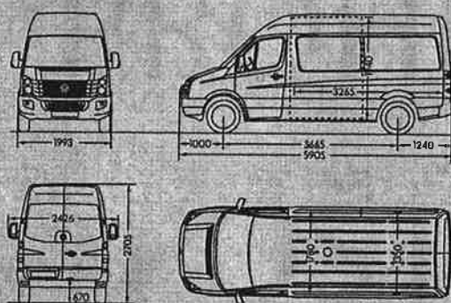
Crafter 30/35 kombi, střední rozvor s vysokou střechou
