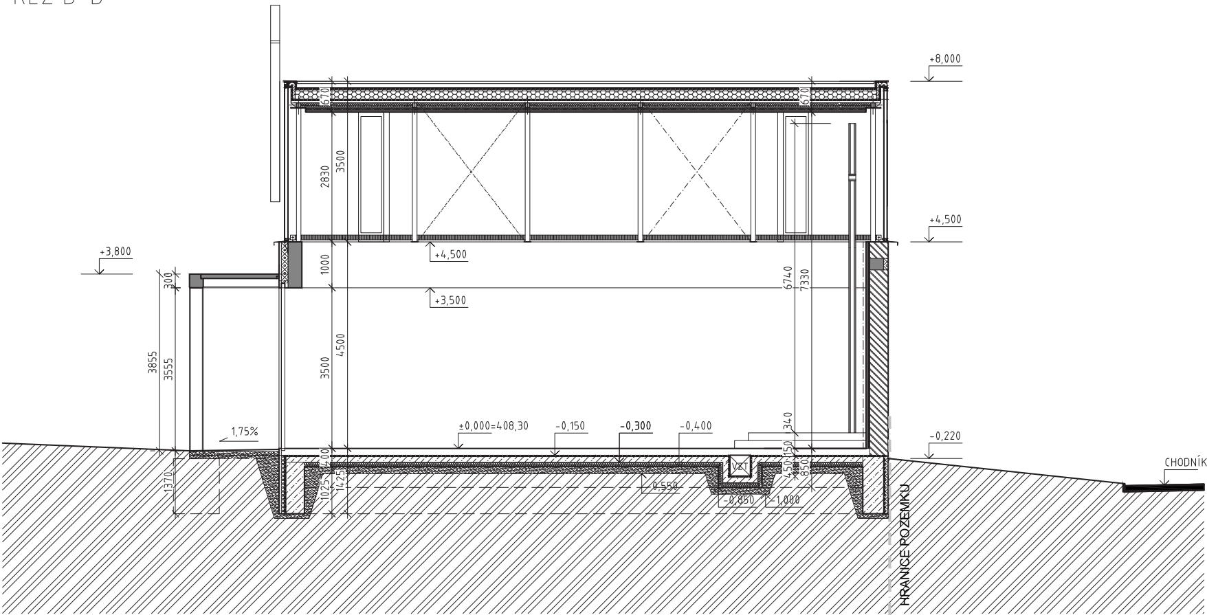
ŘEZ B-B'
