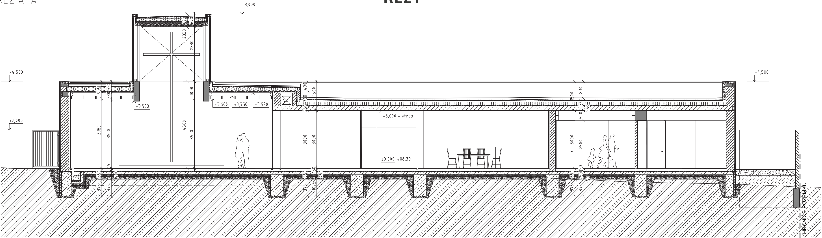
ŘEZ A-A'
