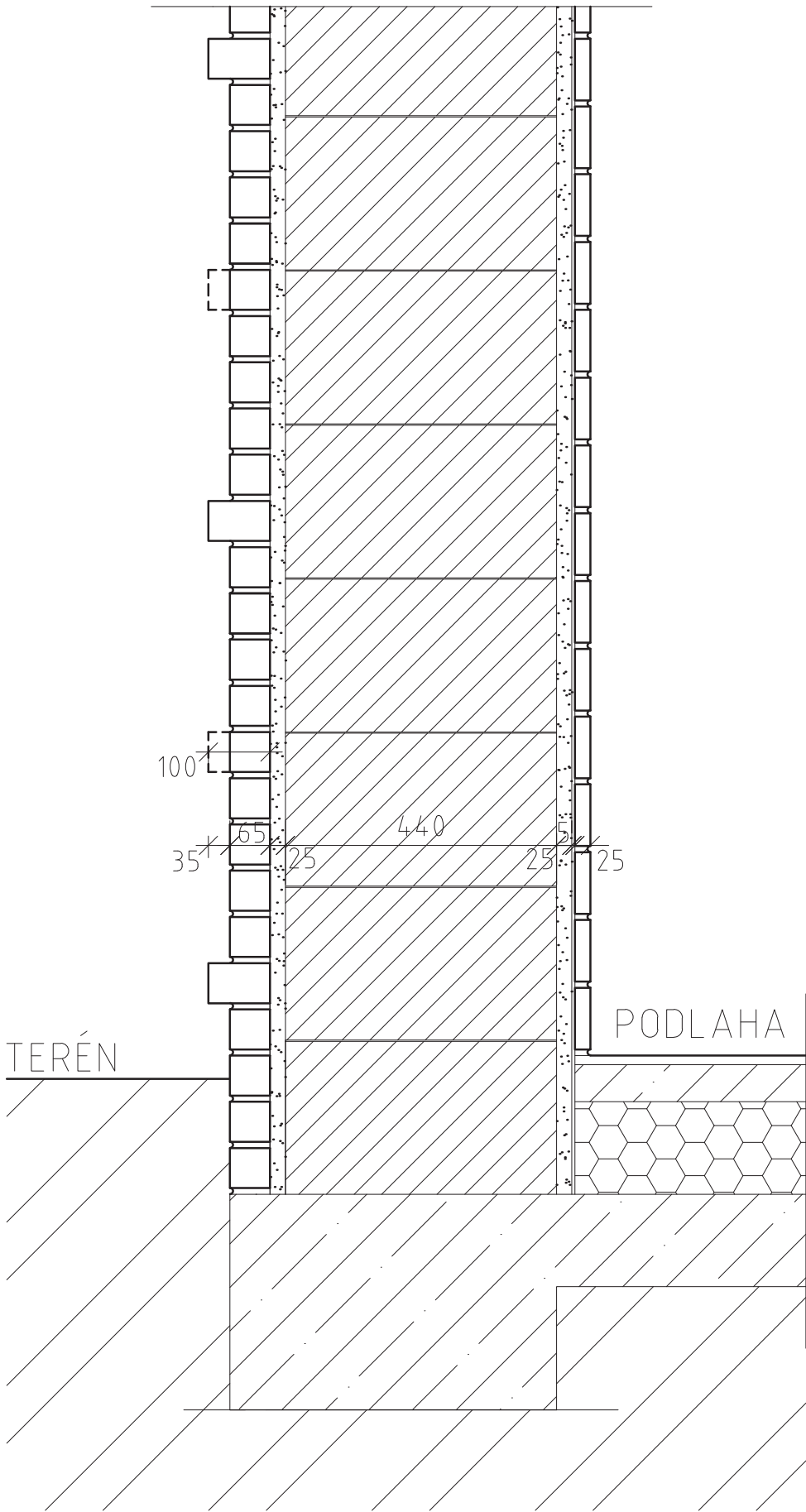
ŘEZ:
