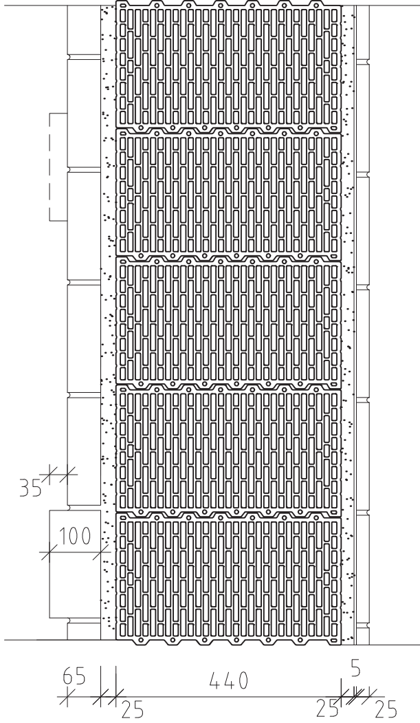
PŮDORYS:
