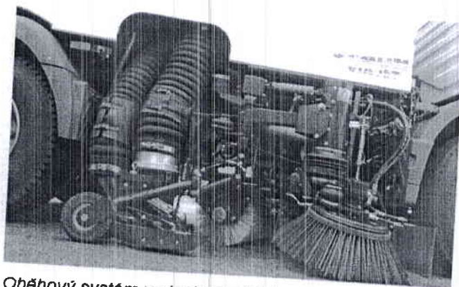
Oběhový systém vzduchu s přífukem do sacího vozíku vzadu proti směru jízdy
