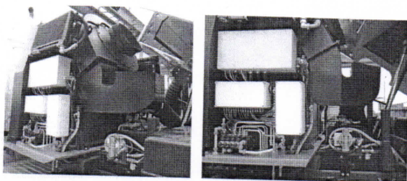
Vodotěsné provedení elektrické a elektro-pneumatické instalace, centrální umístění vlevo pod karosérií zmetací nástavby
