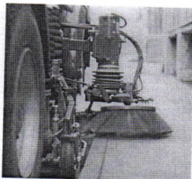
Teleskopické zavěšení krajního kartáče, možnost dvouúrovňového metení, z kabiny měnitelný sklon kartáče
