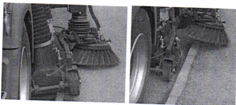
Stranově výkyvný sací vozík s kopírováním nerovností, stranově výkyvný výložník talířového zametacího kartáče
