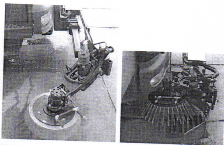
Přední přídavný kartáč, příčně teleskopický o 500 mm, stranově výkyvný, možnost použití agresivního lanového výpletu
