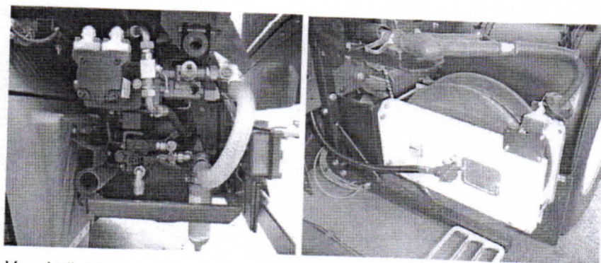
Vysokotlaké vodní čepadlo Speck 100 bar/15 lit/min, naviják, hadice a pistole
