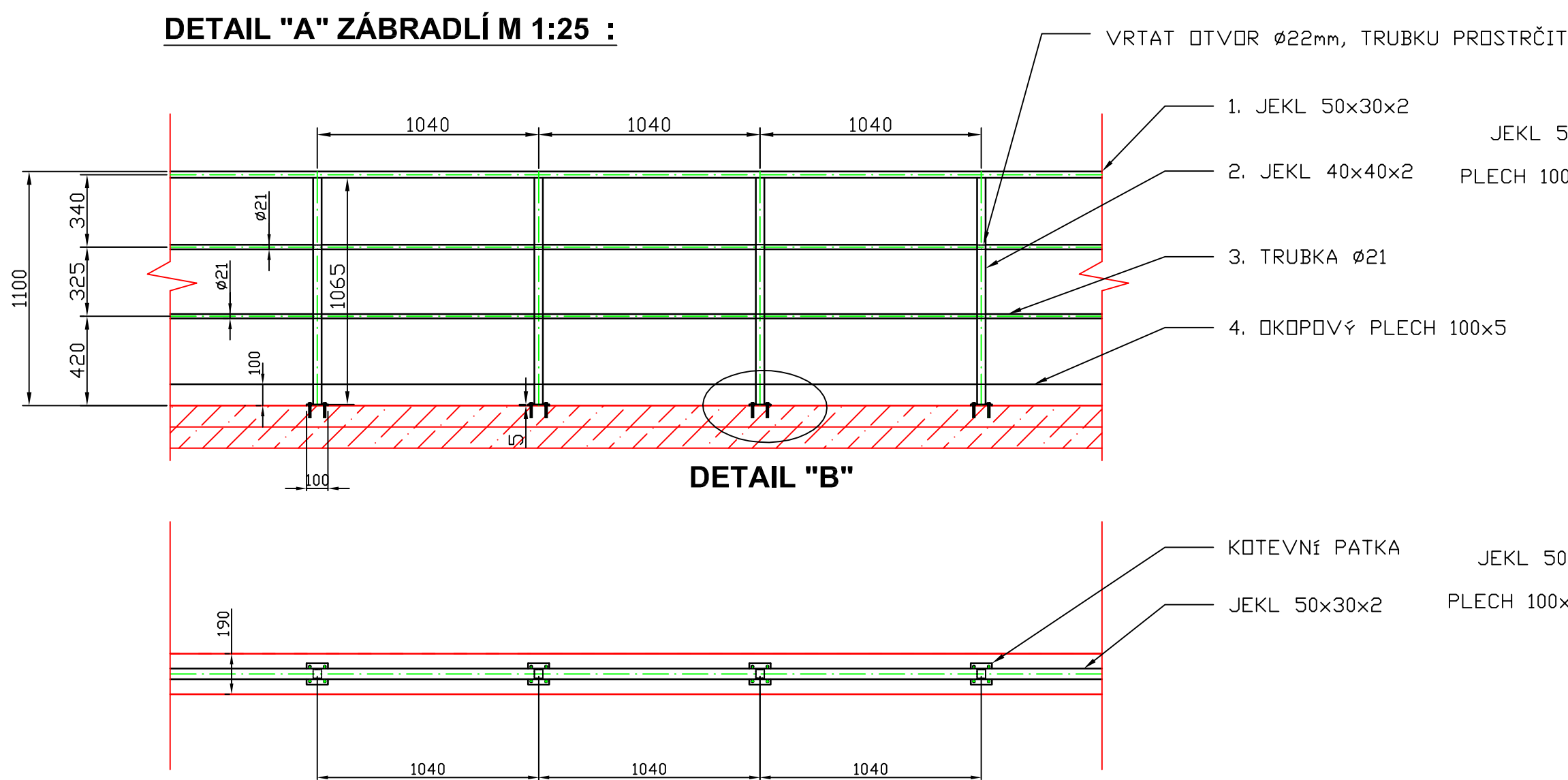
DETAIL "A" ZÁBRADLÍ M 1:25 :
