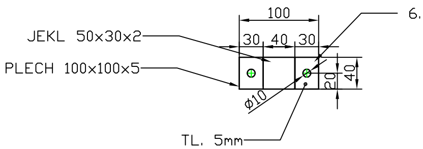
DETAIL "C" KOTEVNÍ PATKA M1:10 : - 2ks
