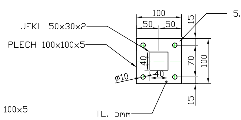
DETAIL "B" KOTEVNÍ PATKA M1:10 : - 71ks
