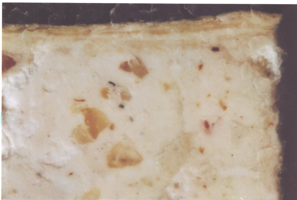
Obrázek 5- mikronábrus vrstvou B, pohled v odraženém světle, zvětšeno 150 x
