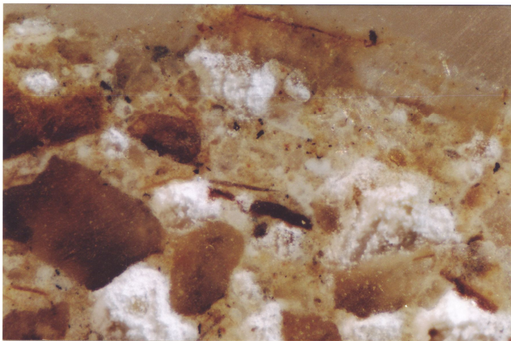
Obrázek 6 – mikronábrus vrstvou C, pohled v odraženém světle, zvětšeno 300 x
