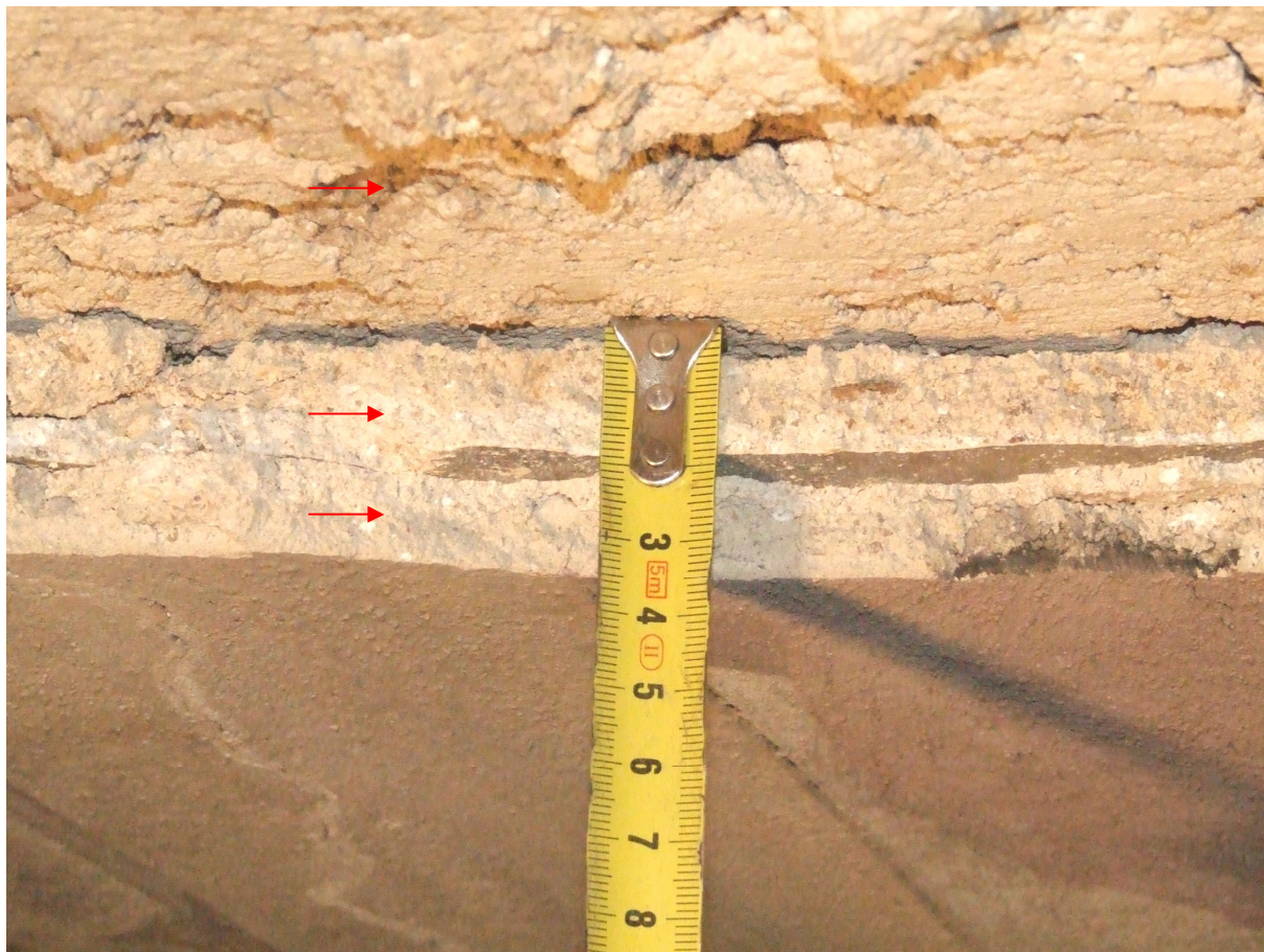
Obrázek 1 – tři vrstvy omítek : 1-jádrová okrová, středně zrnitá vápenná omítka nestejnoměrné síly, vyrovnávající cihelné zdivo klenby 2-cca 1.5 cm vysoký, středně až hrubý štuk se závalky vápna s hlazeným vápenným povrchem a secco malbou – viz obr 3 3-cca 1 cm vysoký, jemně až středně zrnitý naředlý štuk s jemně zrnitým povrchem a okrovou lazurou v al fresco
