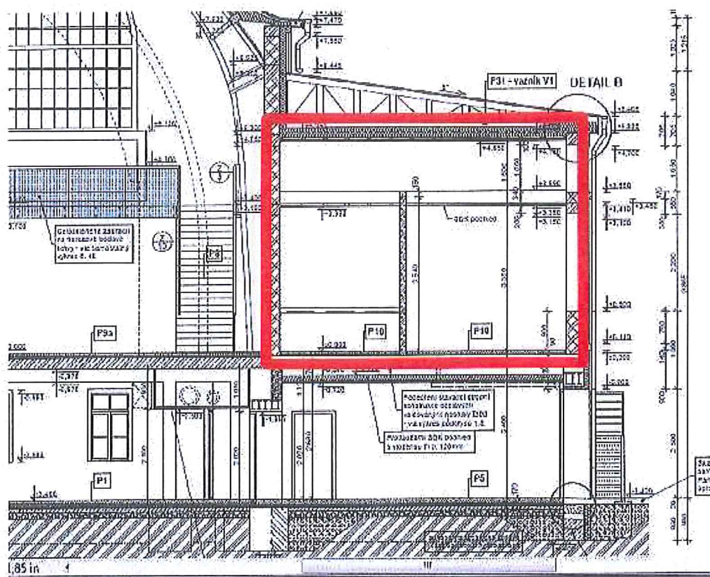
Obrázek 2: Řez sálem
