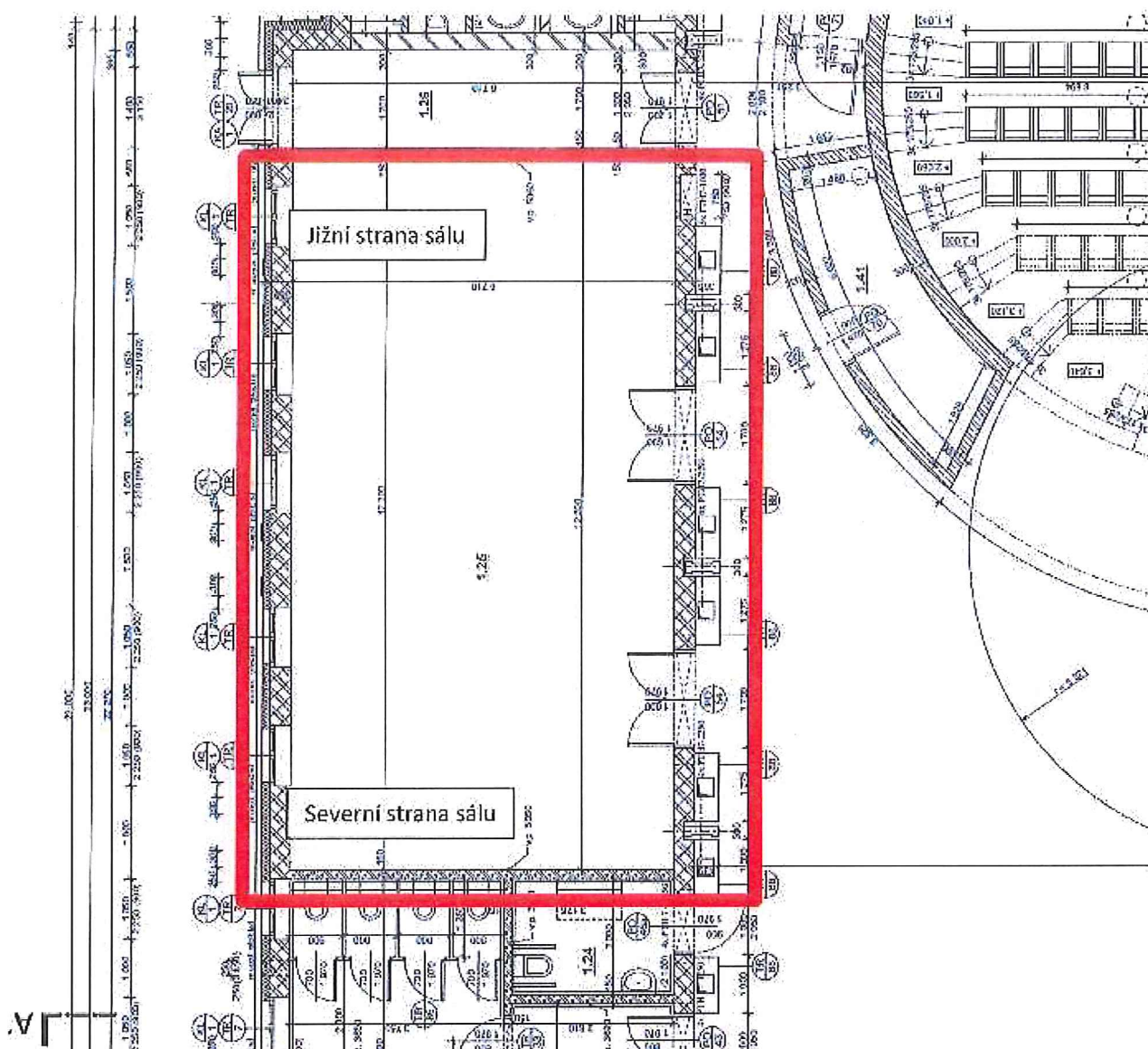
Obrázek 1: Půdorys sálu
