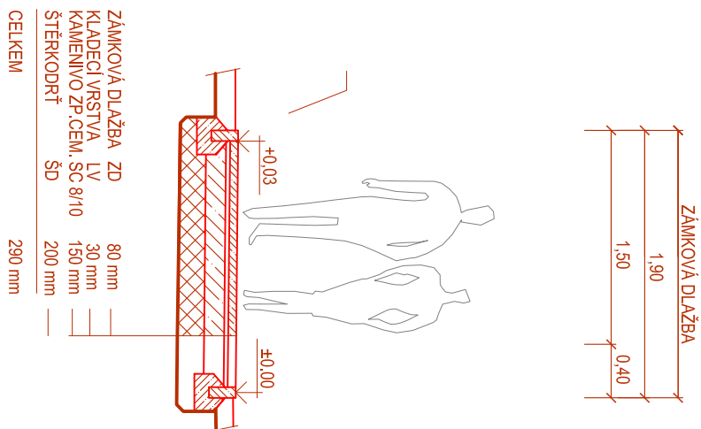
CHODNÍK V KŘÍŽENÍ VJEZDU - VZOROVÝ ŘEZ 1 : 50
