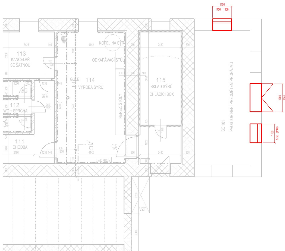
Obr. 1 – repase oken a dveří (položka č. 6 a č. 5)
