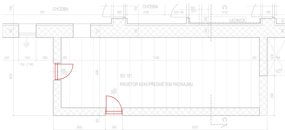
Obr. 2 – doplnění nových dveří (položka č. 3 a č. 4)
