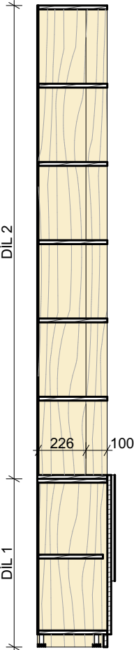
řez příčný M 1:25
