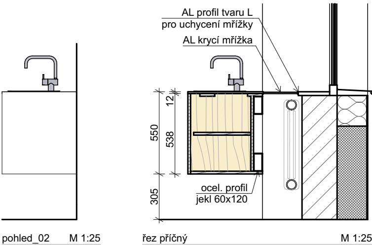
pohled_02 M 1:25 řez příčný M 1:25
