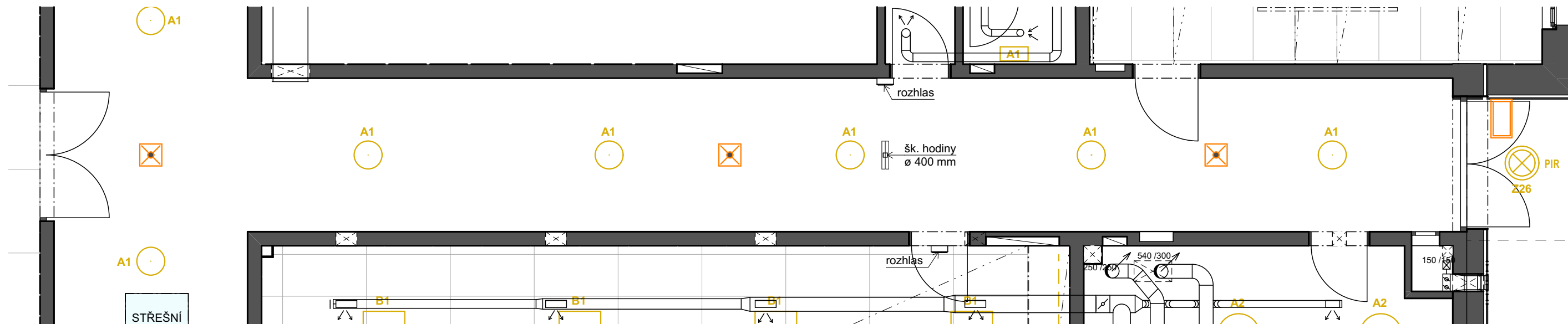
PŮDORYS PODHLEDU
