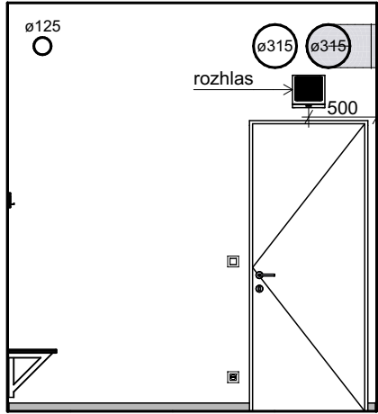
POHLED 1.14_03
