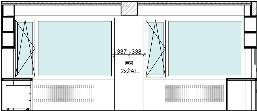
POHLED 1.33_03
