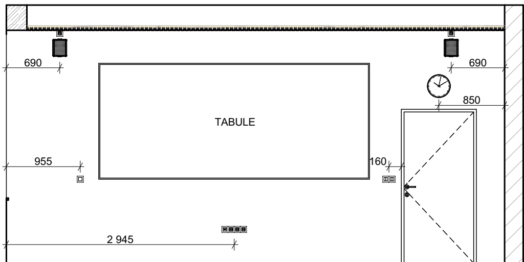
POHLED 2.24_02
