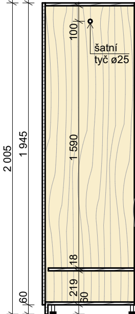
řez příčný M 1:25
