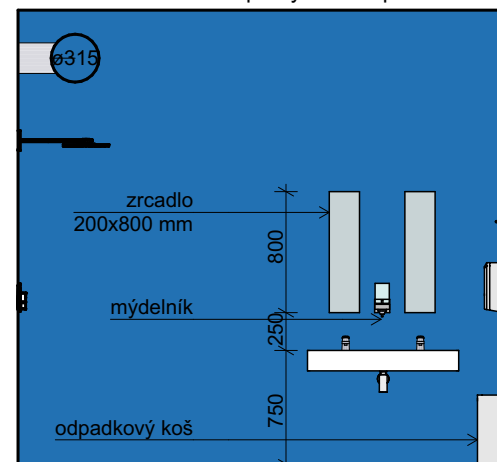
POHLED 1.10_05
