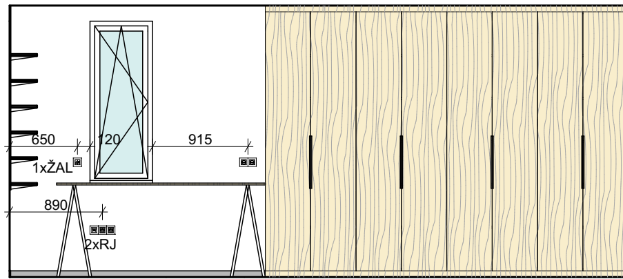
POHLED 2.11_02
