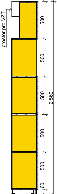
řez příčný
