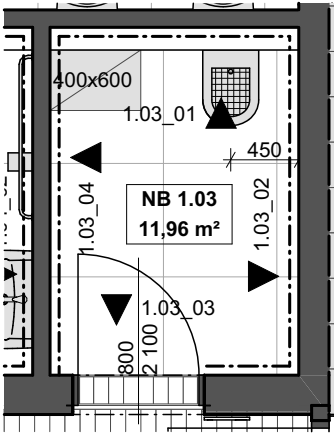
PŮDORYS
