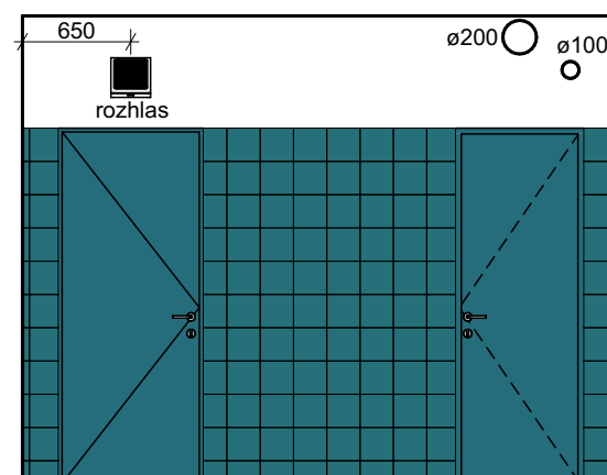
POHLED WC 1.06_05
