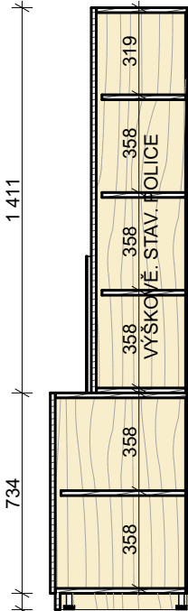
řez příčný M 1:25
