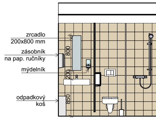
POHLED 2.10_04
