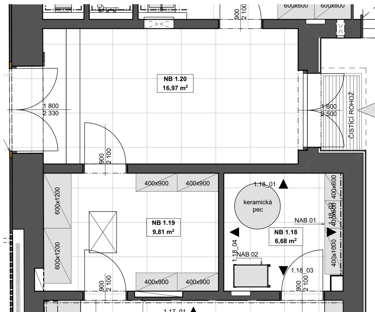
PŮDORYS
