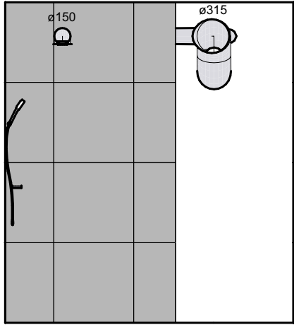
POHLED 1.15_03
