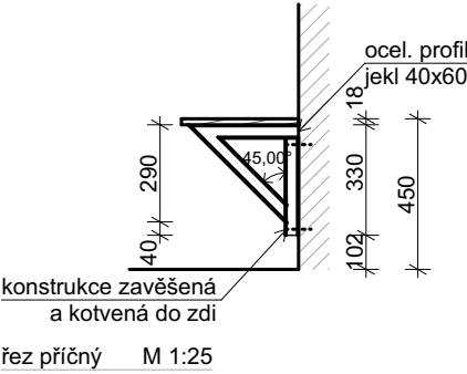
řez příčný M 1:25
