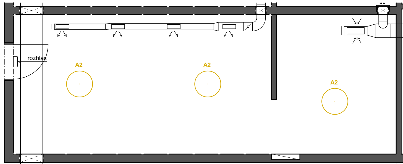
PŮDORYS PODHLEDU
