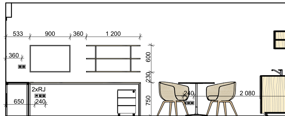
POHLED 1.28_04
