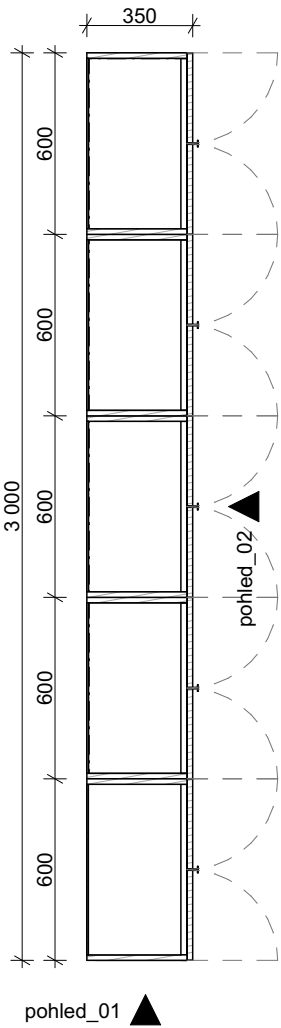
půdorys M 1:25
