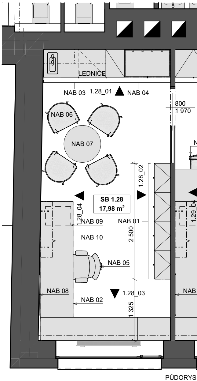
PŮDORYS
