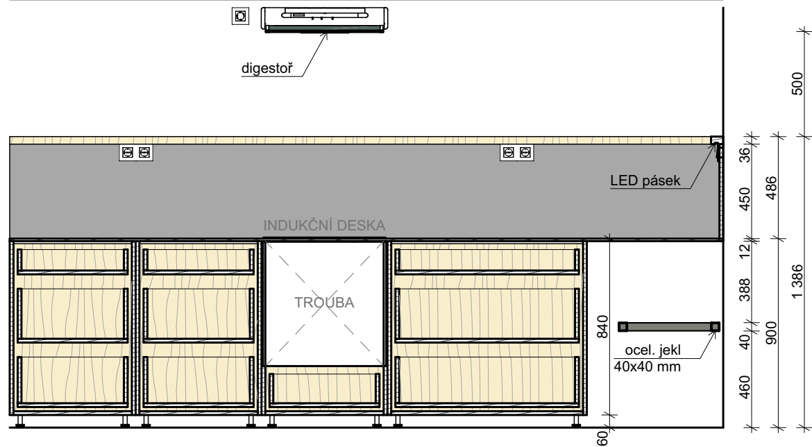
řez podélný 02 M 1:25
