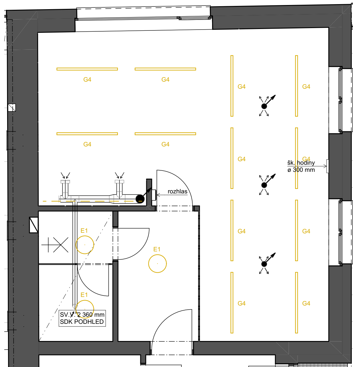
PŮDORYS PODHLEDU
