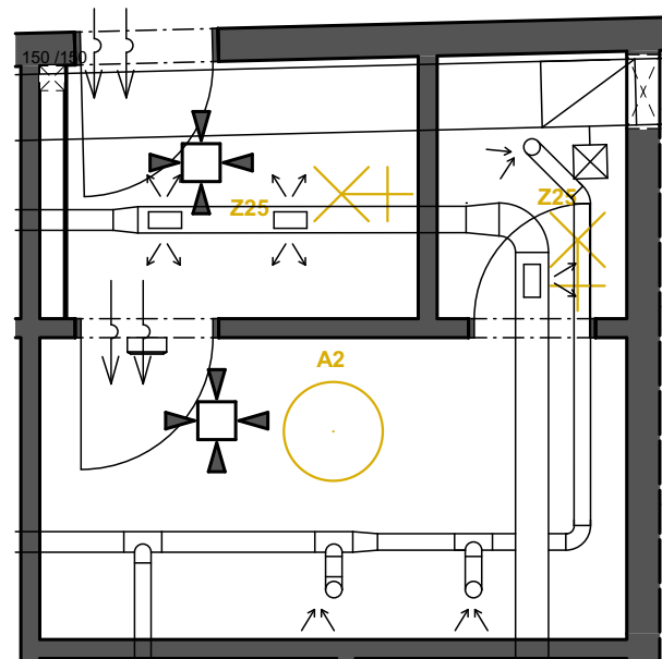
PŮDORYS PODHLEDU
