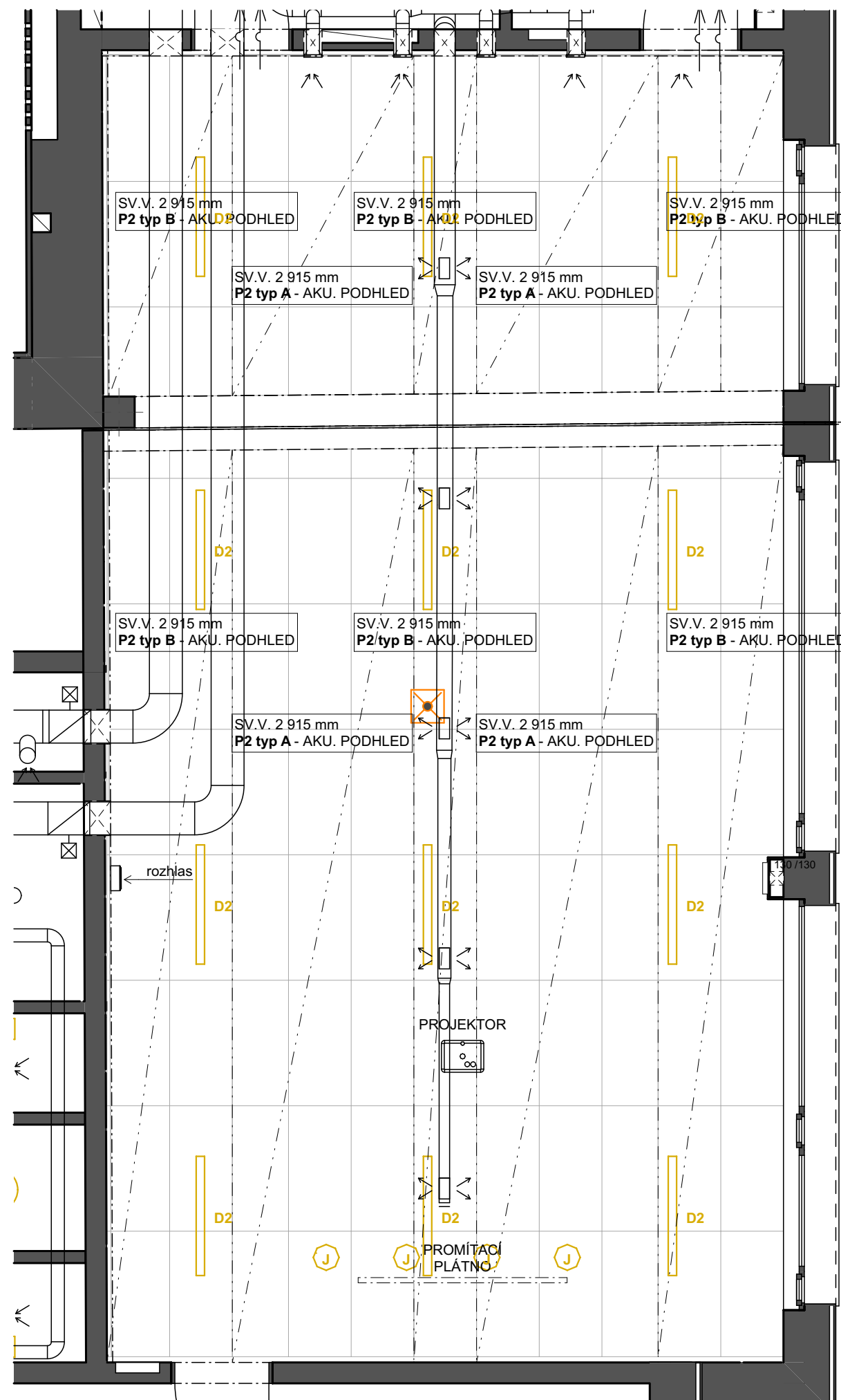
PŮDORYS PODHLEDU
