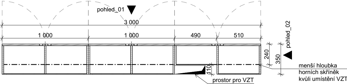
půdorys
