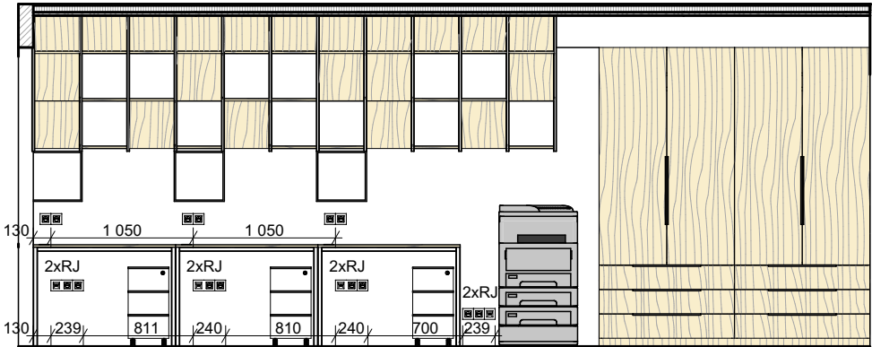
POHLED 1.33_04
