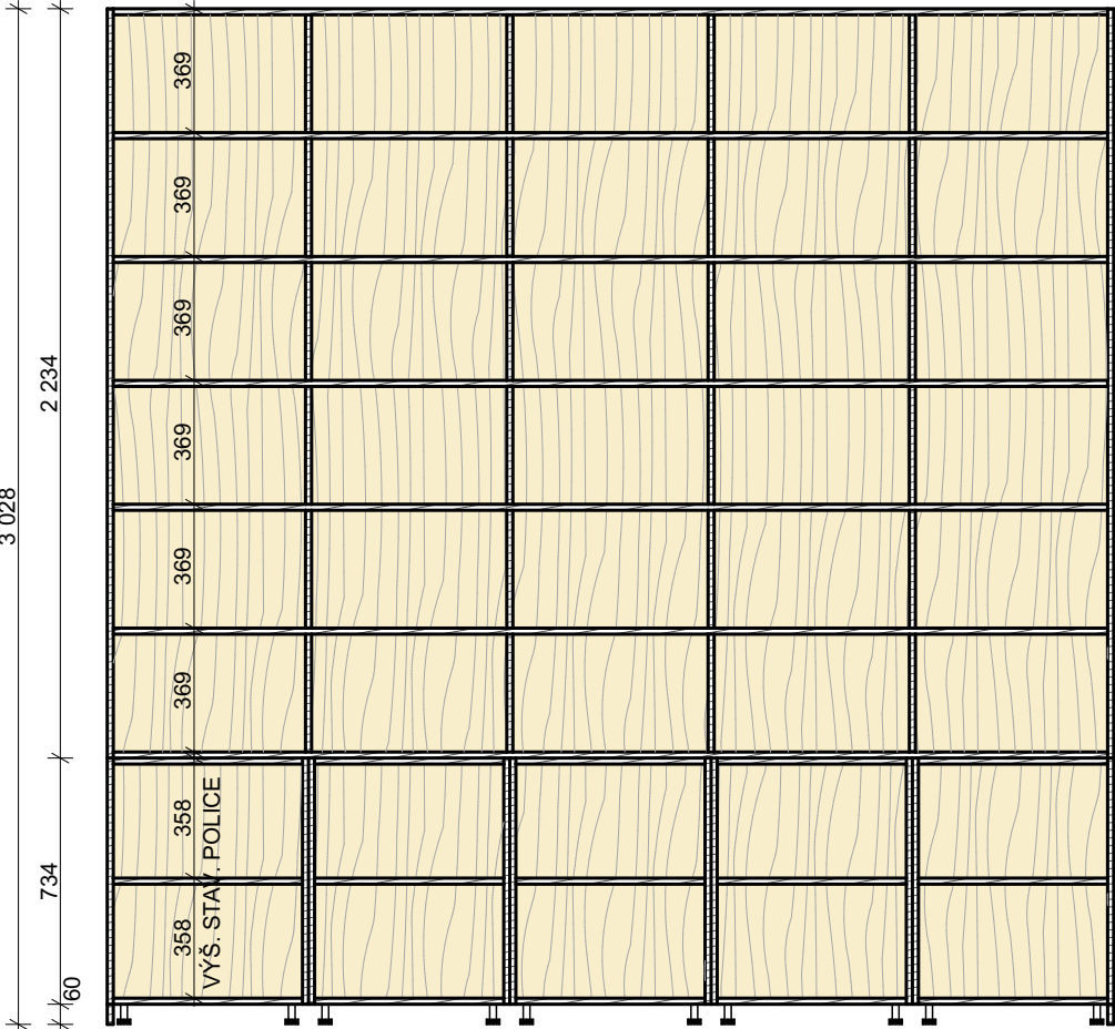
řez podélný M 1:25
