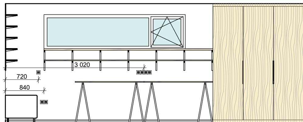
POHLED 2.07_01
