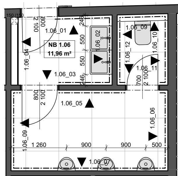
PŮDORYS
