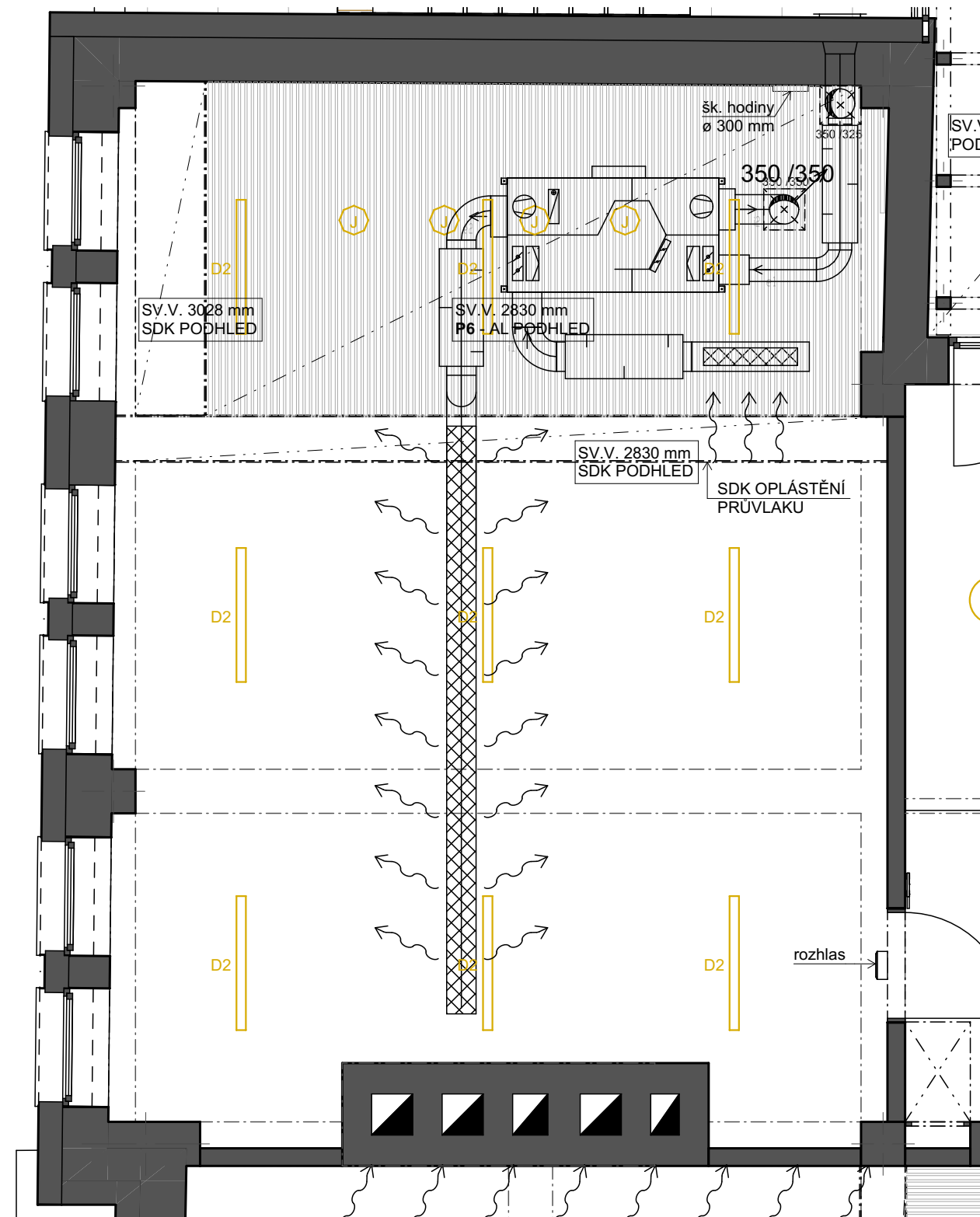
PŮDORYS PODHLEDU
