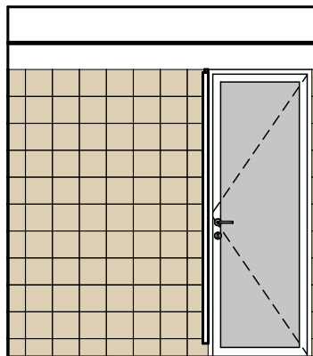
POHLED 2.10_02
