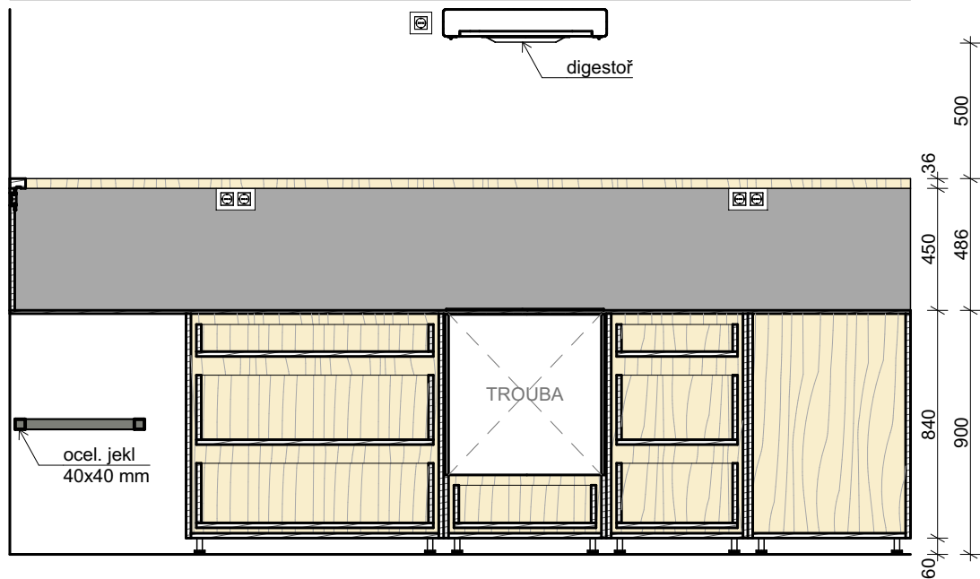
řez podélný 01 M 1:25
