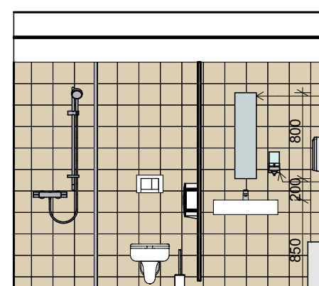
POHLED 2.08_04
