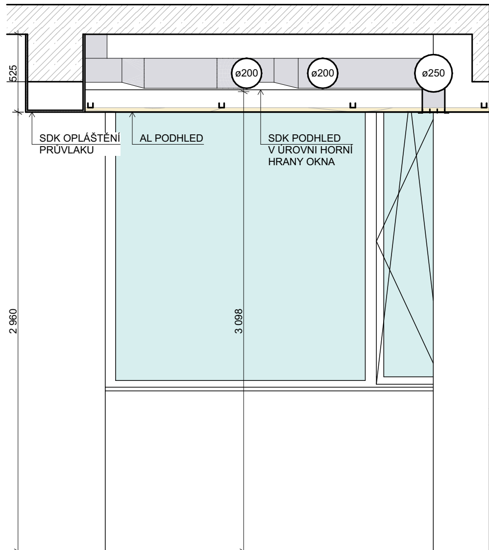
PODÉLNÝ ŘEZ - DETAIL PODHLEDU
