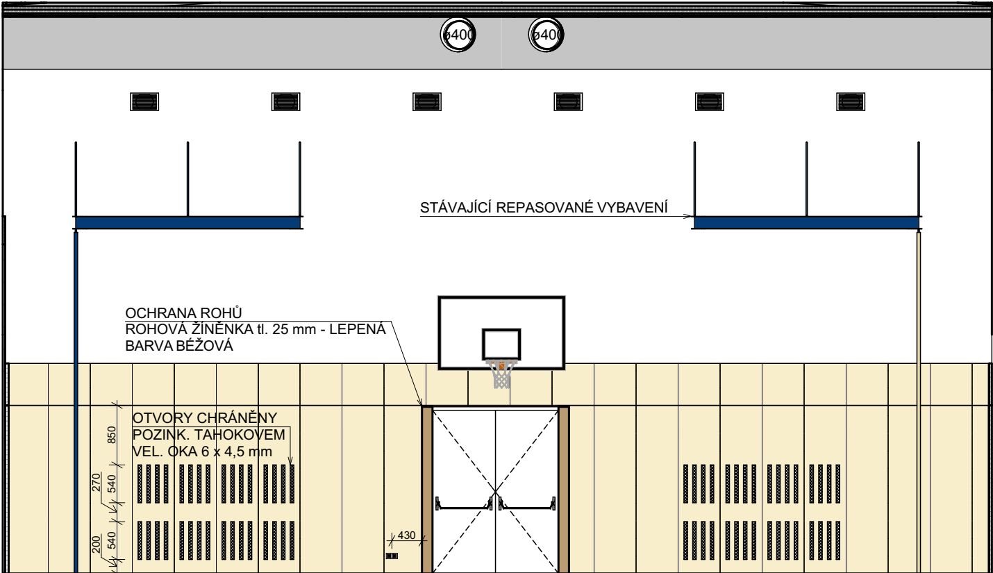
POHLED 1.24_02
