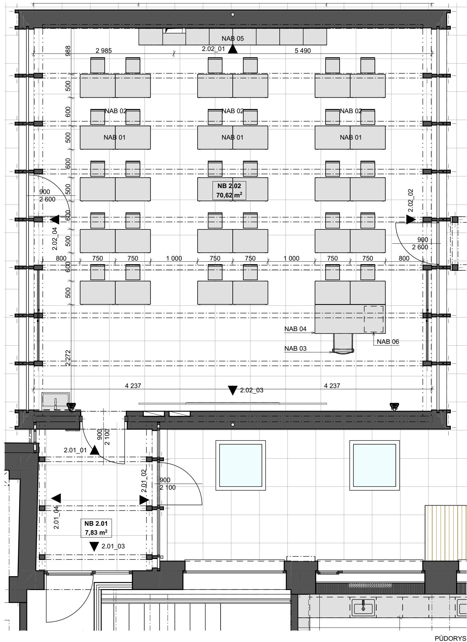
PŮDORYS
