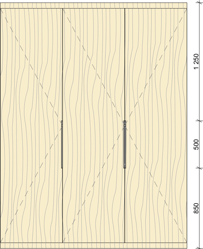
pohled_01 M 1:25
