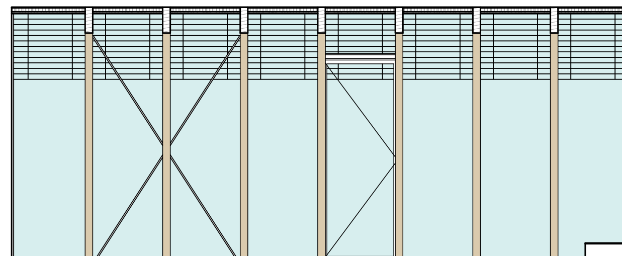
POHLED 2.04_04
