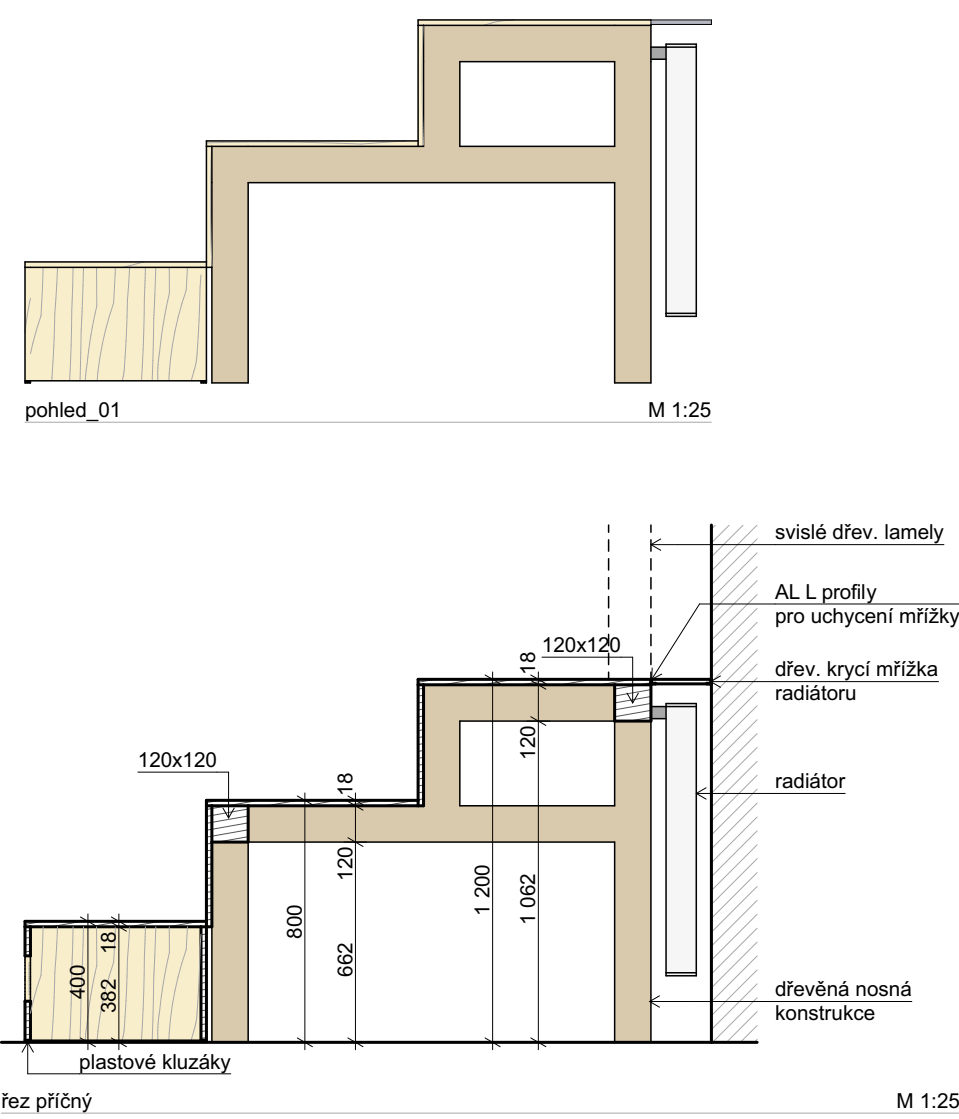
řez příčný
