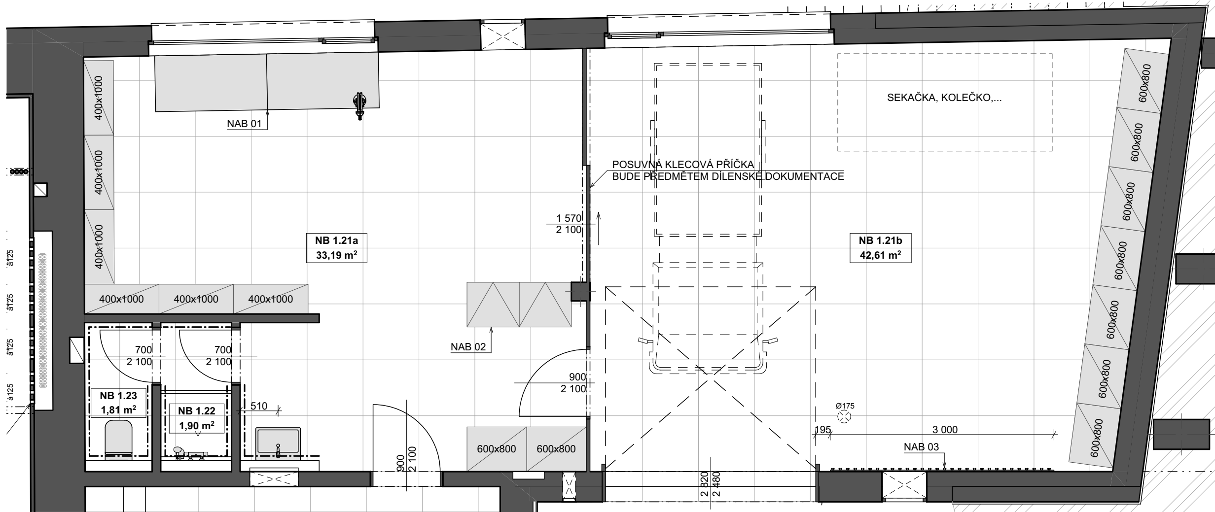
PŮDORYS
