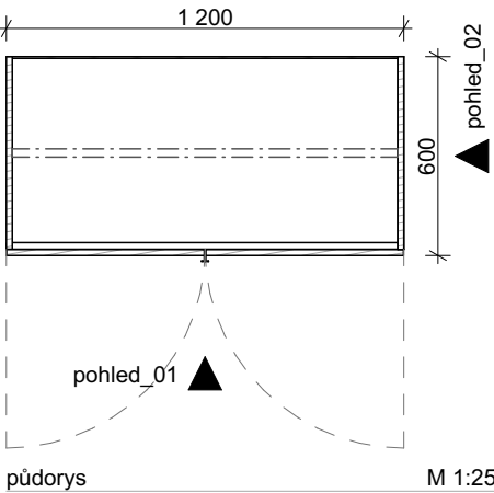
půdorys M 1:25
