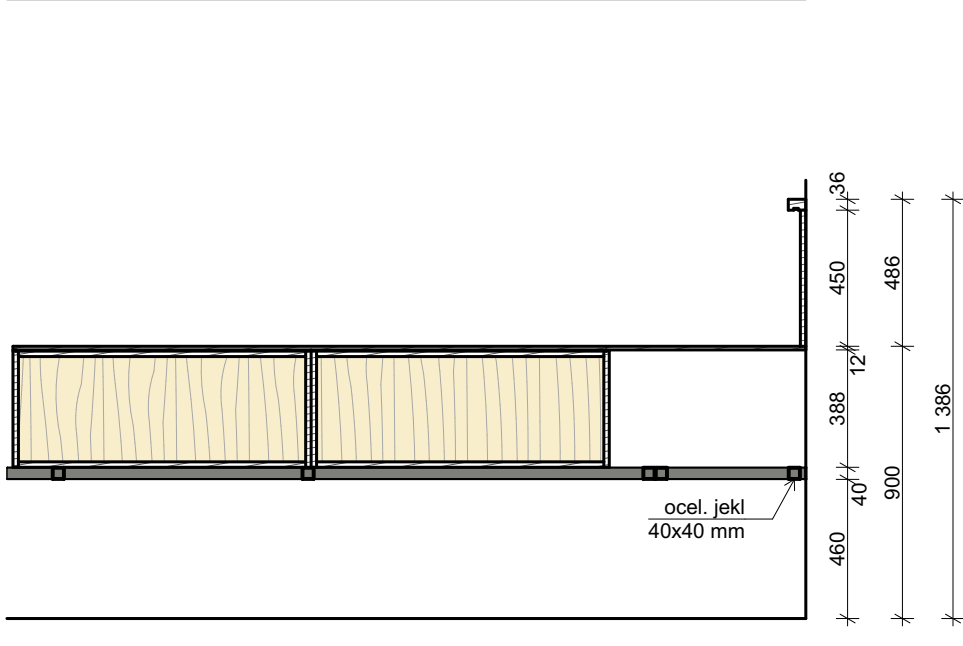
řez podélný 02 M 1:25
