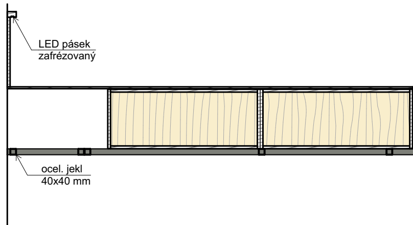
řez podélný 01 M 1:25
