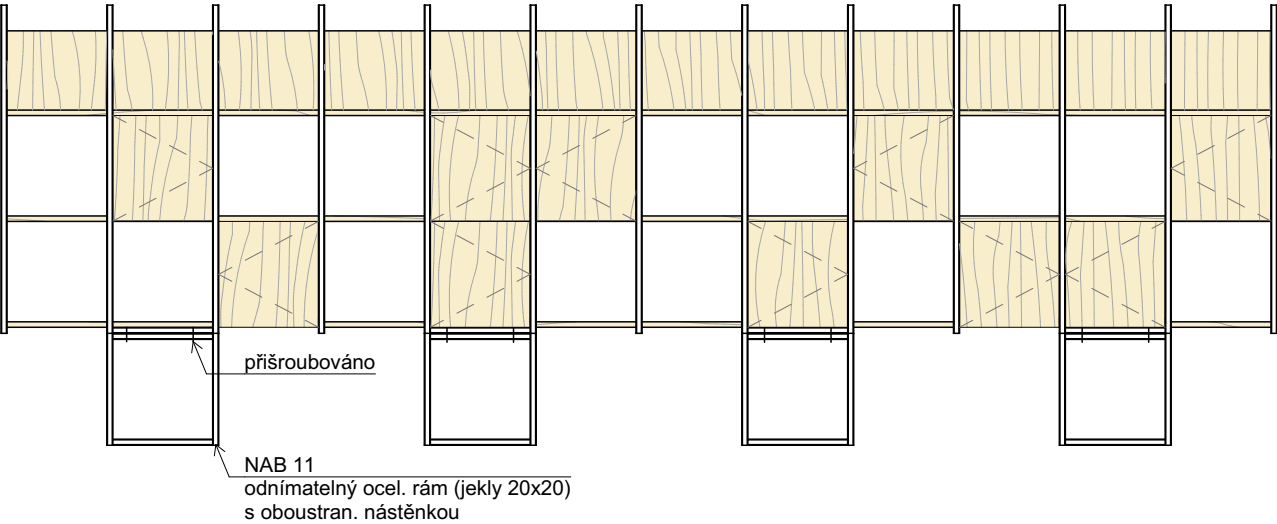
pohled_02 M 1:25
