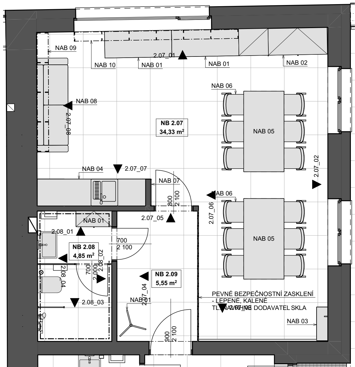
PŮDORYS
