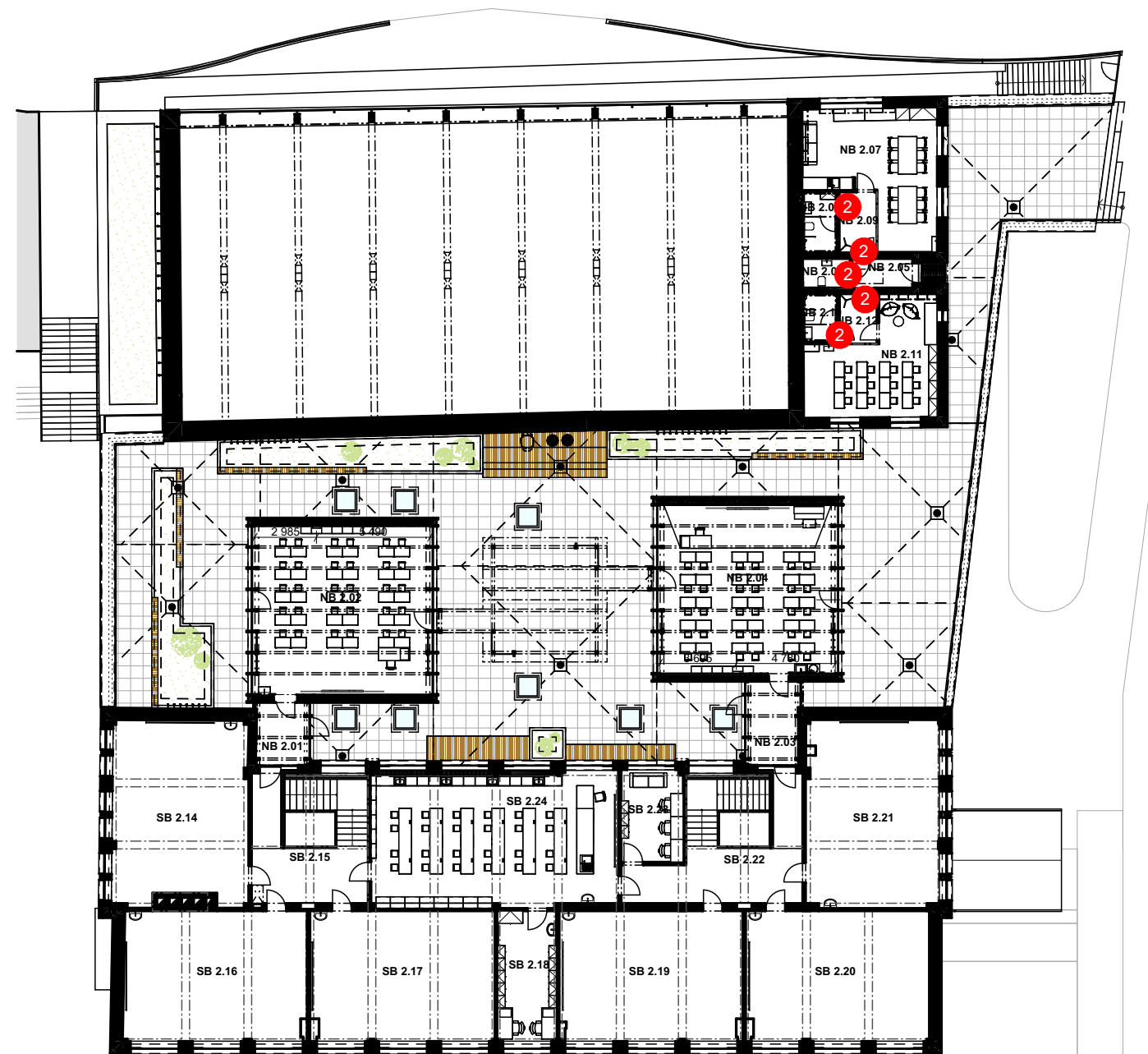
PŮDORYS 2.NP
