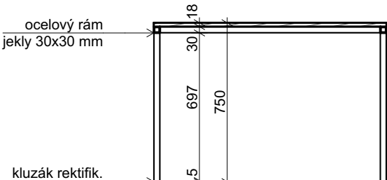
řez podélný M 1:25
