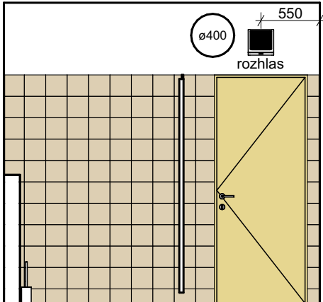
POHLED WC 1.05_05
