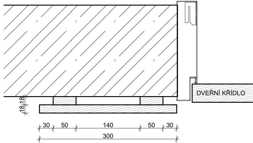
Půdorys M 1:5
