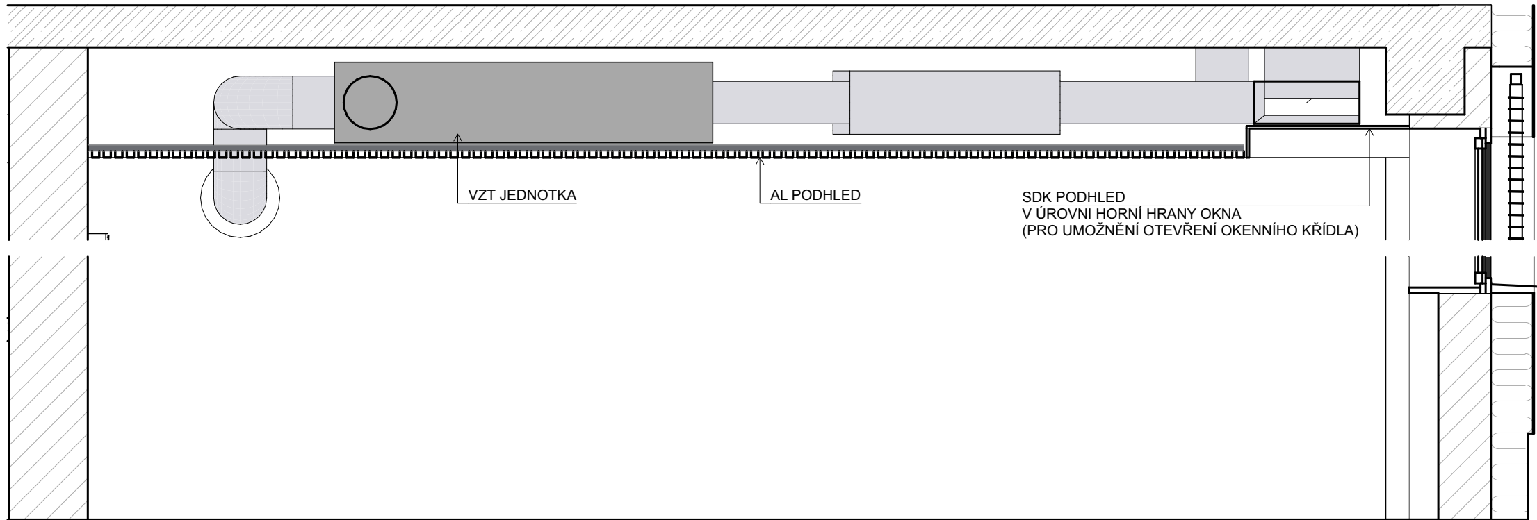
PODÉLNÝ ŘEZ - DETAIL PODHLEDU
