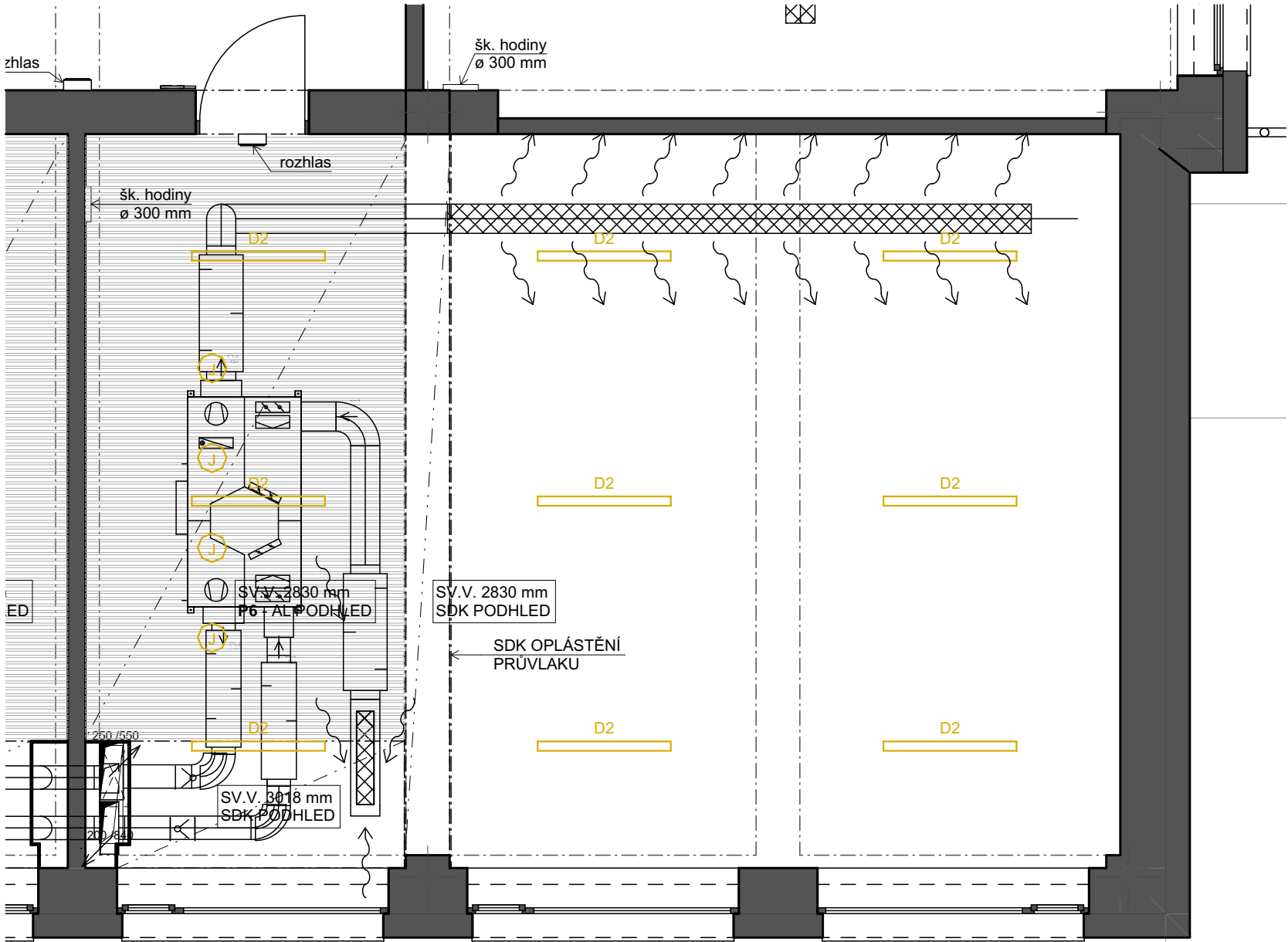
PŮDORYS PODHLEDU
