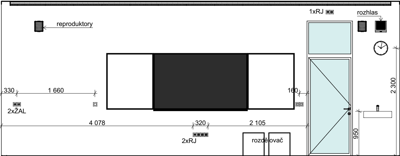
POHLED 2.02_03
