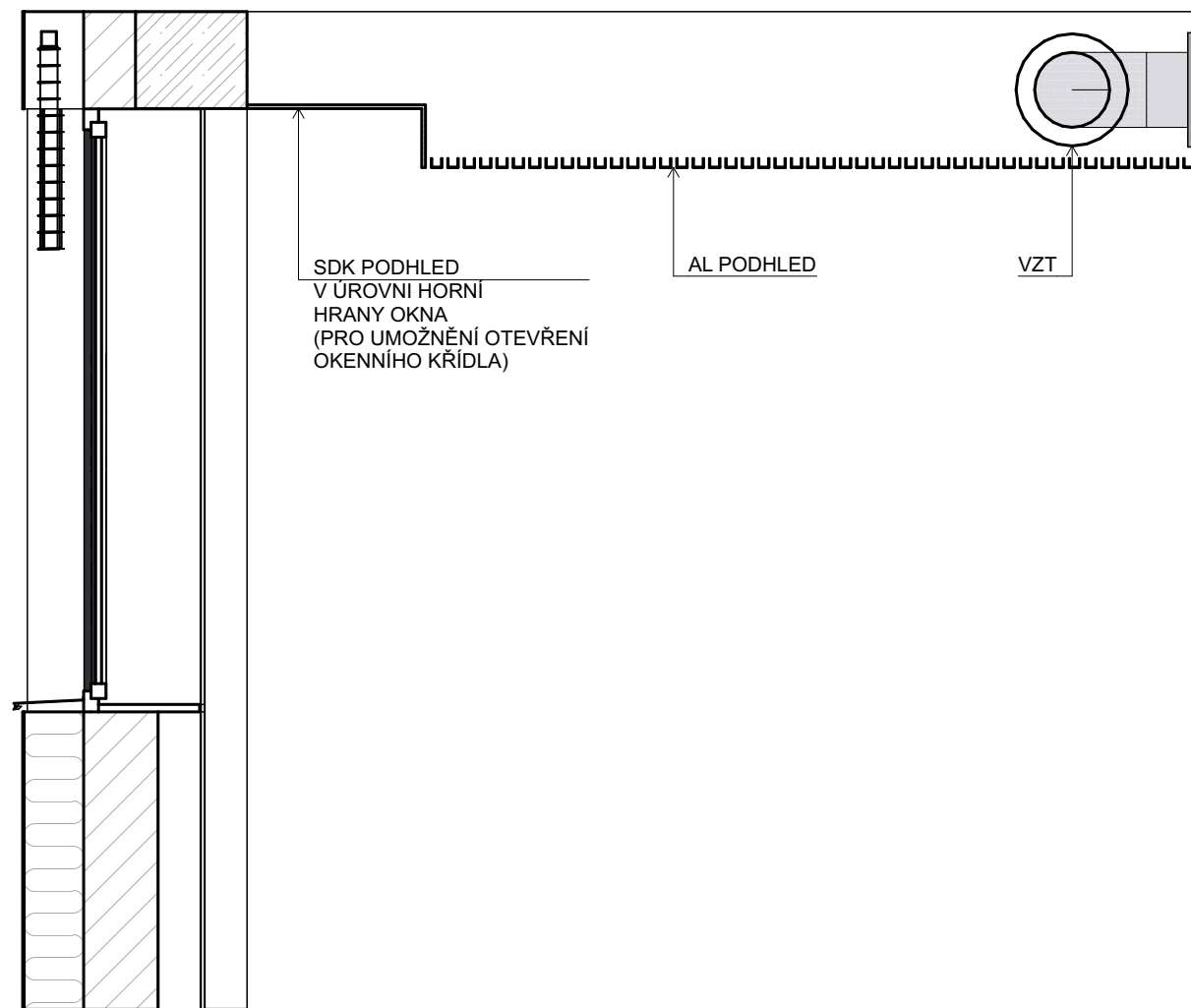
PŘÍČNÝ ŘEZ - DETAIL PODHLEDU
