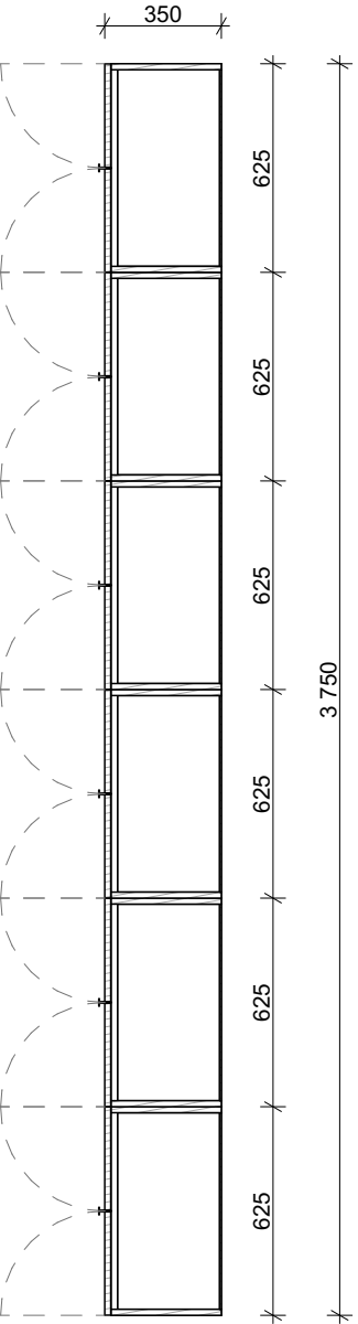
pohled_02 půdorys horních skříněk M 1:25
