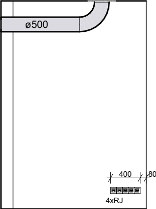
POHLED 1.25_04
