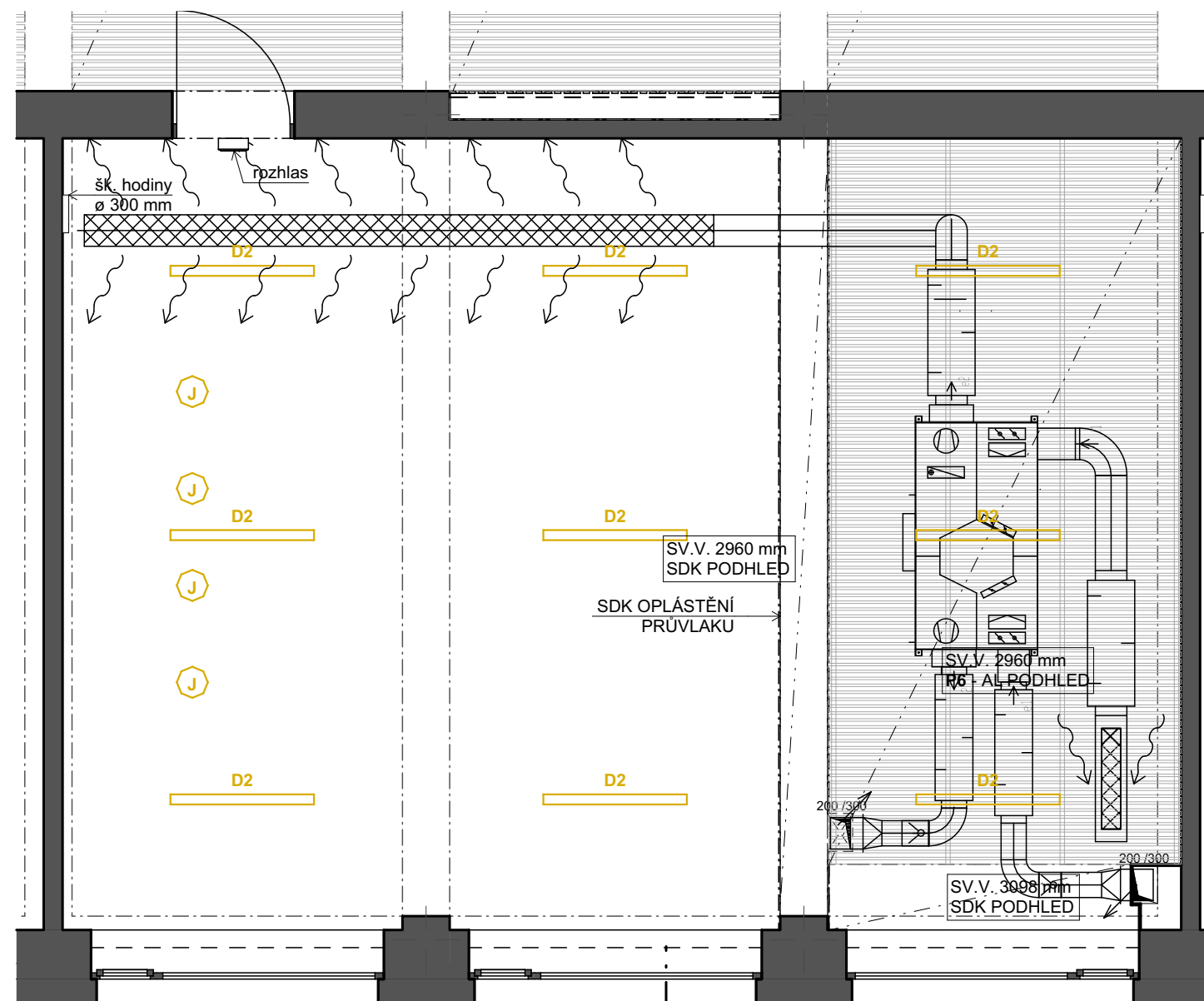
PŮDORYS PODHLEDU
