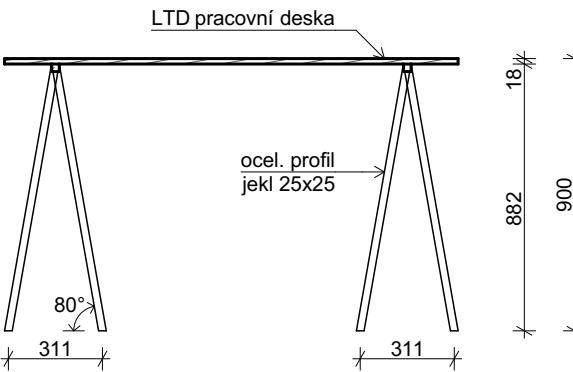
řez podélný M 1:25
