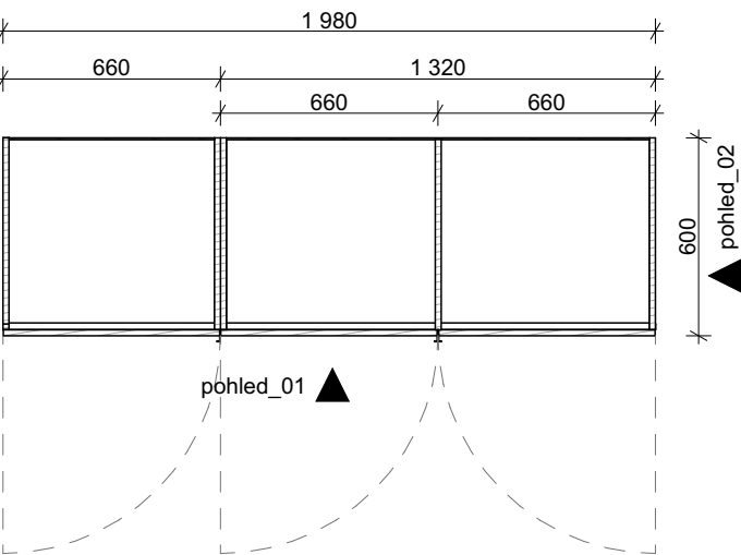
půdorys M 1:25
