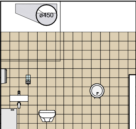
POHLED WC 1.05_07
