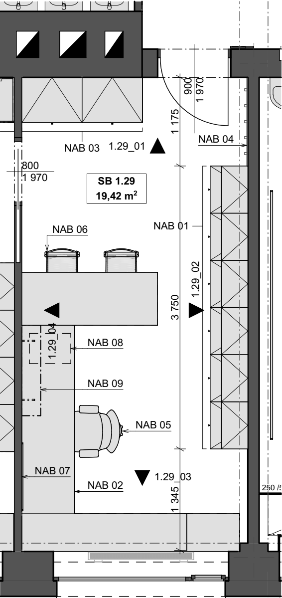
PŮDORYS
