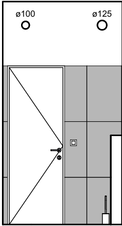
POHLED 1.13_05
