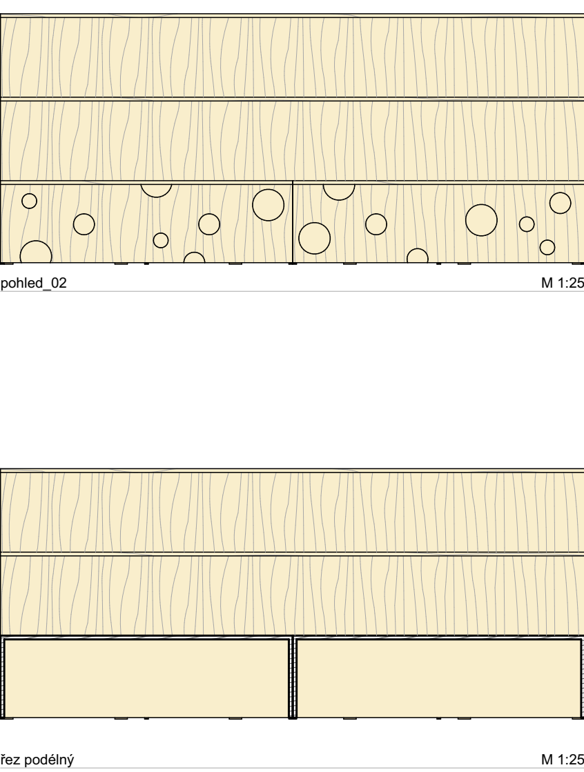
řez podélný
