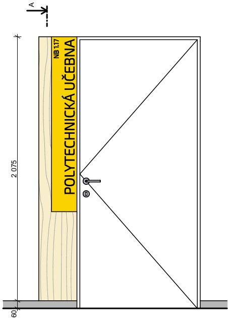
Pohled M 1:30
