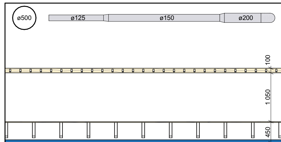
POHLED 1.09_01
