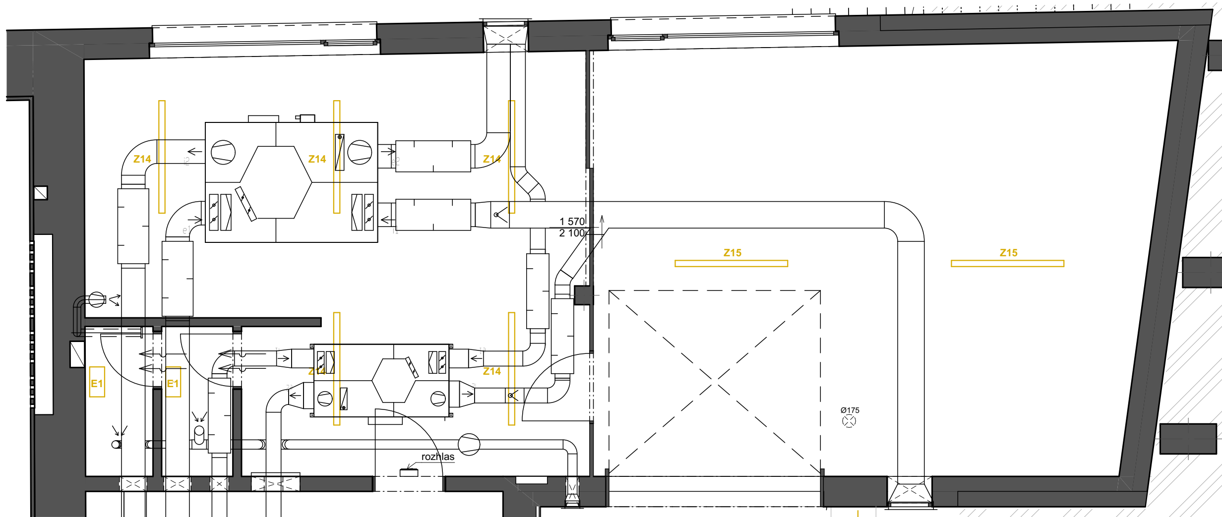
PŮDORYS PODHLEDU
