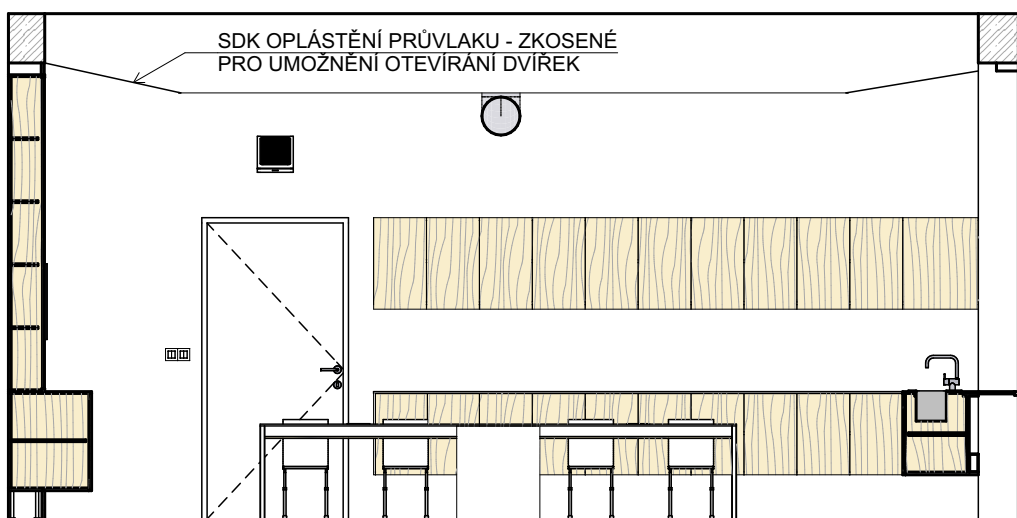
POHLED 2.24_05
