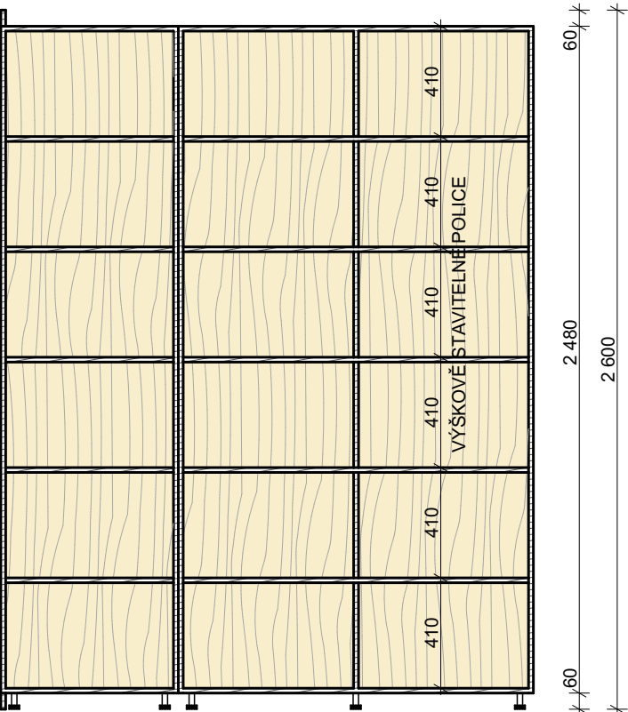
řez podélný M 1:25
