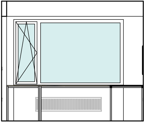
POHLED 1.29_03
