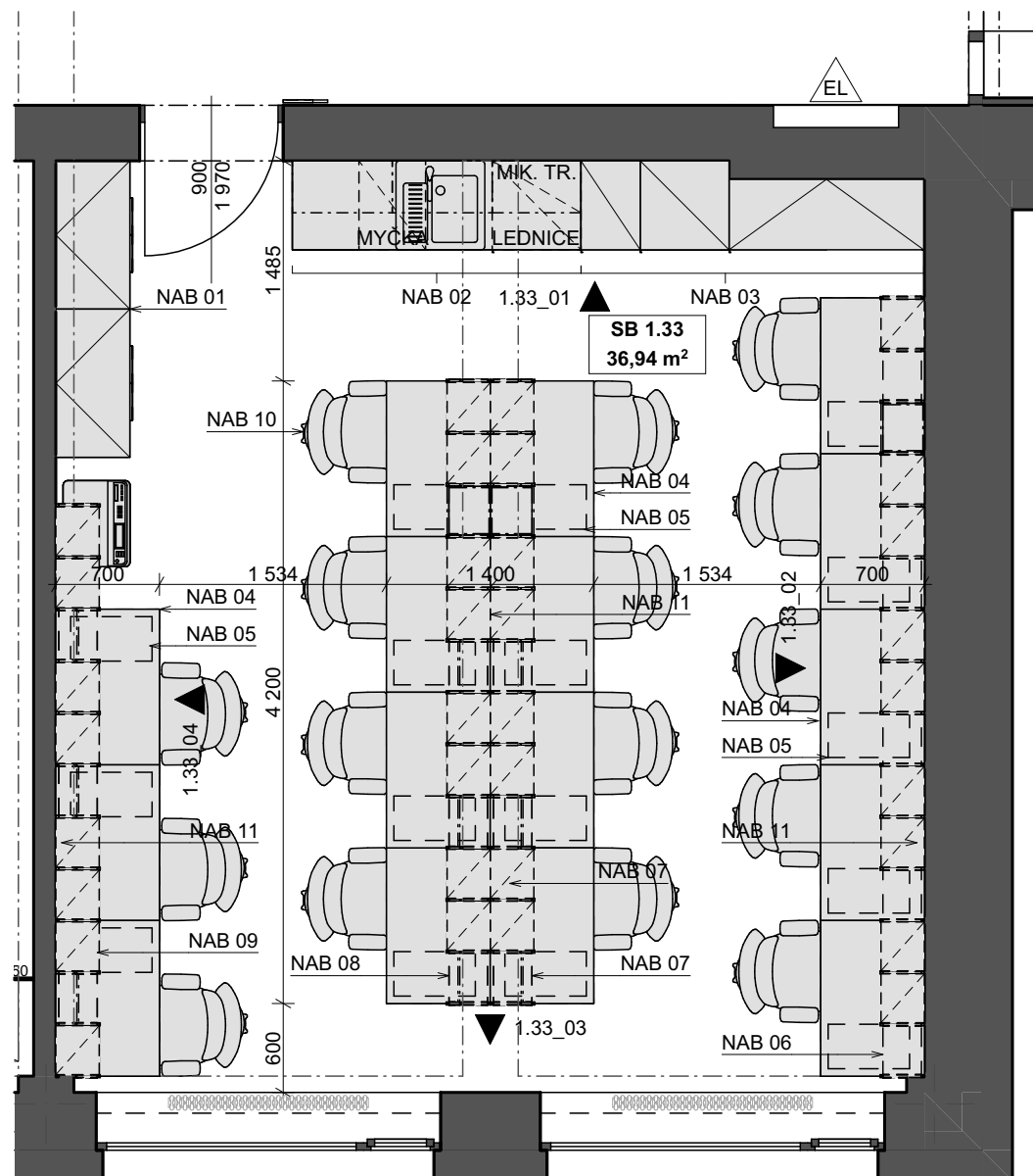
PŮDORYS
