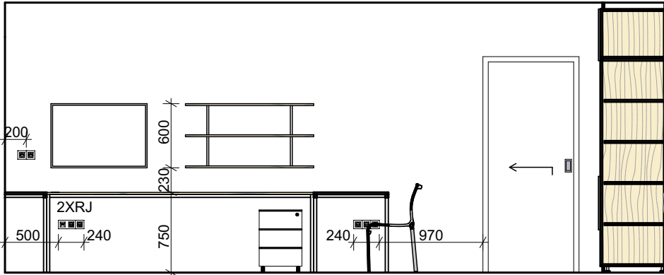
POHLED 1.29_04
