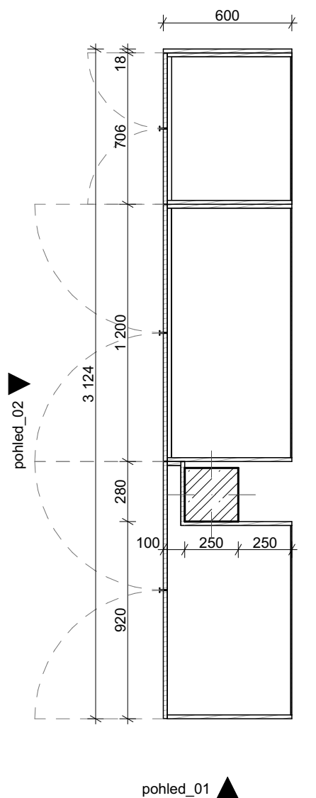
pudorys
