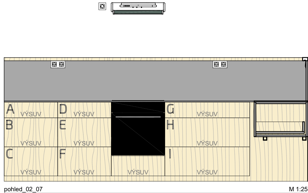
pohled_02_07 M 1:25
