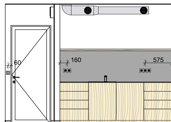
POHLED 2.07_07
