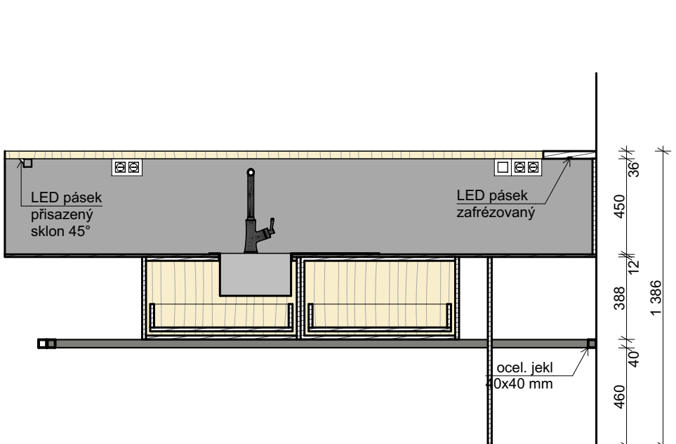
řez příčný M 1:25
