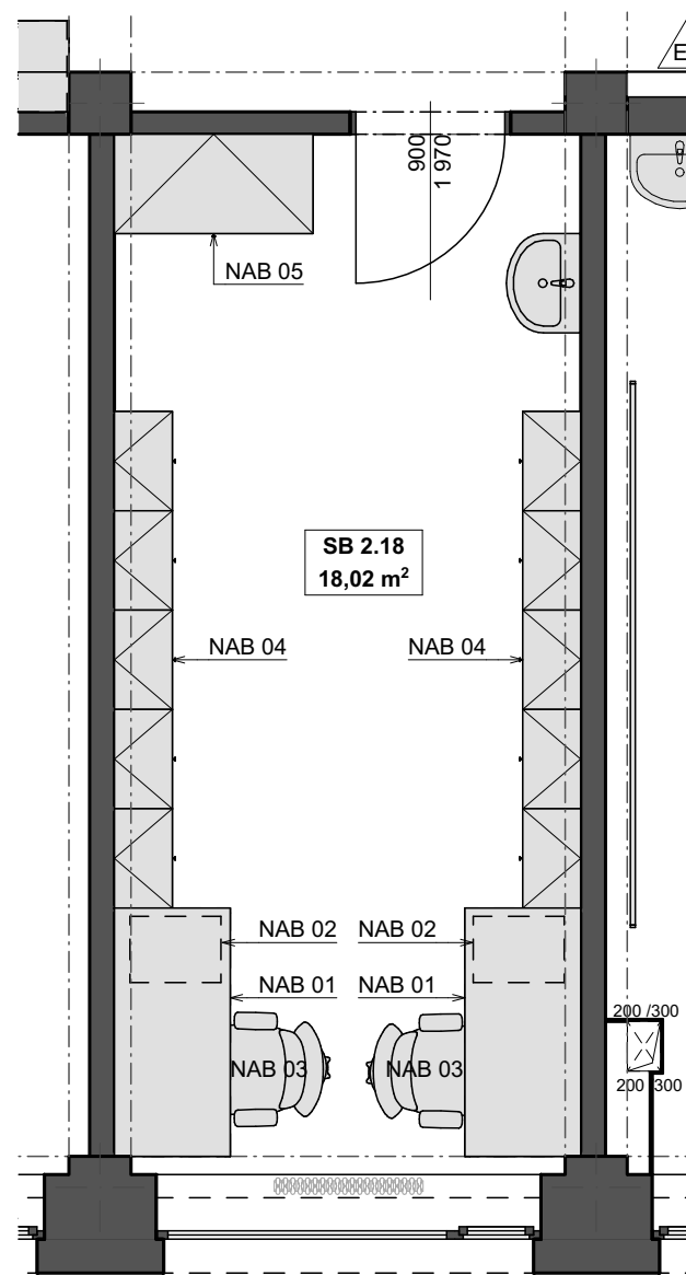
PŮDORYS
