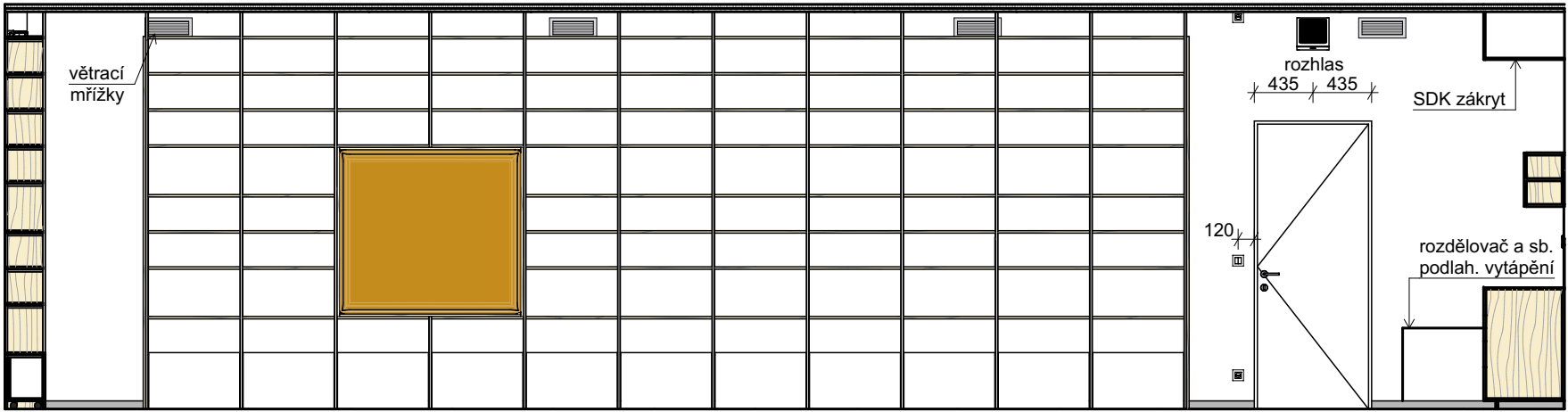
POHLED 1.12_01
