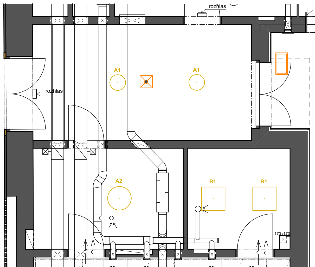
PŮDORYS PODHLEDU
