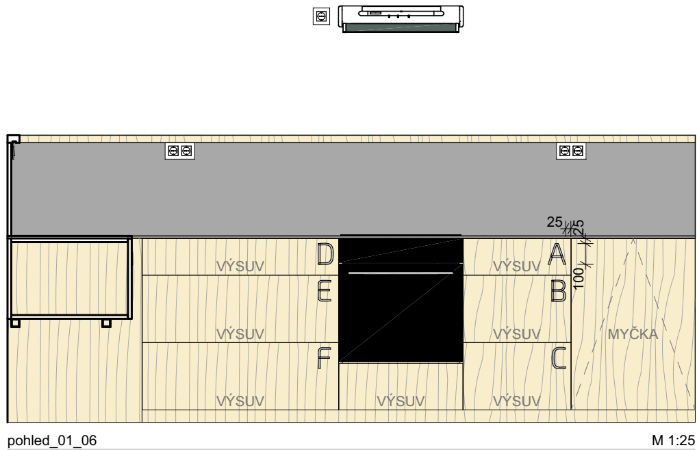
pohled_01_06 M 1:25
