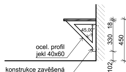
řez příčný M 1:25
