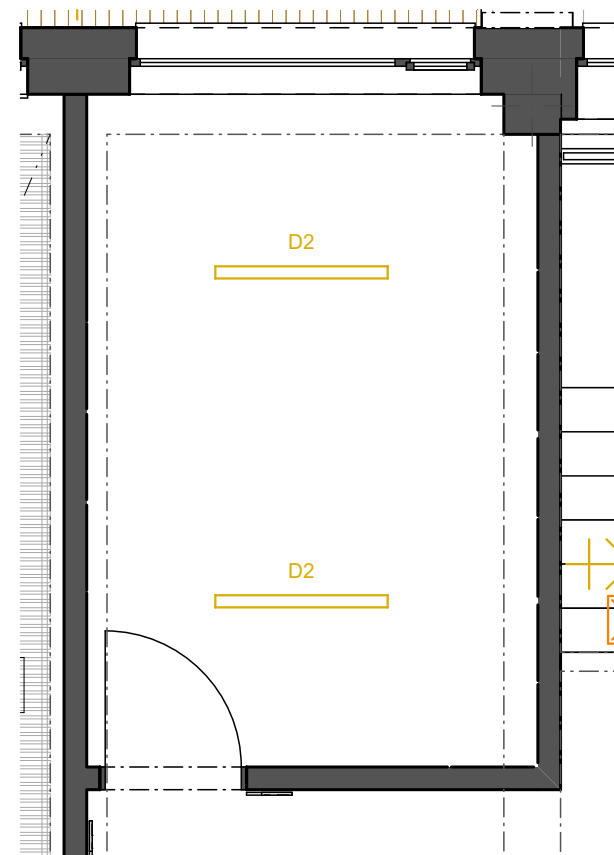
PŮDORYS PODHLEDU
