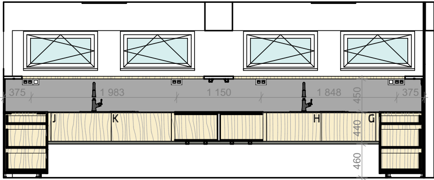
POHLED 01.06_03
