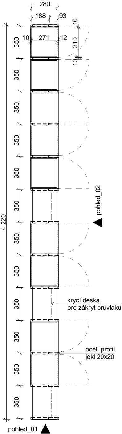
půdorys M 1:25
