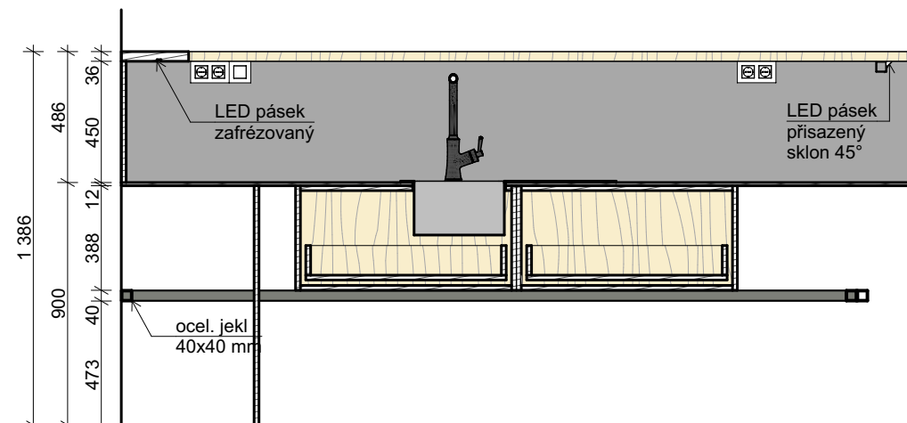
řez příčný M 1:25
