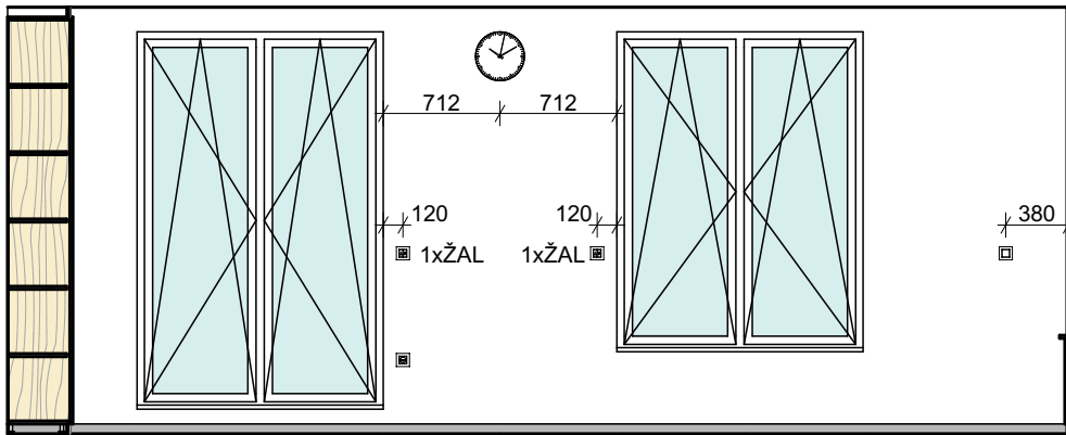
POHLED 2.11_03
