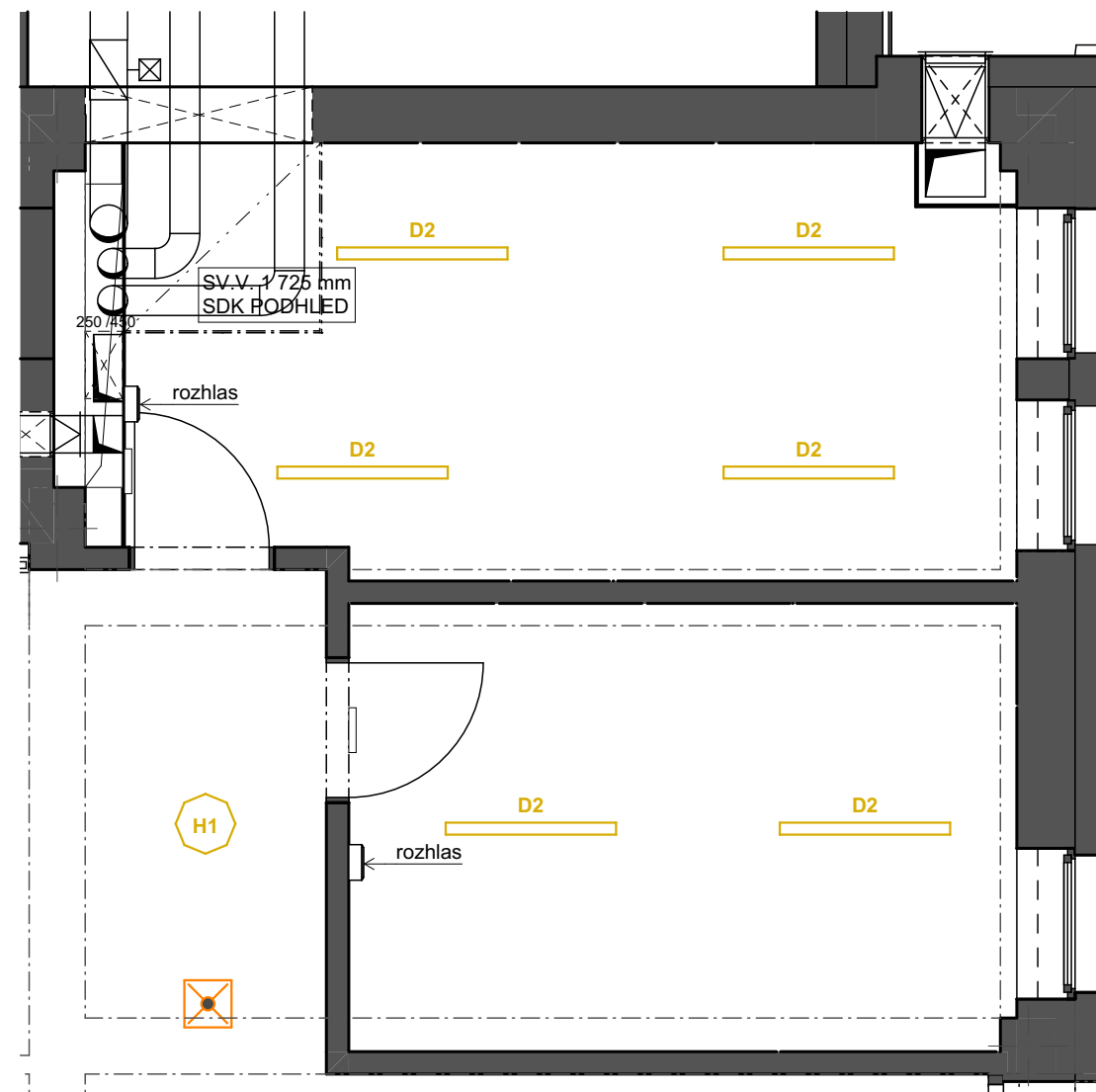
PŮDORYS PODHLEDU
