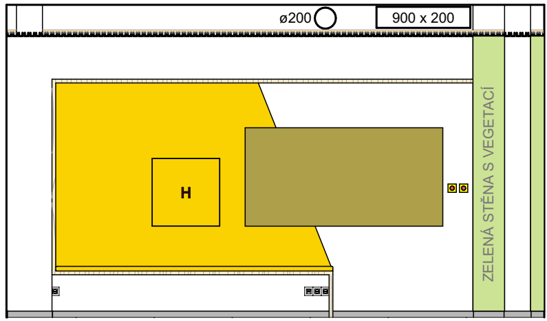
POHLED 1.01_03
