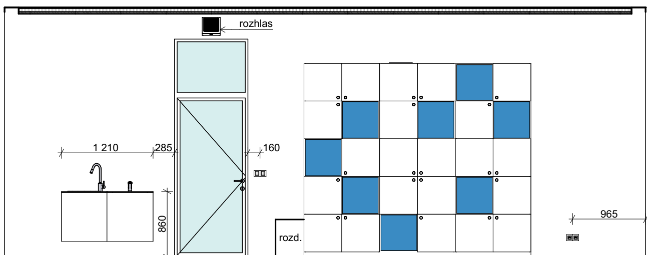
POHLED 2.04_03
