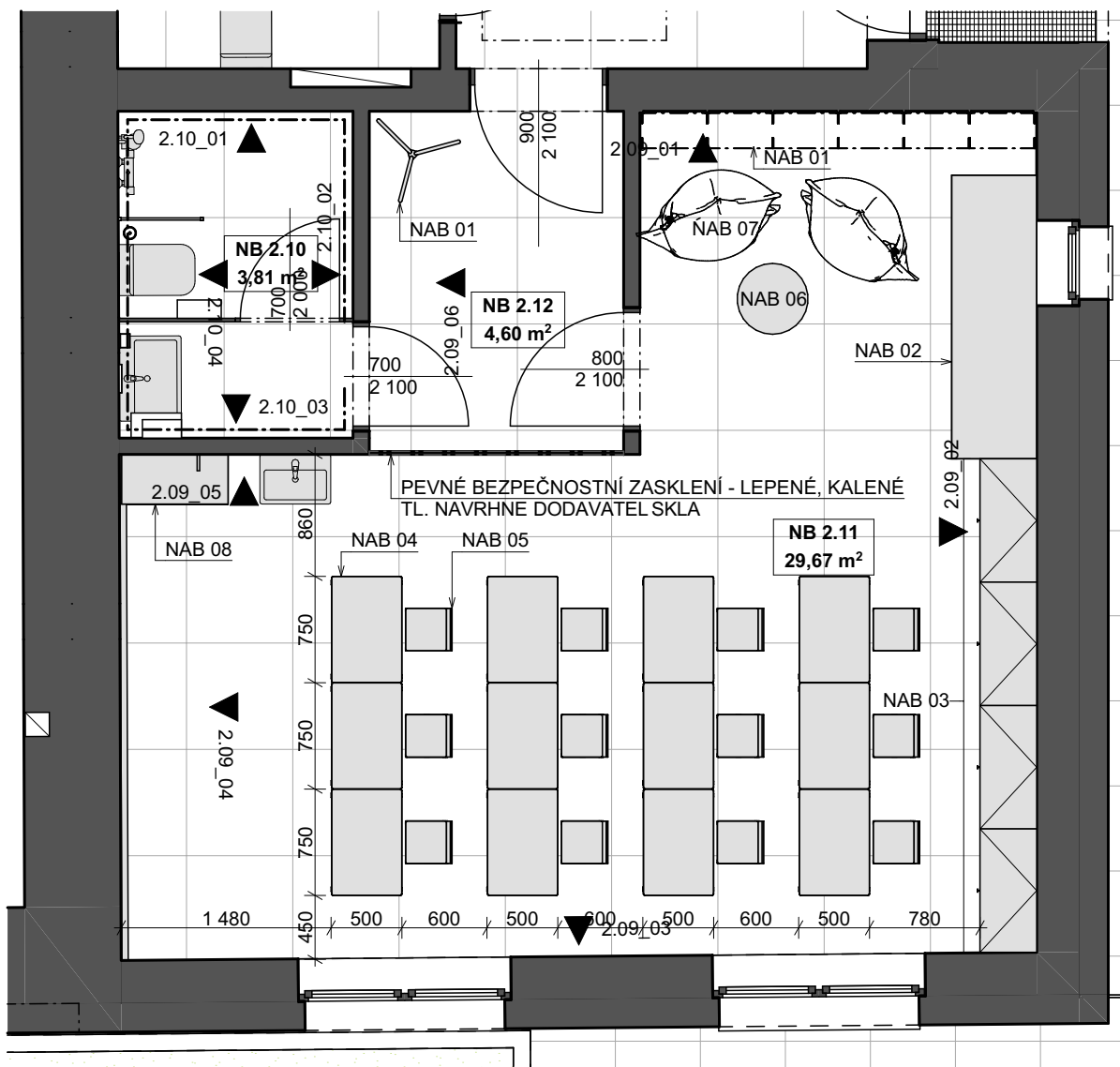
PŮDORYS
