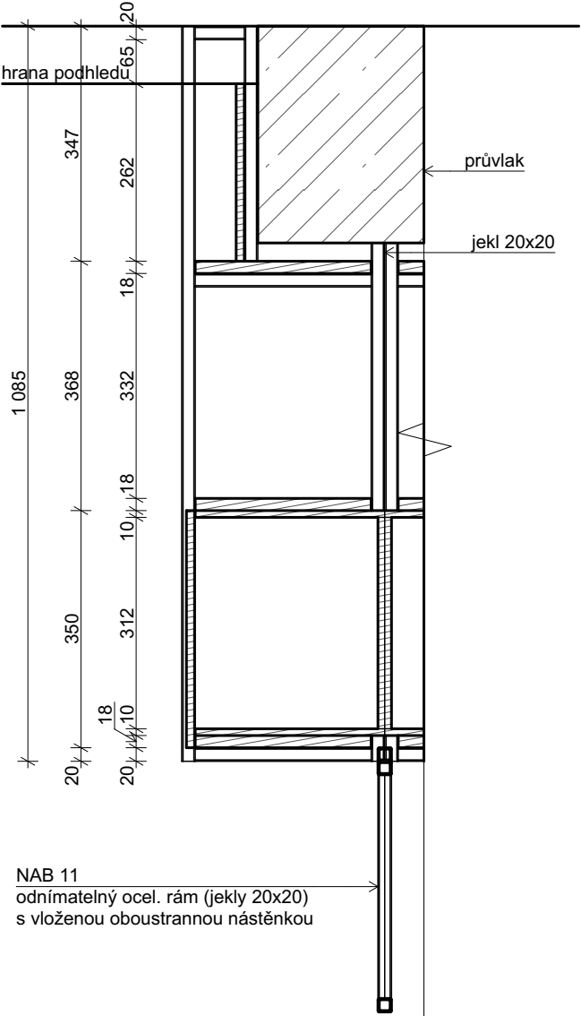
řez příčný M 1:10
