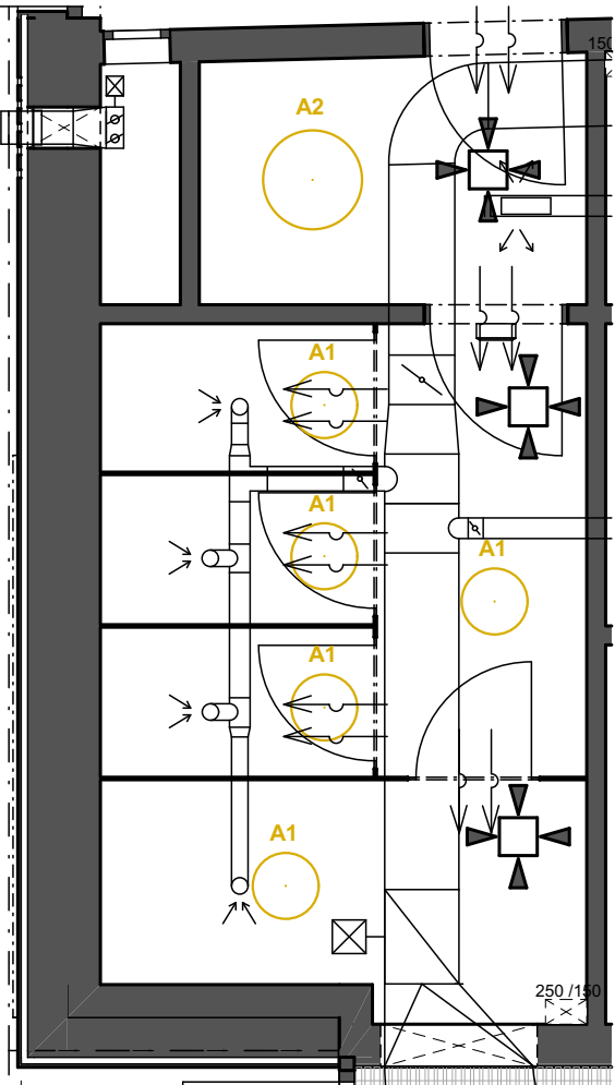
PŮDORYS PODHLEDU
