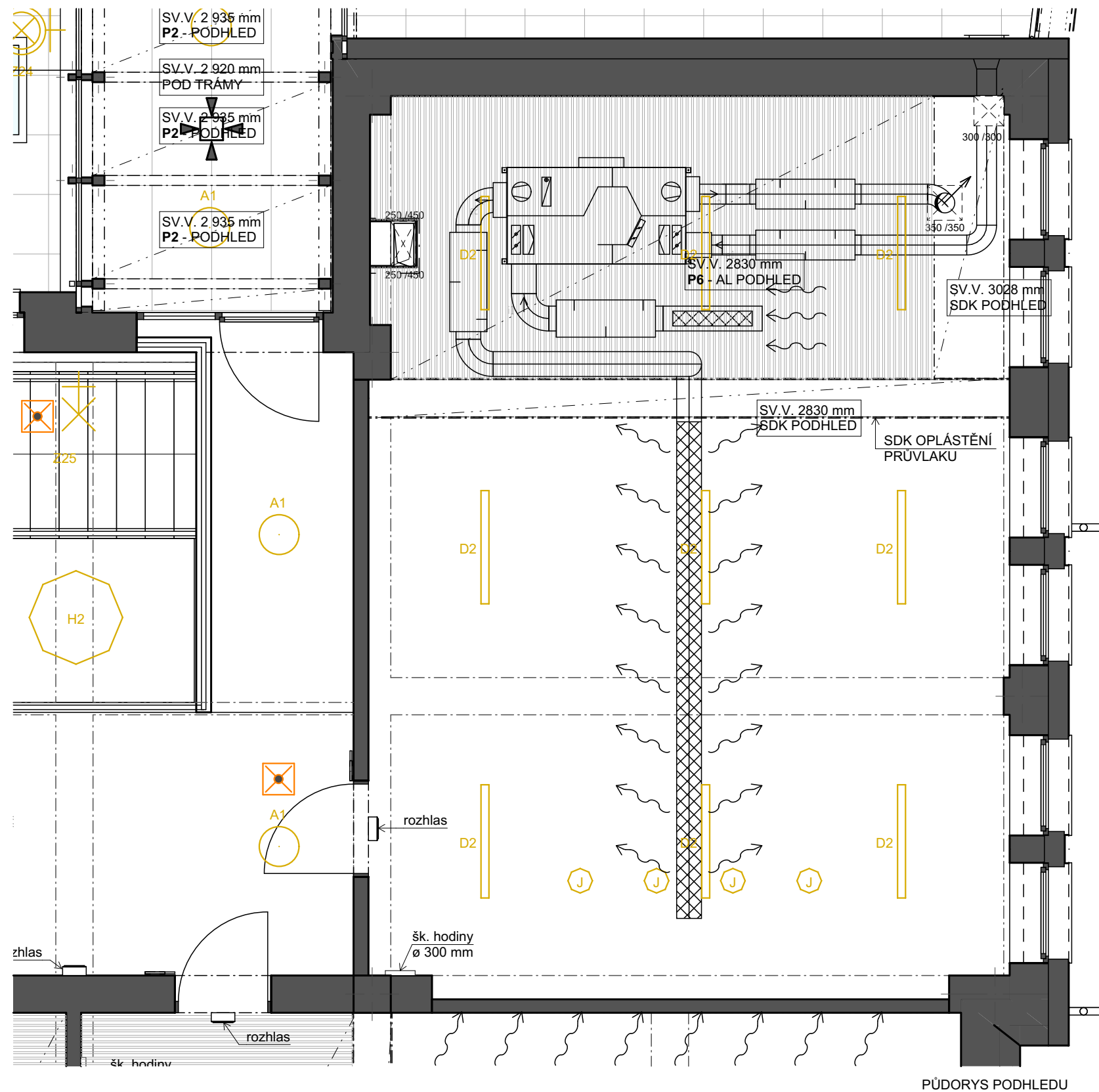
DETAIL PODHLEDU - VIZ UČEBNA 2.14
