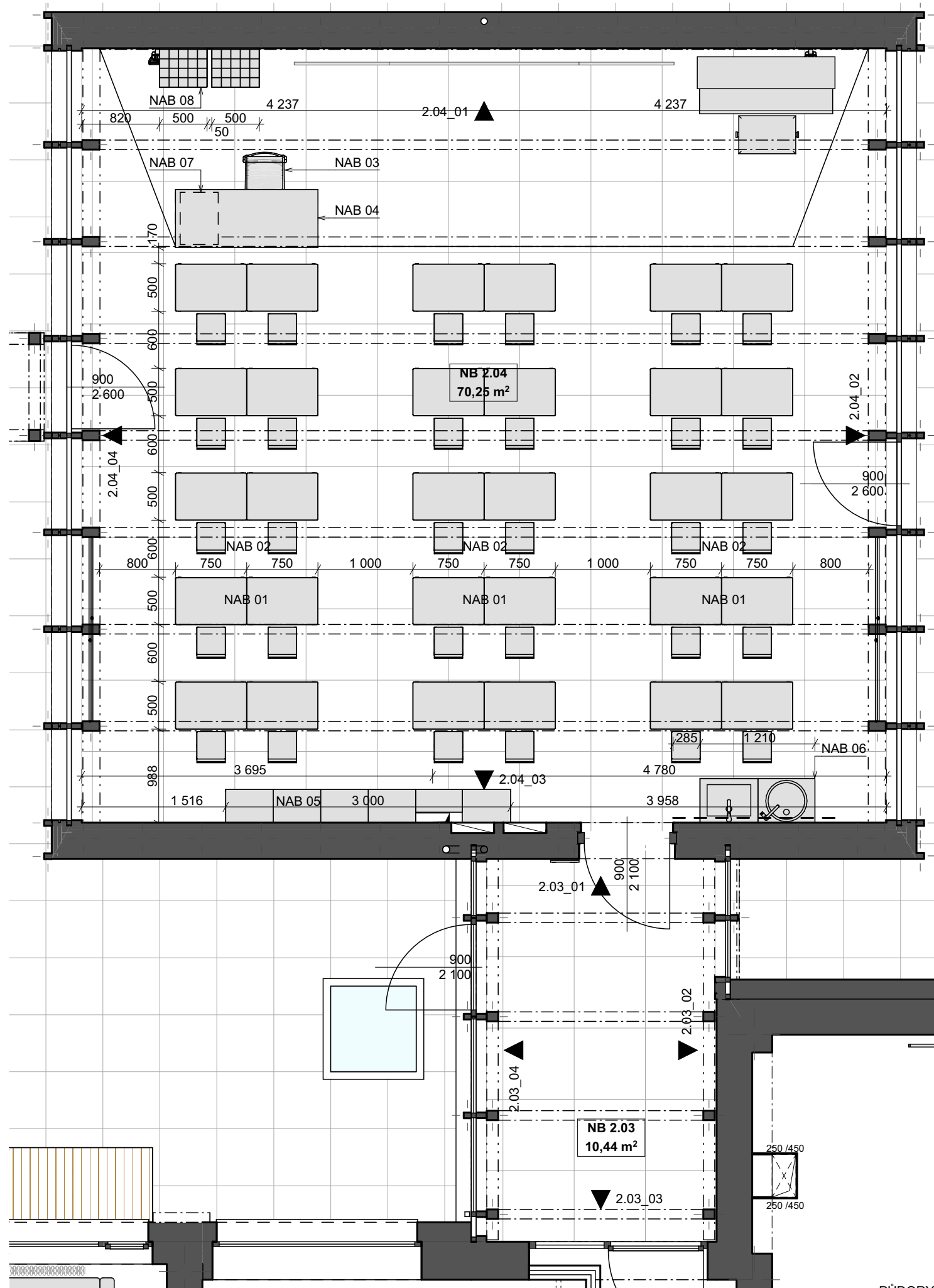
PŮDORYS
