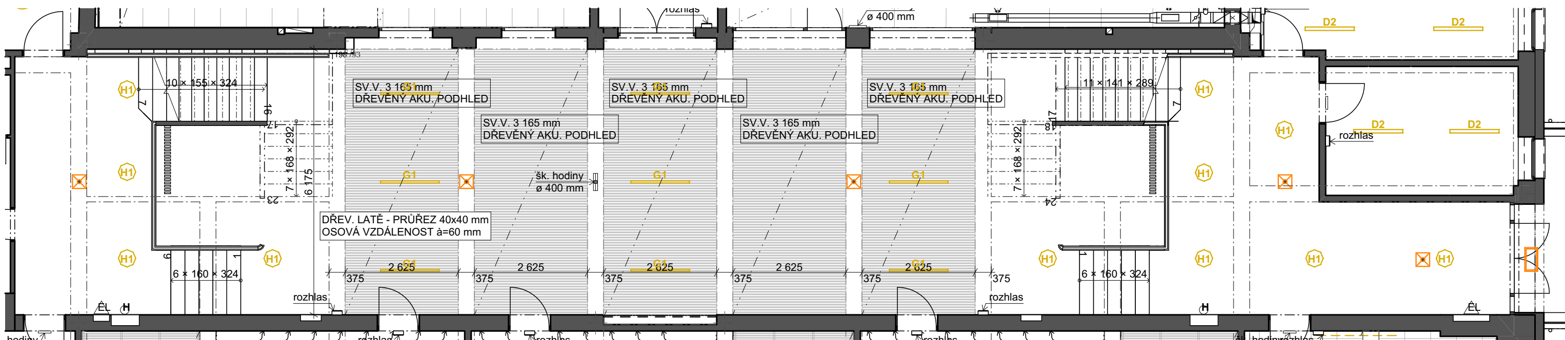
PŮDORYS PODHLEDU
