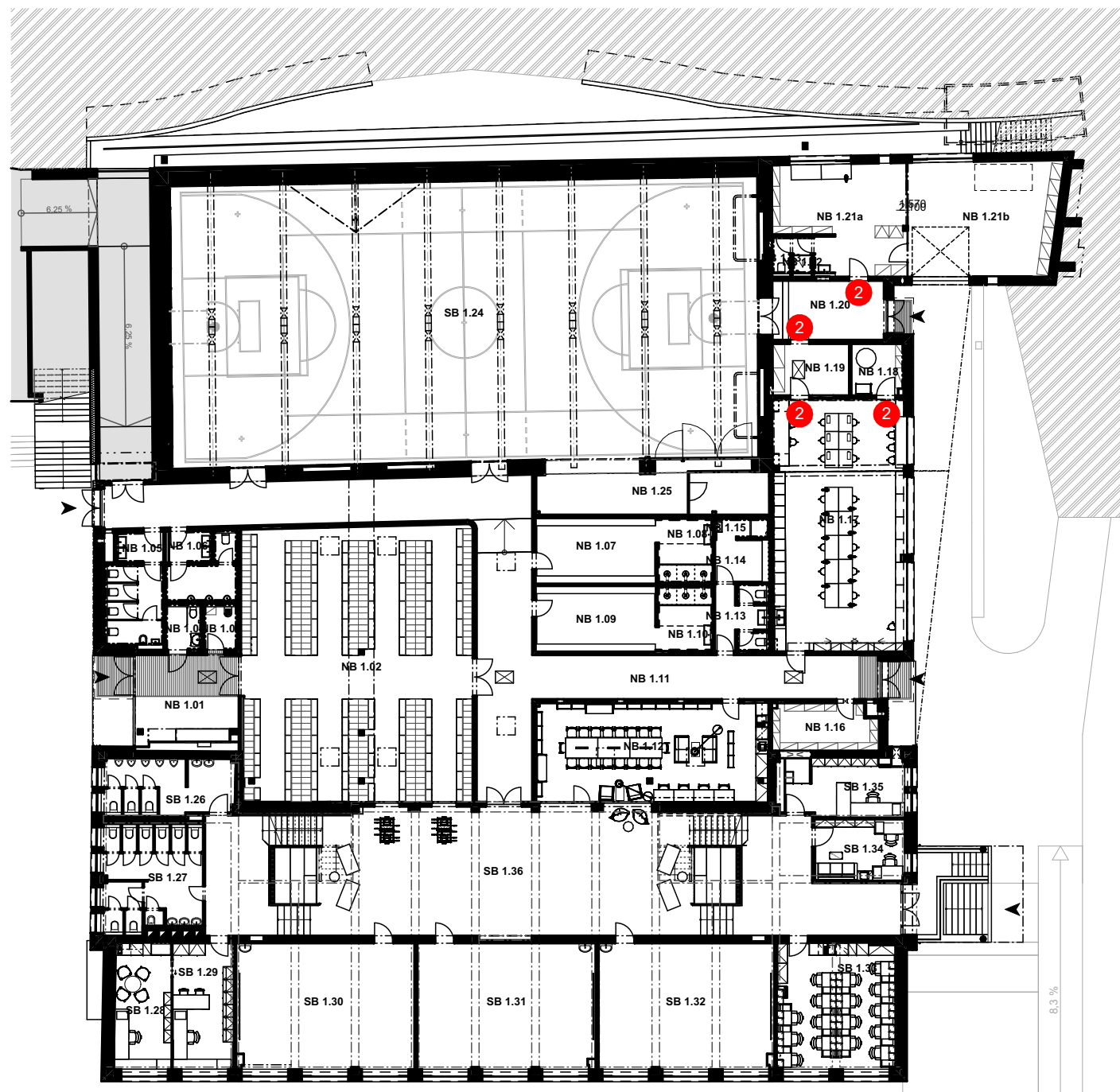
PŮDORYS 1.NP
