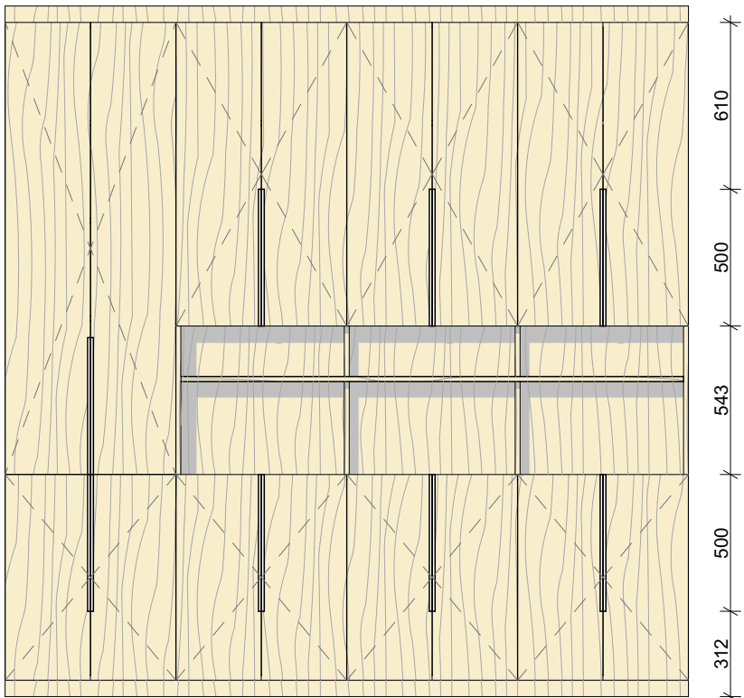
pohled_02 M 1:25
