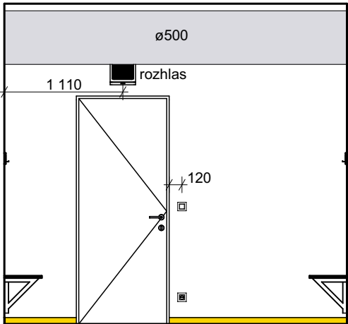
POHLED 1.07_07
