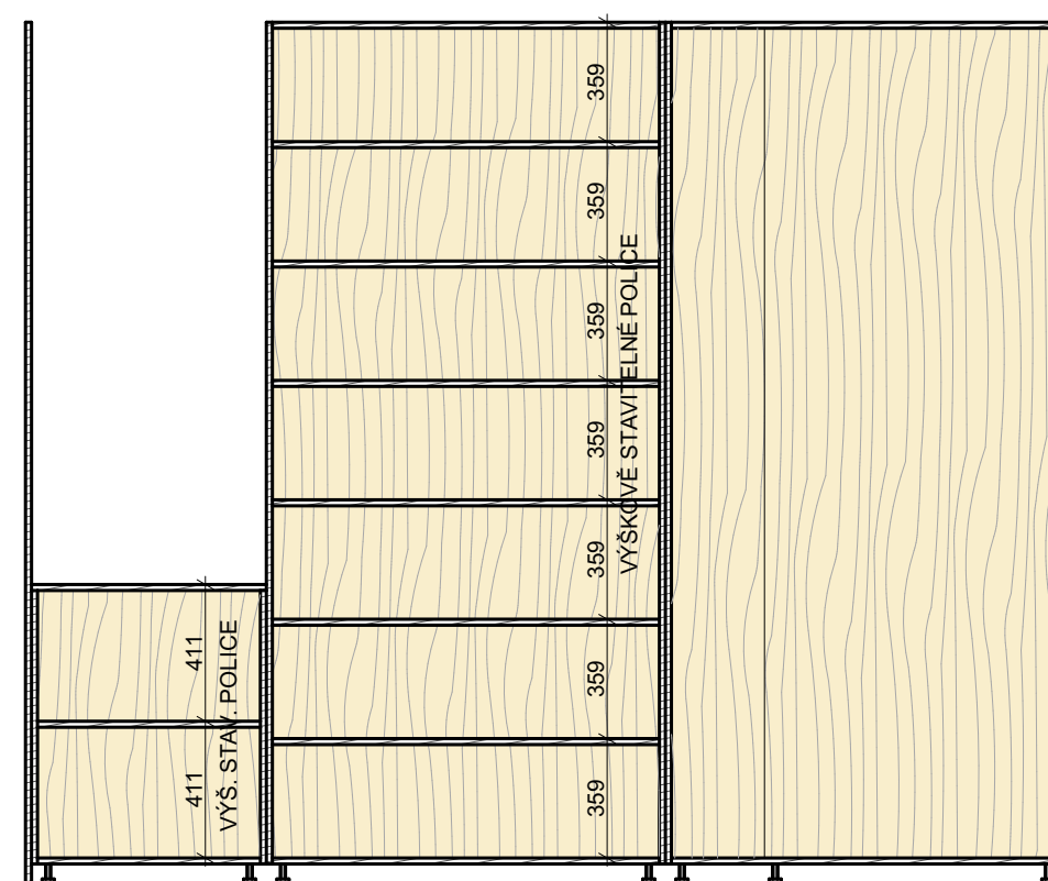
řez podélný
