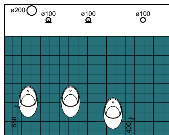
POHLED WC 1.06_07
