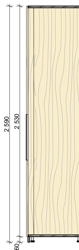
řez příčný
