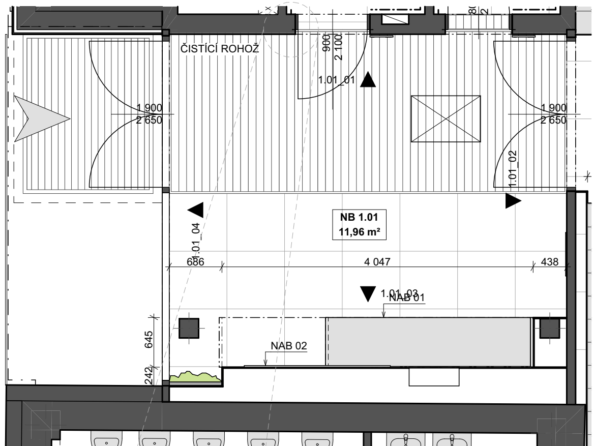
PŮDORYS
