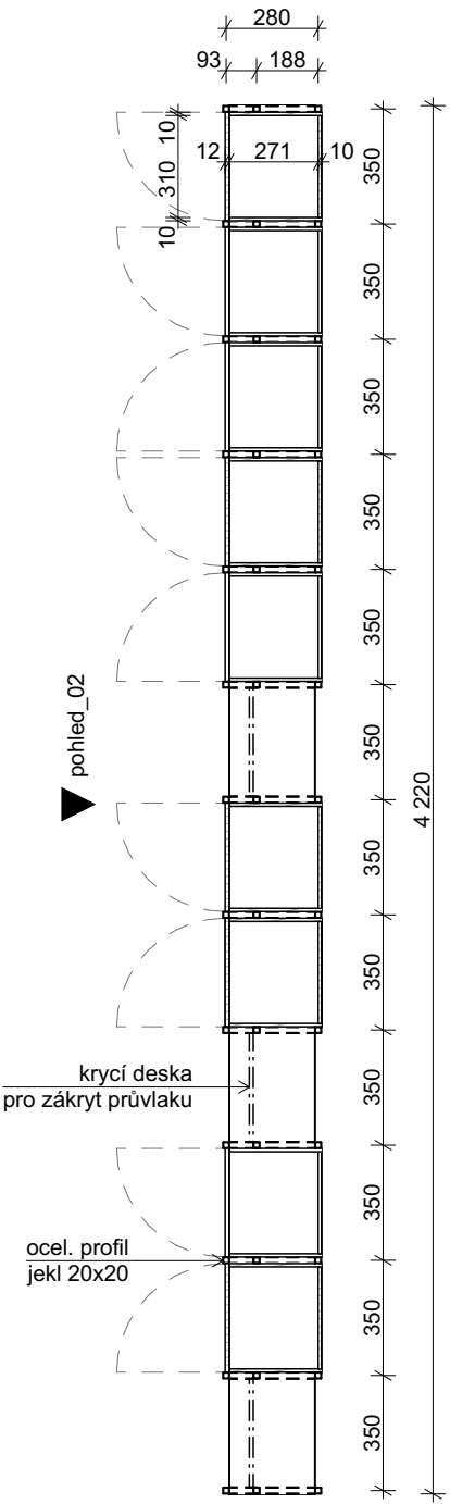
pohled_01 M 1:25
