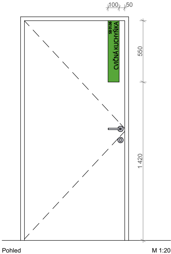
Pohled M 1:20
