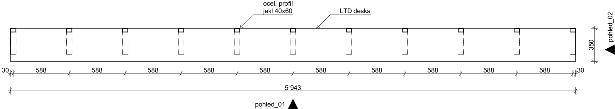
půdorys M 1:25
