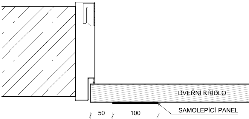
Půdorys M 1:5
