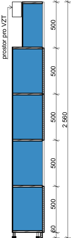
řez příčný
