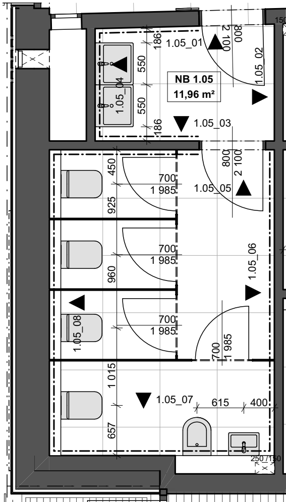
PŮDORYS
