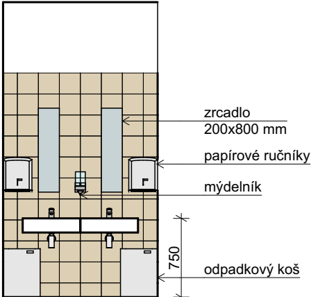
POHLED PŘEDSÍŇ 1.05_04
