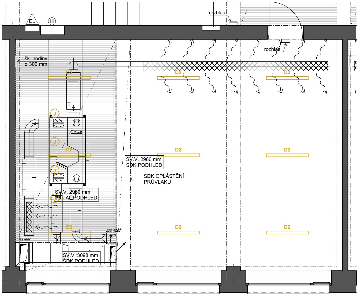
PŮDORYS PODHLEDU
