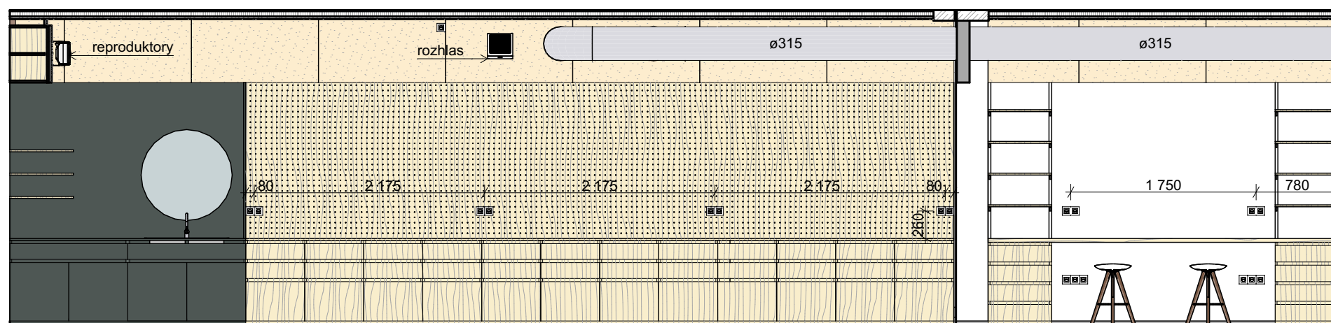
POHLED 1.17_04
