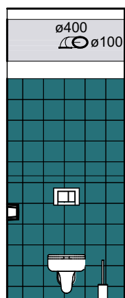
POHLED KABINA 1.06_09
