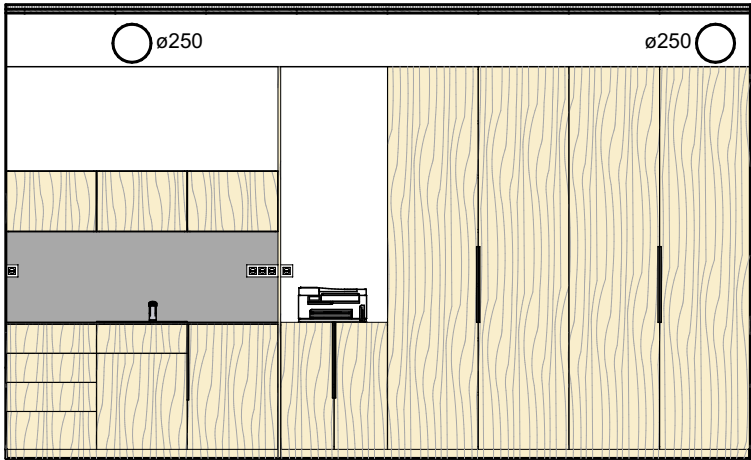
POHLED 1.12_02
