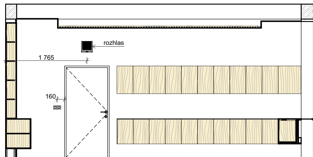
POHLED 2.24_04
