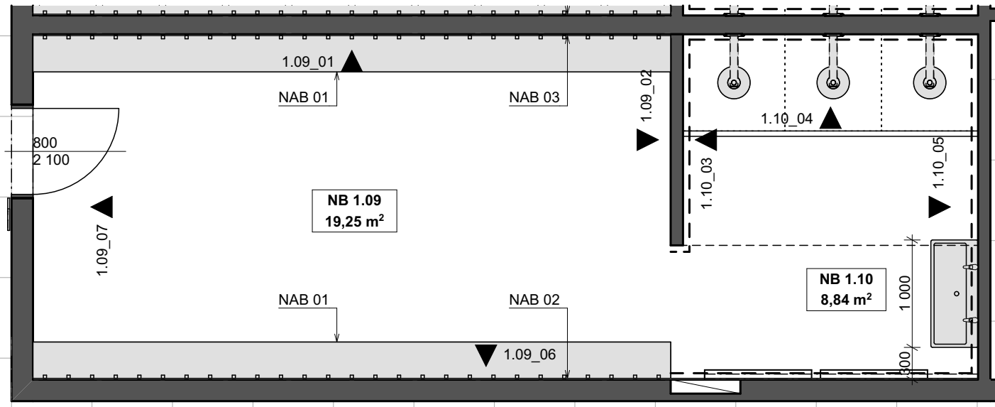
PŮDORYS
