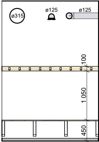
POHLED 1.14_02
