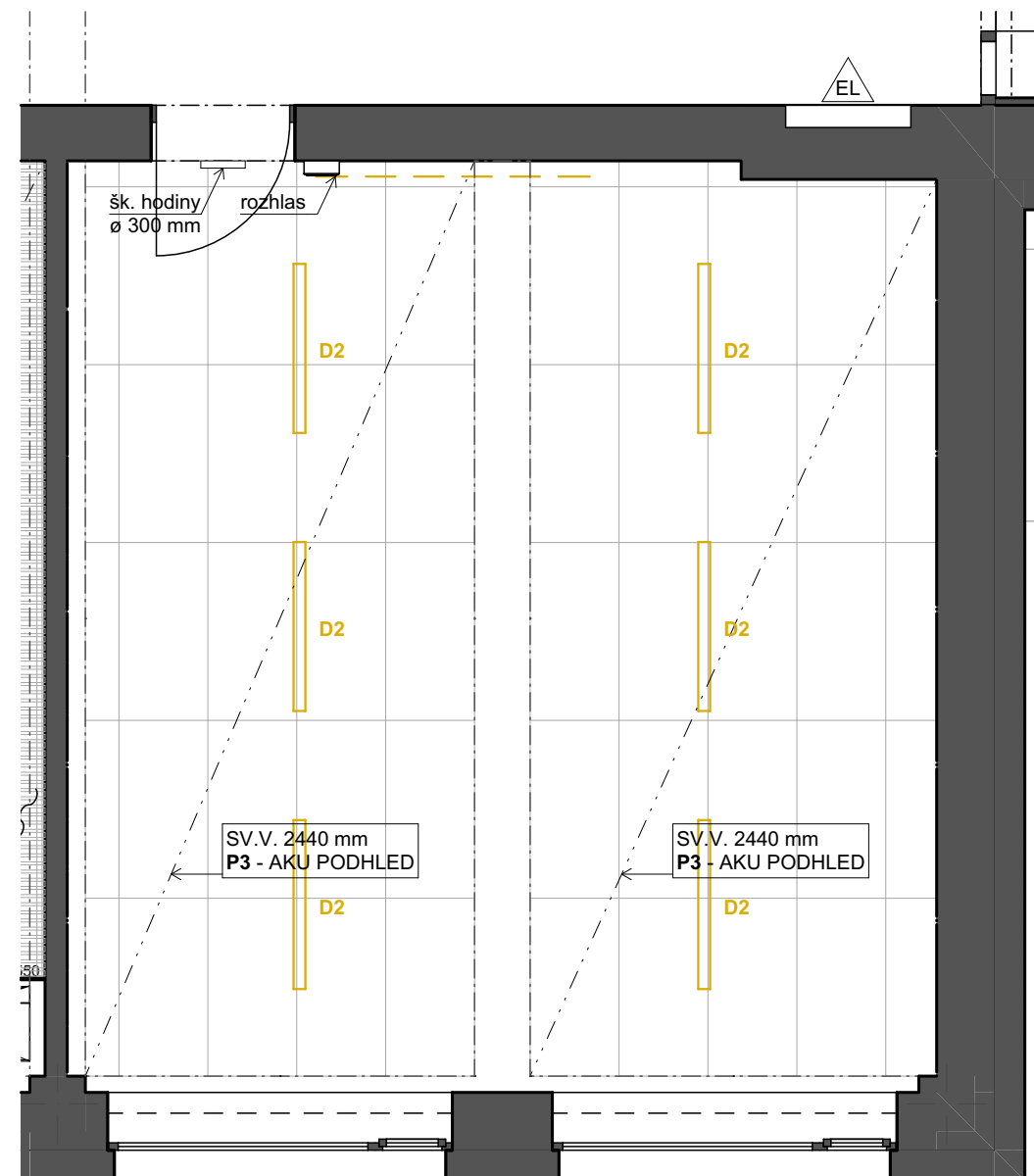
PŮDORYS PODHLEDU
