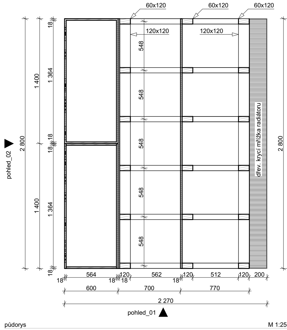
půdorys
