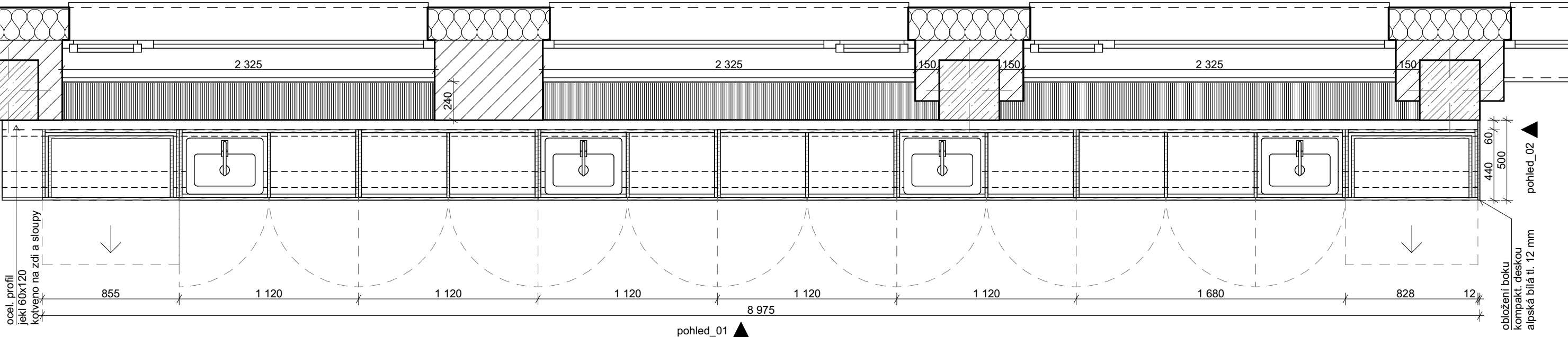
půdorys M 1:25
