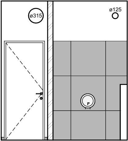
POHLED 1.13_01
