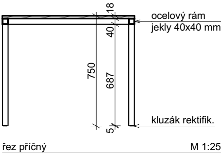
STŮL NAB 02
