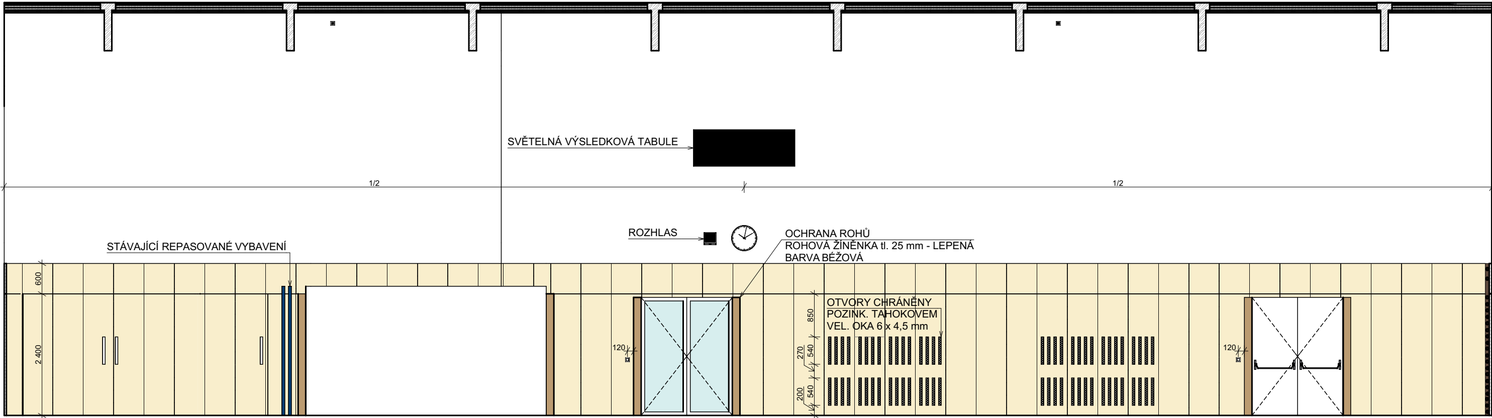
POHLED 1.24_03
