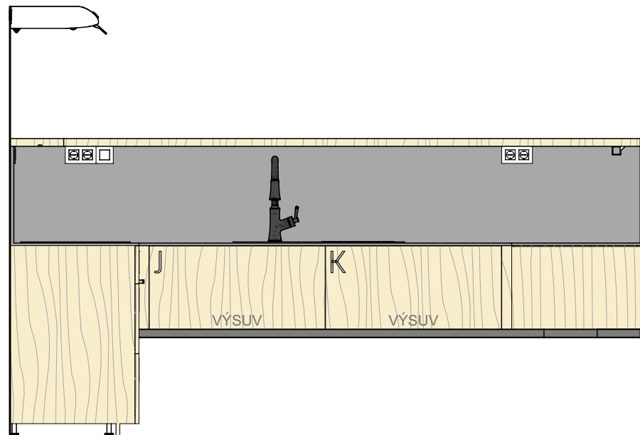
pohled_03_07 M 1:25
