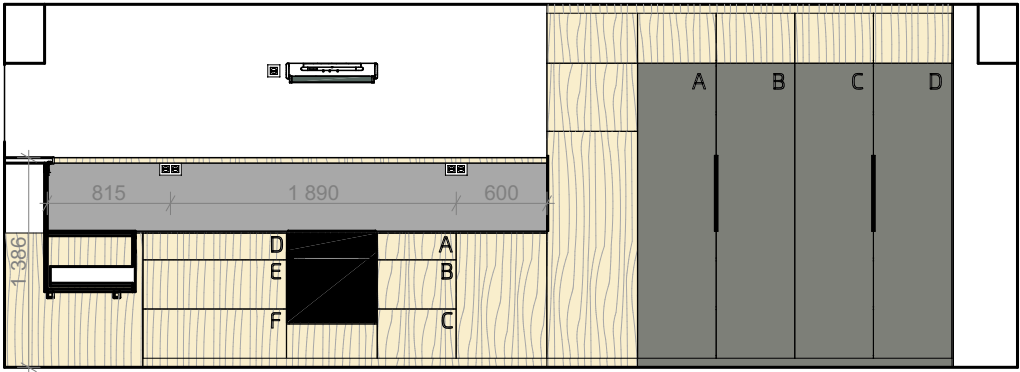
POHLED 01.06_04
