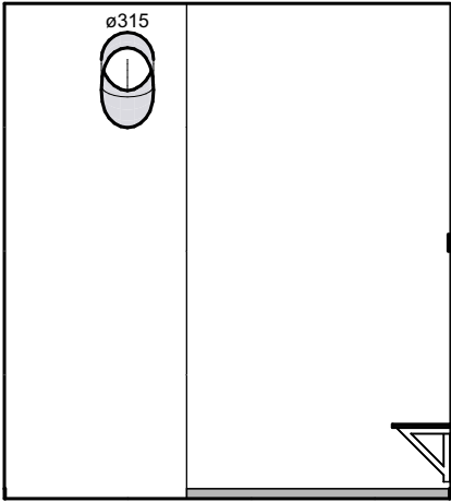
POHLED 1.14_01
