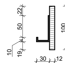
řez příčný M 1:5
