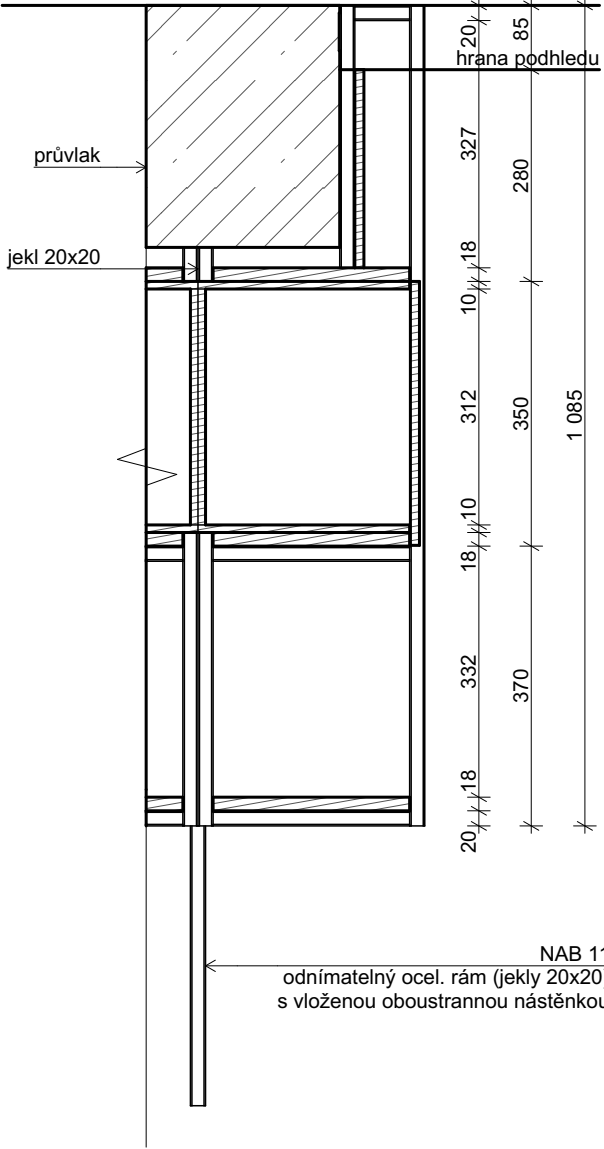
řez příčný M 1:10
