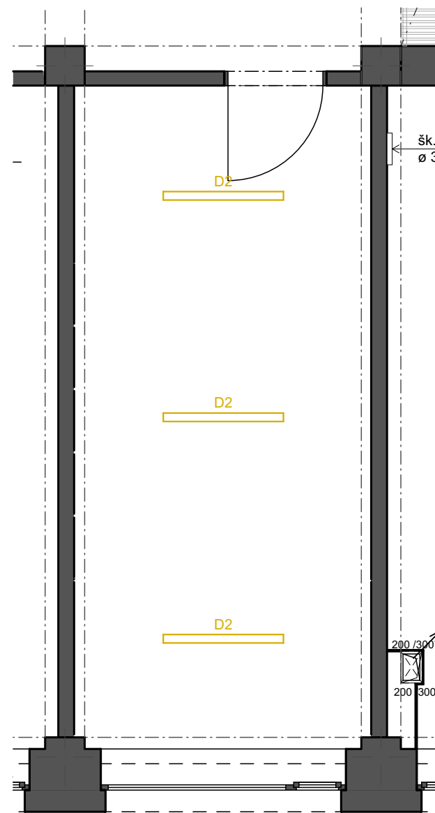
PŮDORYS PODHLEDU
