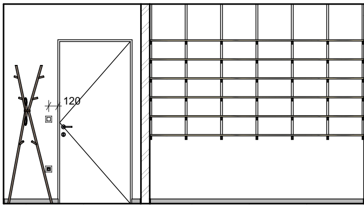
POHLED 2.11_01
