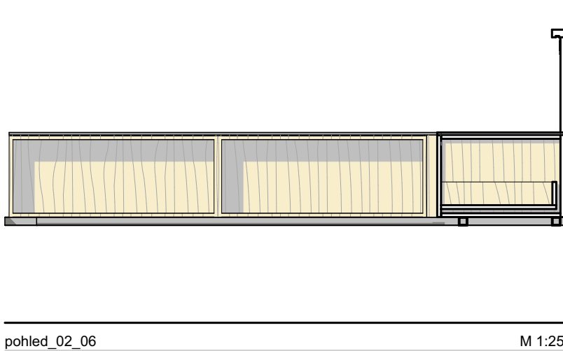
pohled_02_06 M 1:25
