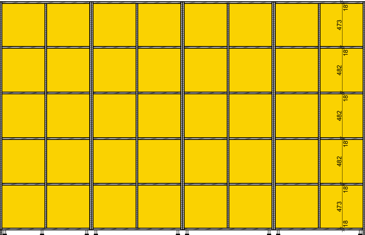
řez podélný
