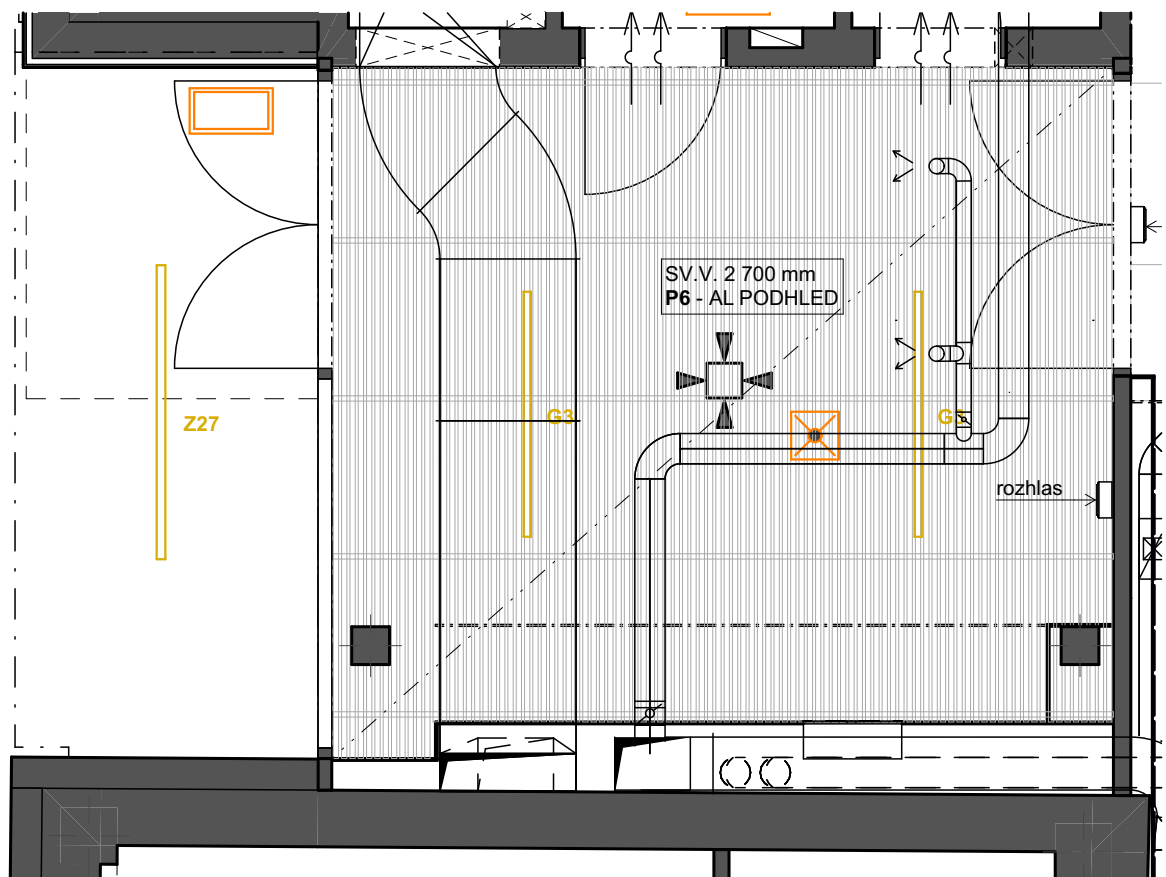
PŮDORYS PODHLEDU
