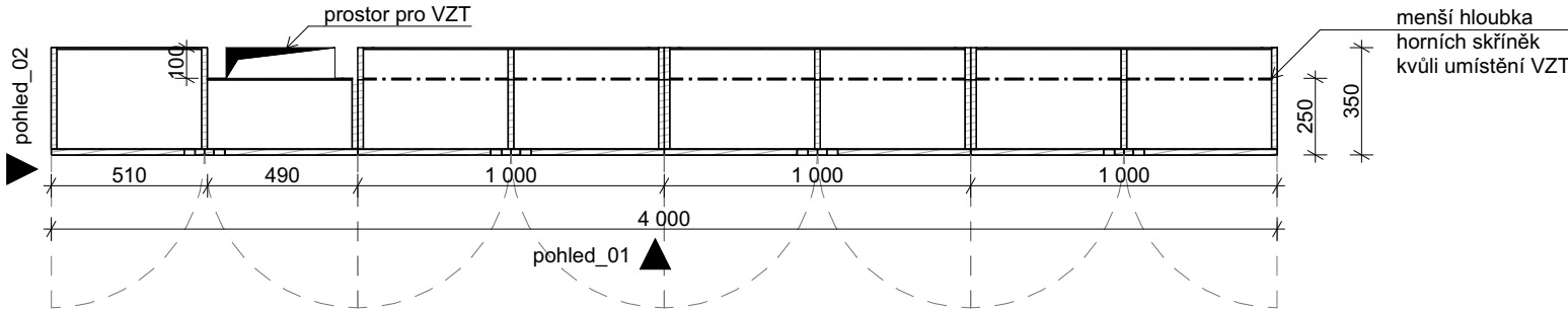
půdorys
