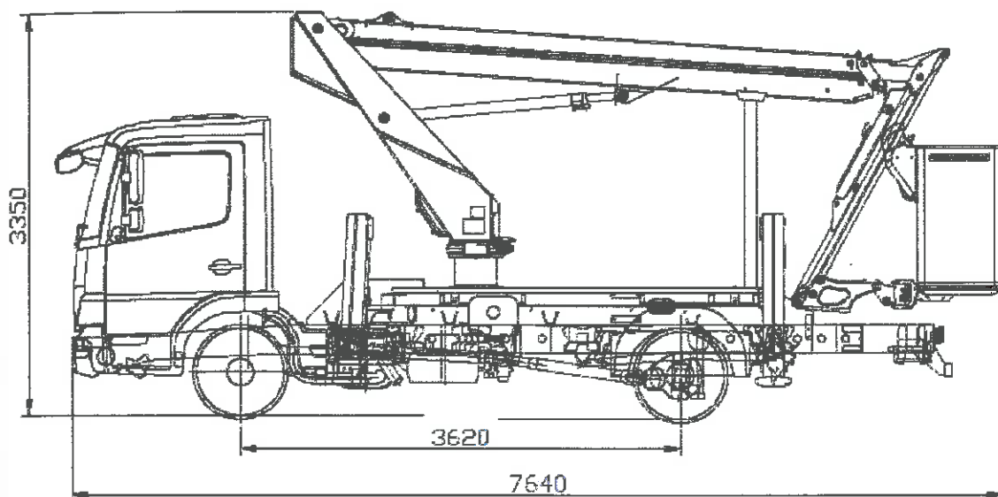
Obr. Rozměrový výkres plošiny PT190J na podvozku Mercedes
