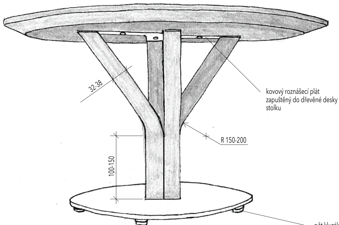
POHLED HORNÍ na dřevěnou nohu
