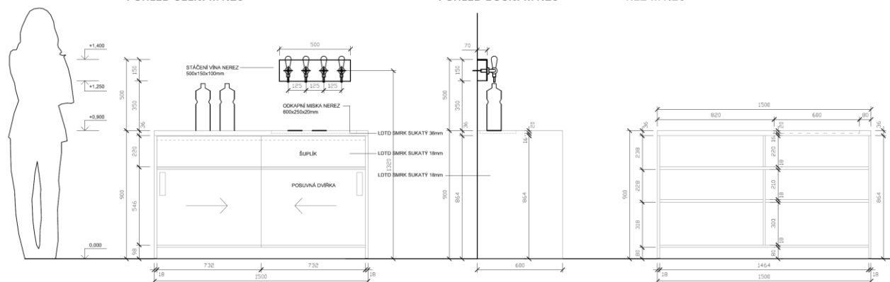
POHLED ČELNÍ M1:20
