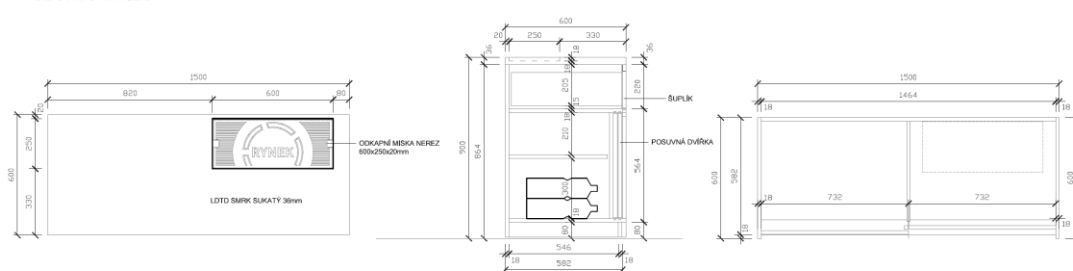
PŮDORYS M1:20
