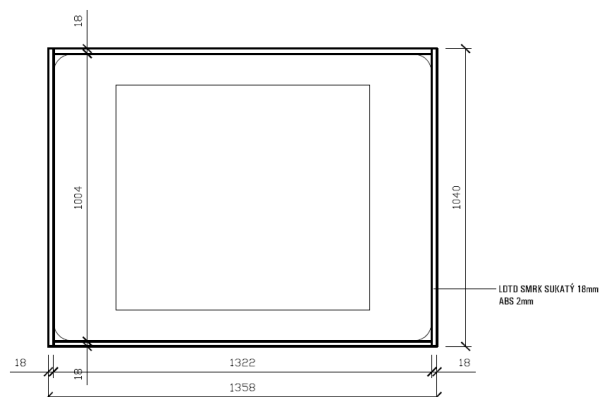
Obr. č.5 – Řešení opláštění van – nutno řešit dle skutečného rozměru van. PŮDORYS M1:20
