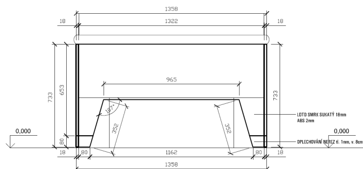
POHLED BOČNÍ M1:20
