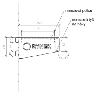
POHLED BOČNÍ
