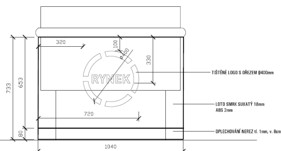
POHLED ČELNÍ M1:20
