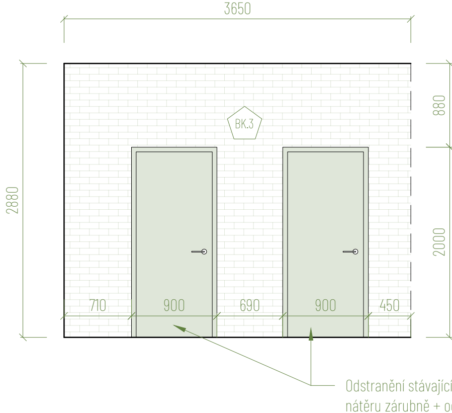
Pohled I
