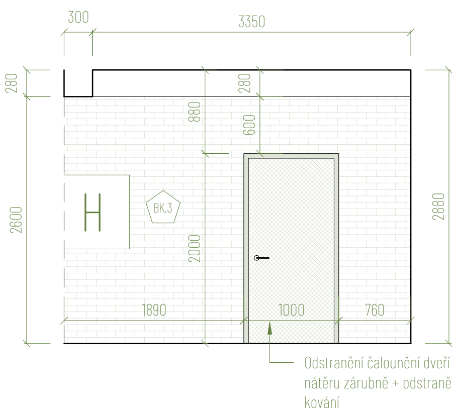
Pohled I
