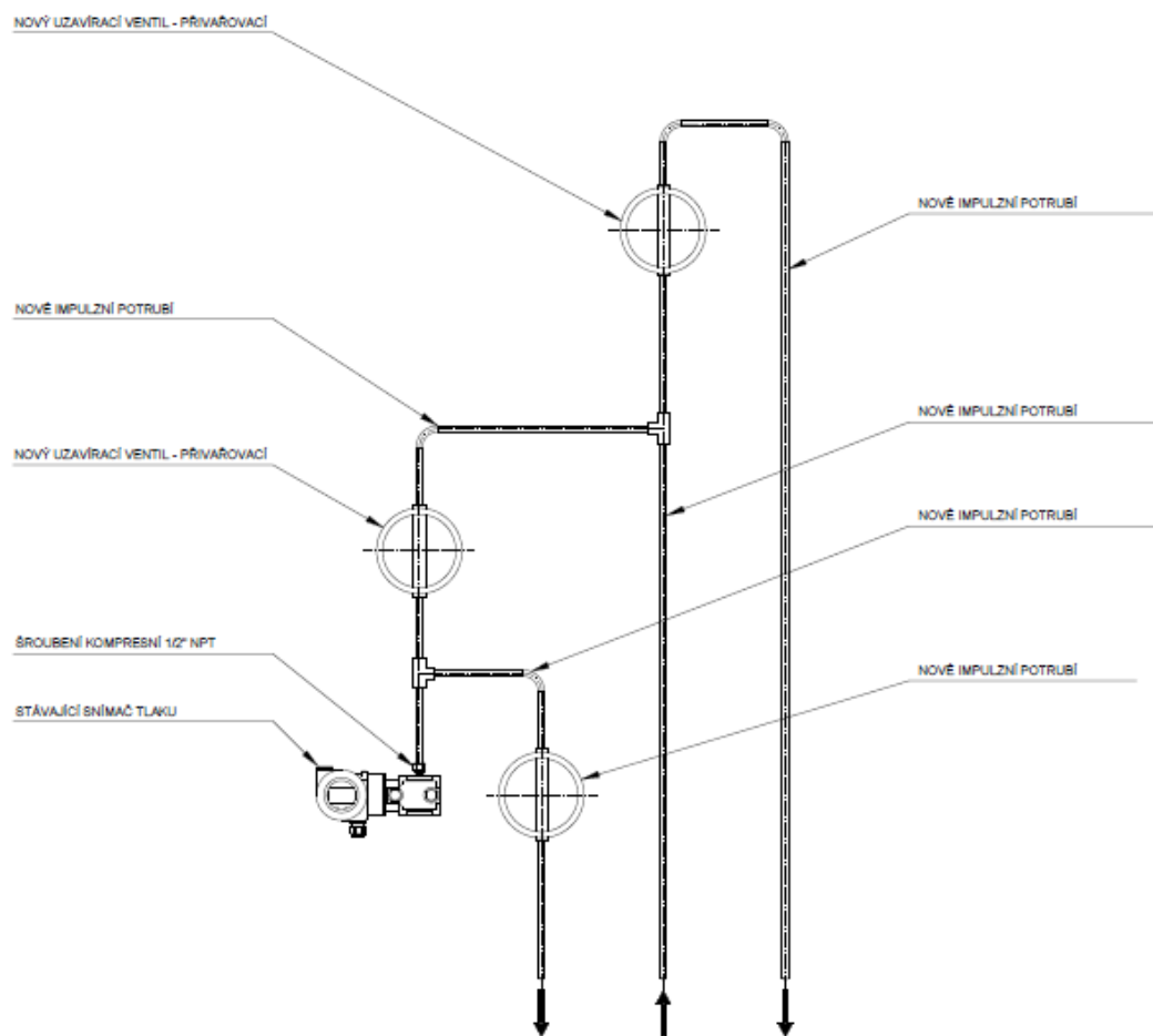
SOUVISEJÍCÍ VÝKRES: Příloha_7_TECHNOLOGIE_MĚŘENÍ TLAKU PÁRY-ROZVODY IMPULSNÍHO POTRUBÍ
