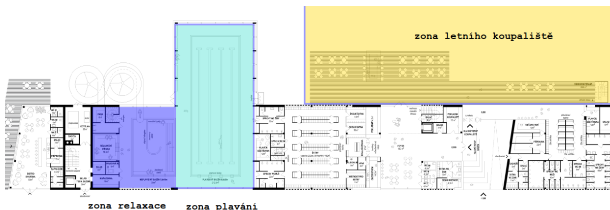
Obrázek 69 – Půdorys 1.NP – placené zóny
