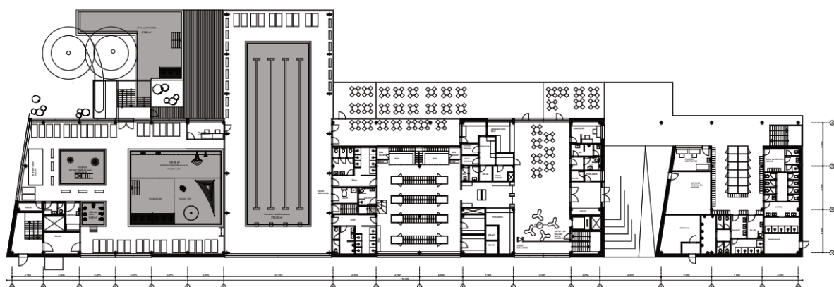
Obrázek 72 – Půdorys 1.NP po úpravách
