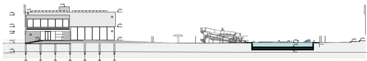
Obrázek 66 – Řez příčný
