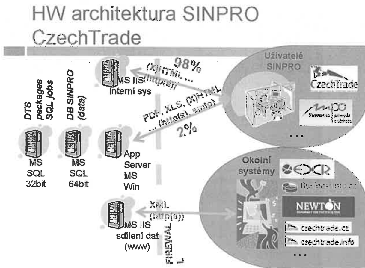
Obrázek 1-1: Základní HW architektura IS SINPRO
