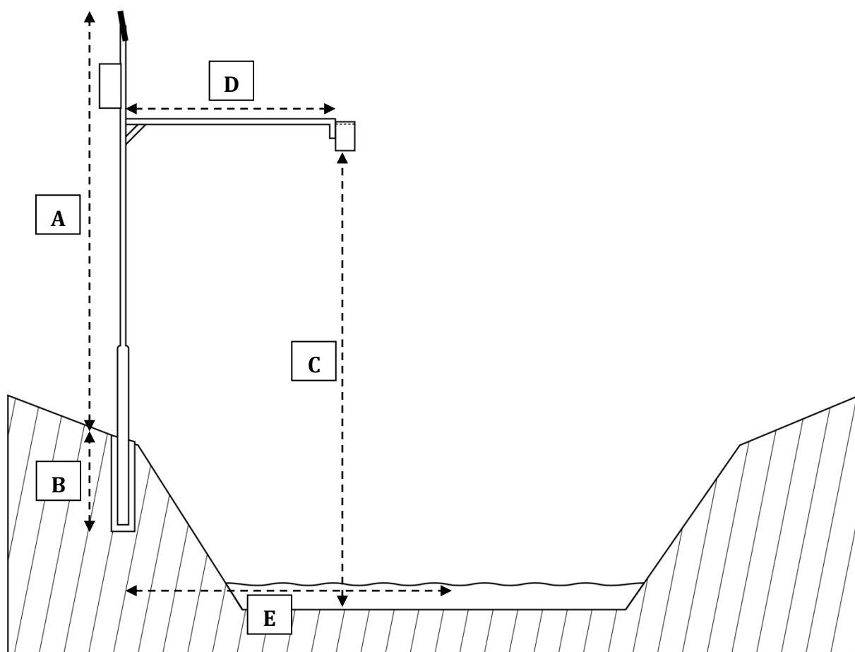
Technické schéma instalace vodoměrné stanice
