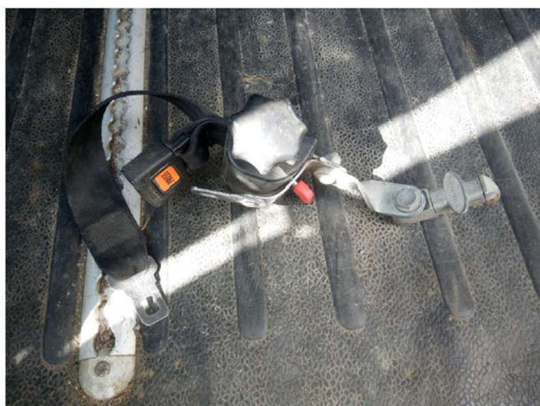
Možné řešení kotvících prvků pro uchycení invalidního vozíku v ližinách v mikrobusu.
