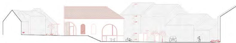
m1200 POHLED JIŽNÍ
