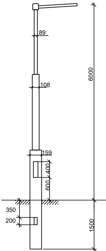
Stožár A1-A4, C3-C6 typ JBUD 6ST (159/108/89) Výložník UD1/89 - 1500
