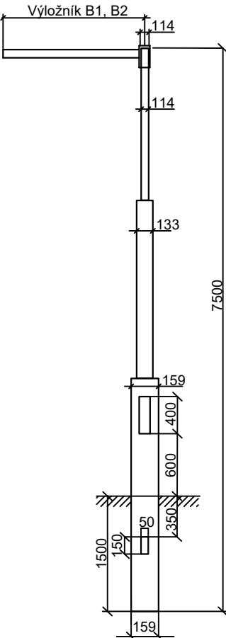
Stožár B1,B2 typ STP 6 - D
