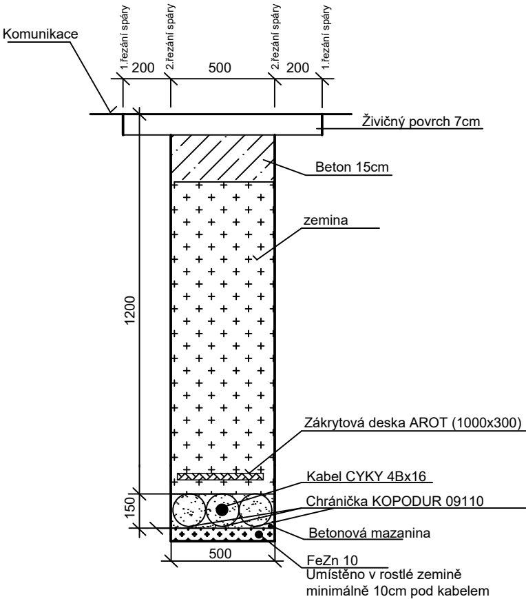
Uložení kabelu pod komunikací
