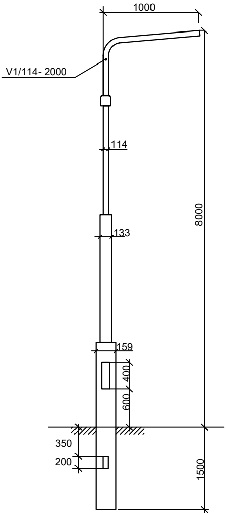
Stožár C1, C2 typ JB8T (159/133/114) Výložník V1/114 - 1000
