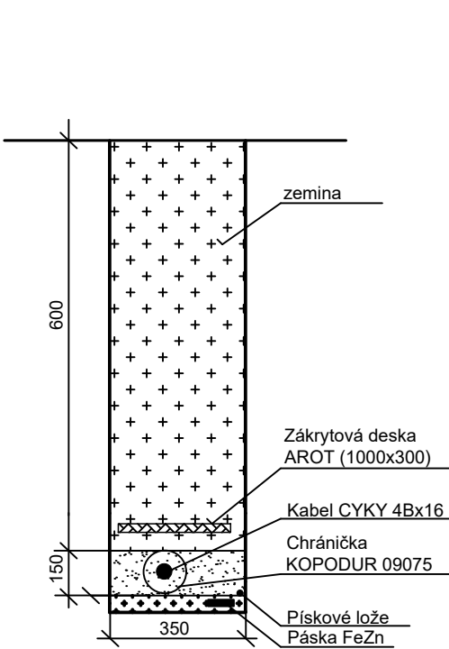
Uložení kabelu v chodníku a pod volným terénem
