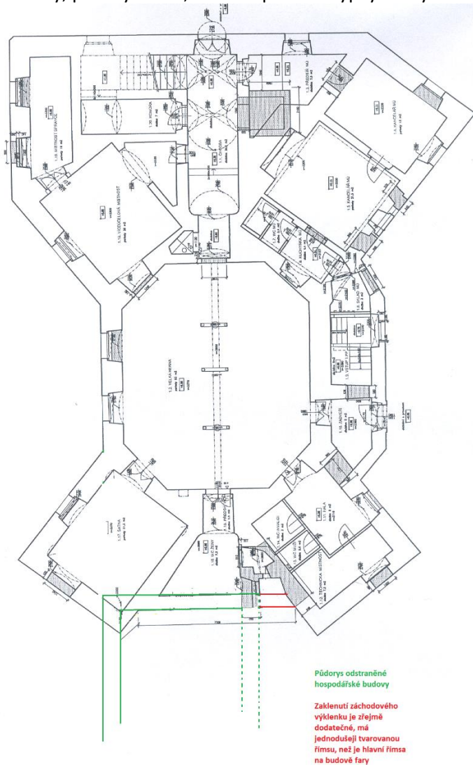
1.g. Tuklaty, půdorys 1.NP, schéma průniku sýpky a fary
