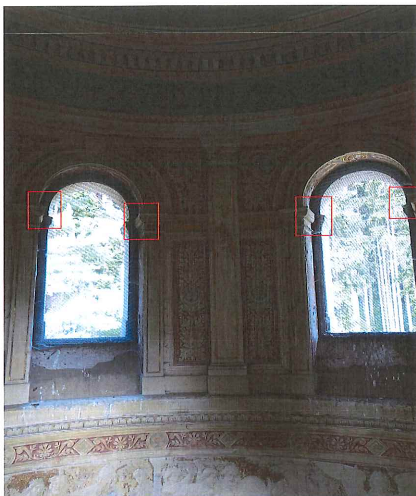
Detail dřevěných rámu a znázorněný problém při demontáži rámu
