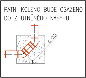
DETAIL PŘECHODU ODPADNÍHO POTRUBÍ NA SVODNÉ
