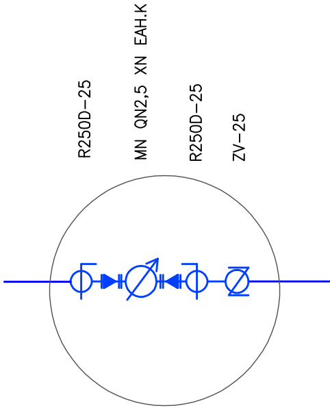
Detail vybavení vodoměrné šachty
