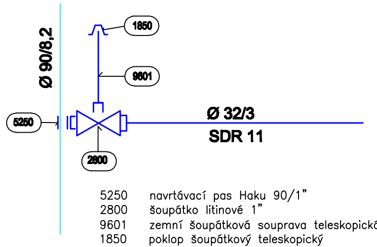
Detail napojení přípojky
