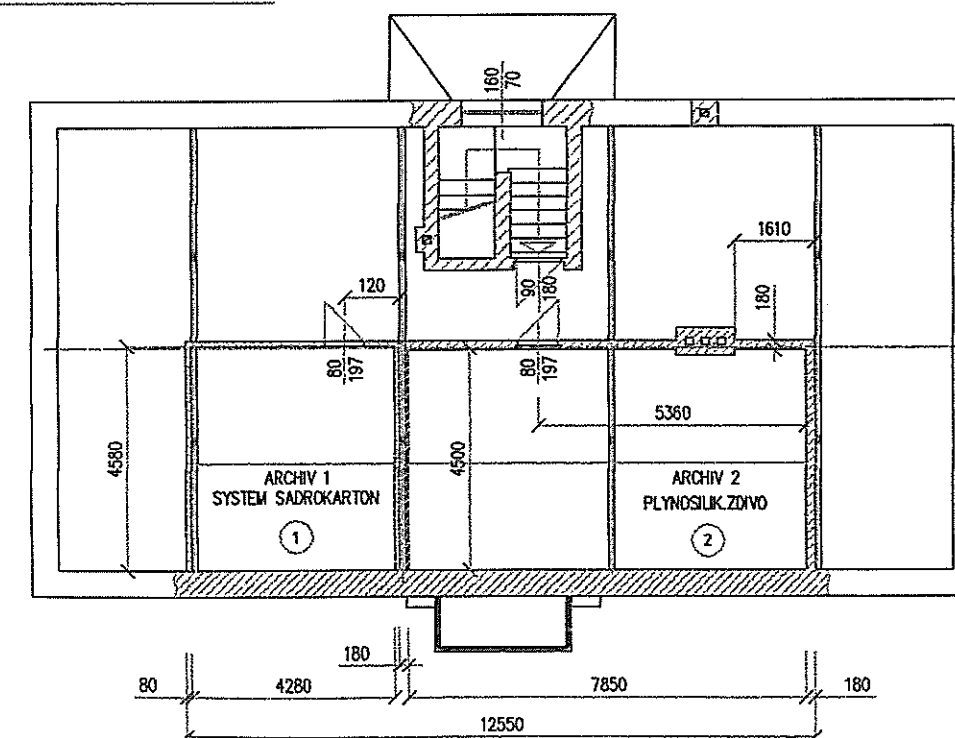
PŮDORYS PŮDNÍ VESTAVBY
