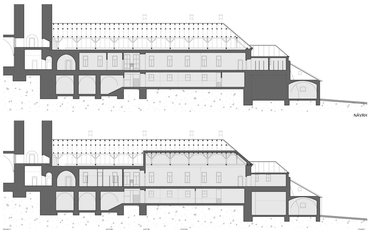
Architektonická studie centra obnovy - klášter Louka, podélný řez (autor Ing. arch. Vratislav Zíka).
