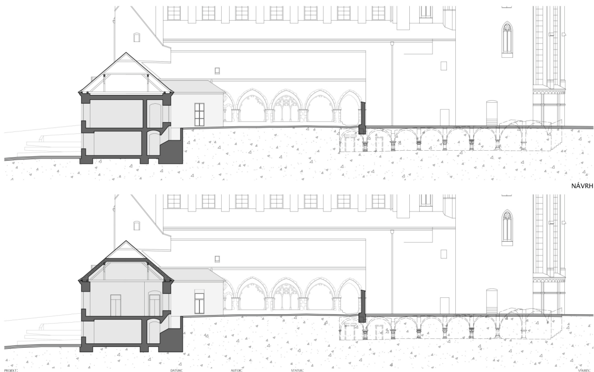
Architektonická studie centra obnovy - klášter Louka, příčný řez (autor Ing. arch. Vratislav Zíka).
