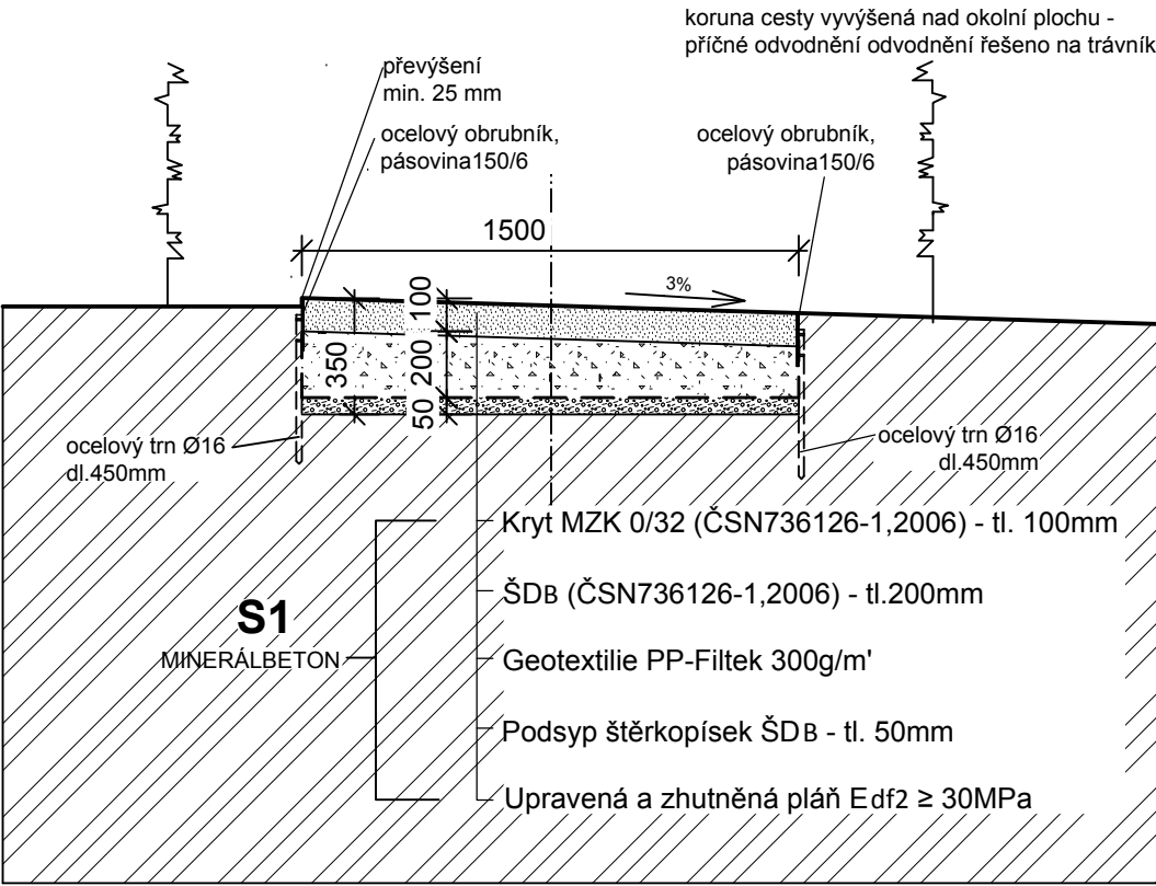
ŘEZ 3-3'
