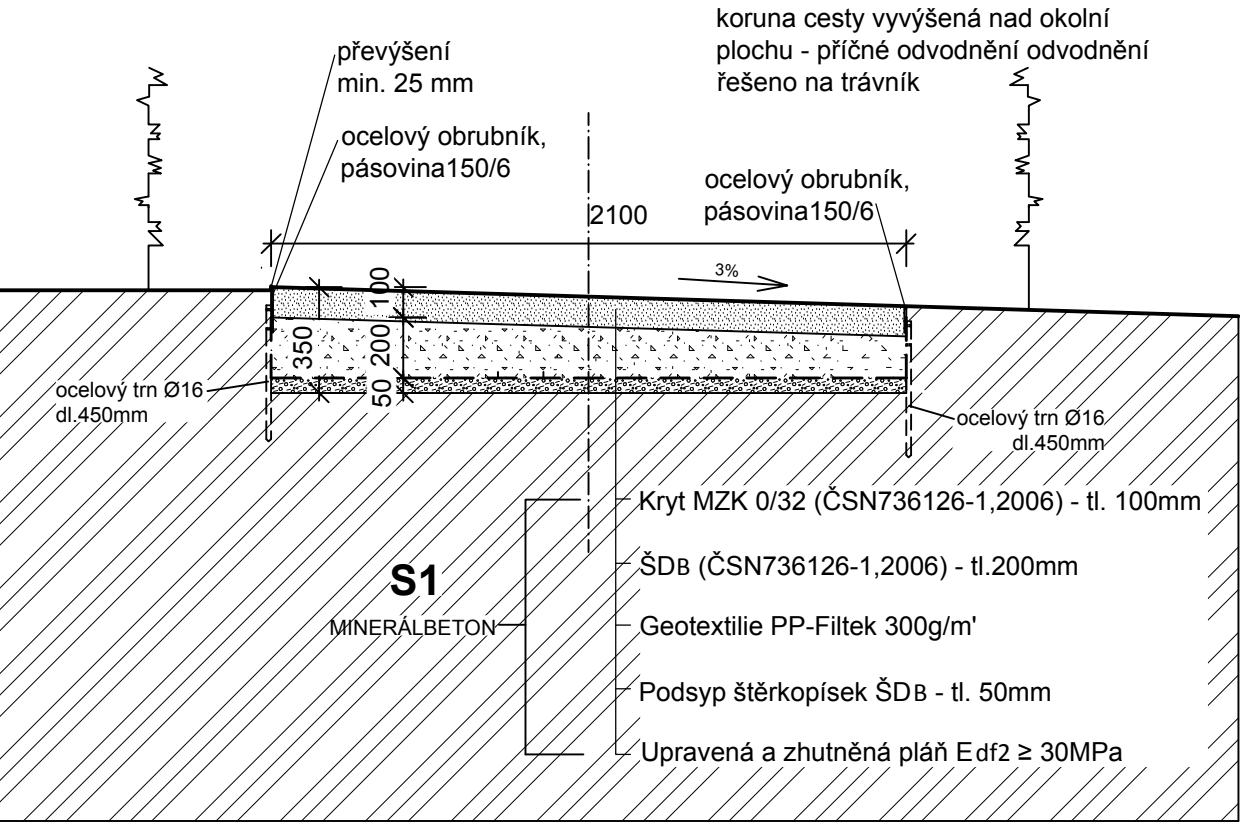
ŘEZ 2-2'
