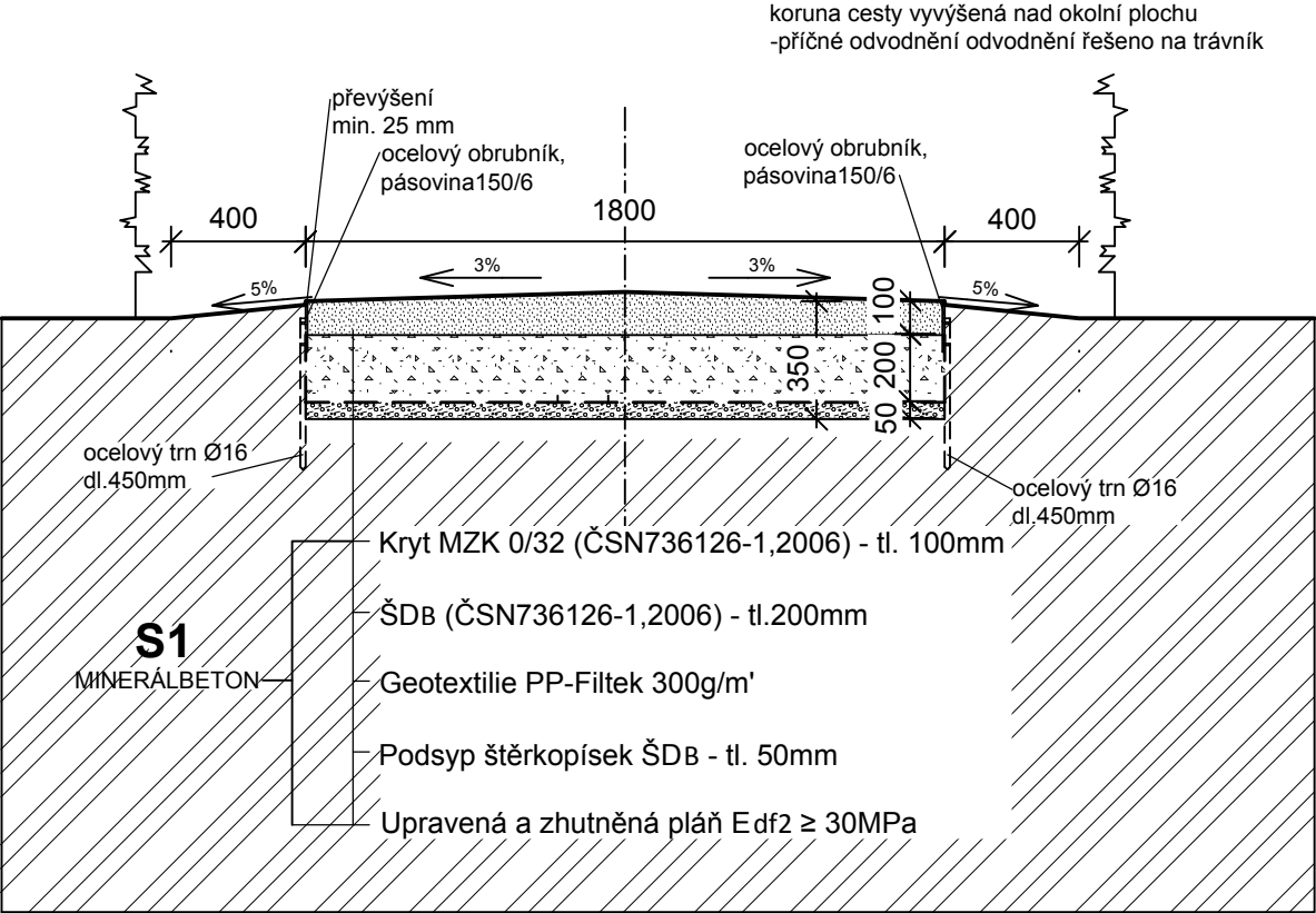
ŘEZ 1-1'
