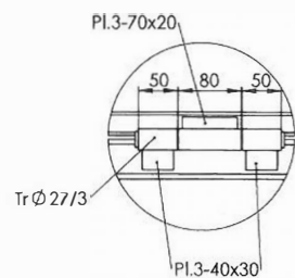
DETAIL C MĚŘITKO 1 : 5
