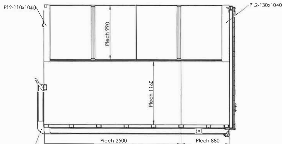
ŘEZ D-D
