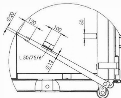
DETAIL B MĚŘITKO 1 : 10
