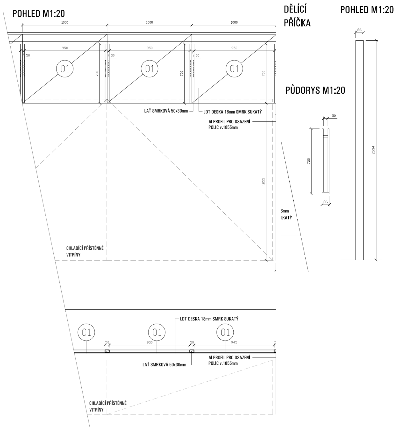
Obr.č. 3 – Schematické řešení dřevěného obložení Provedení za přístěnnými vitrínami
