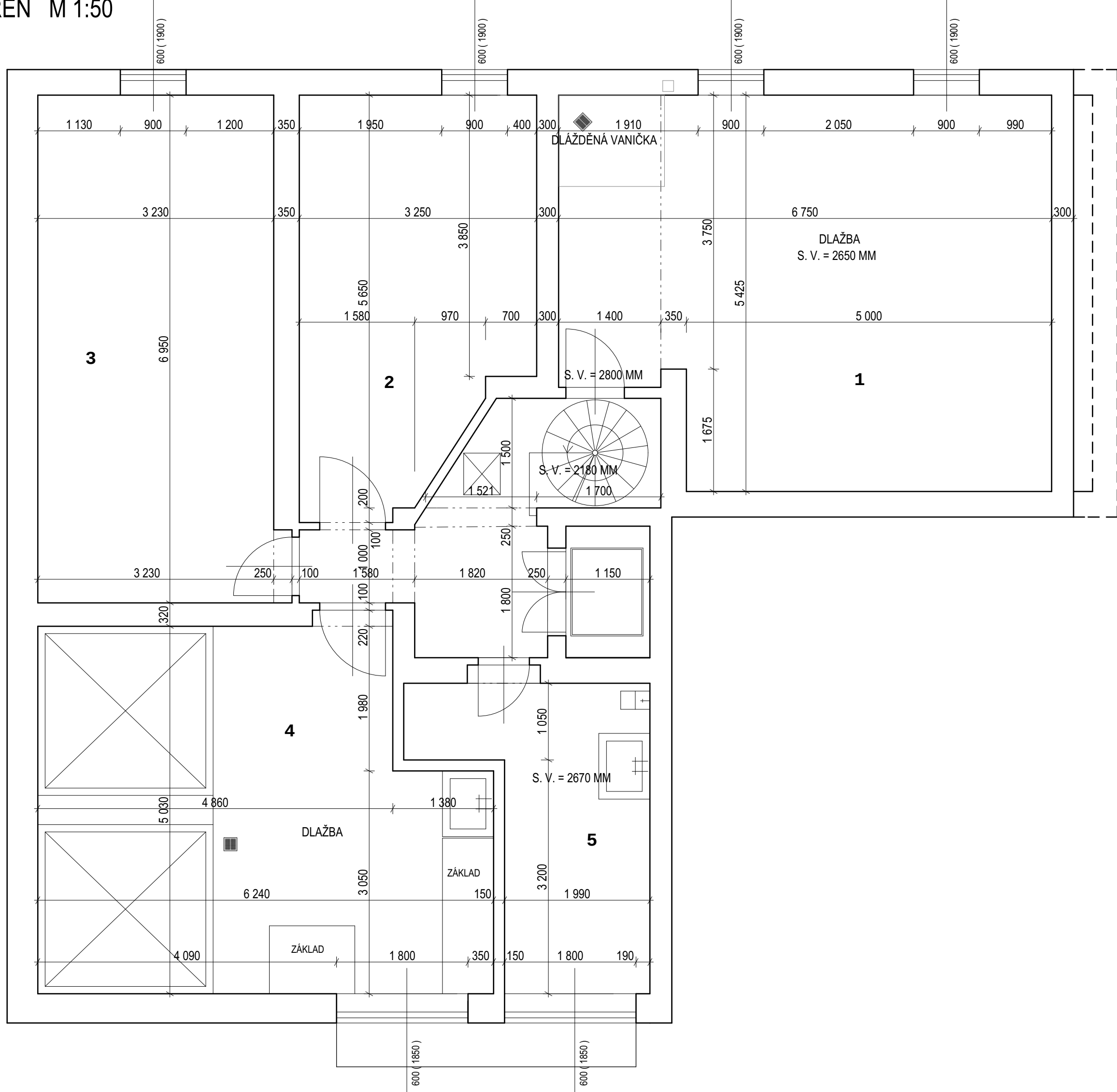
PŮDORYS SUTERÉN M 1:50
