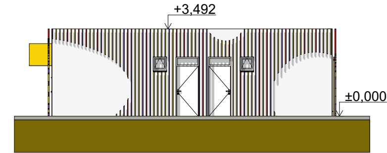
Severní pohled
