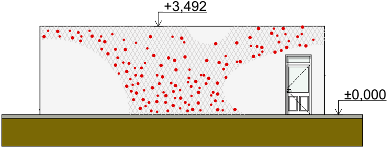
Jižní pohled
