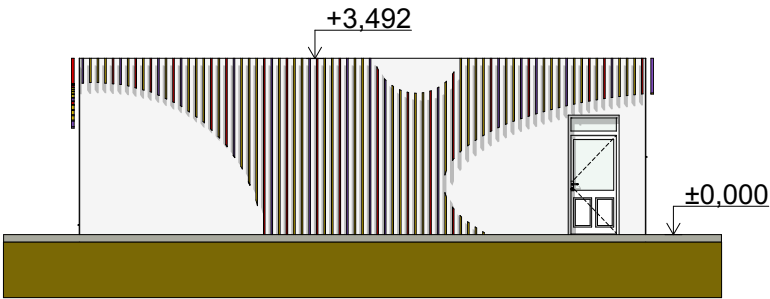
Jižní pohled
