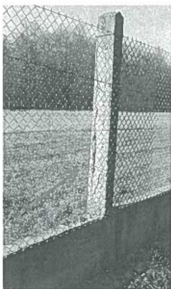
Obr. 2: Poruchy betonového sloupku, obnažená výztuž
