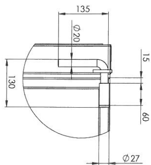
DETAIL A MÉRITKO 1 : 5
